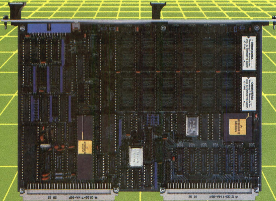
OB68K/VME1™
