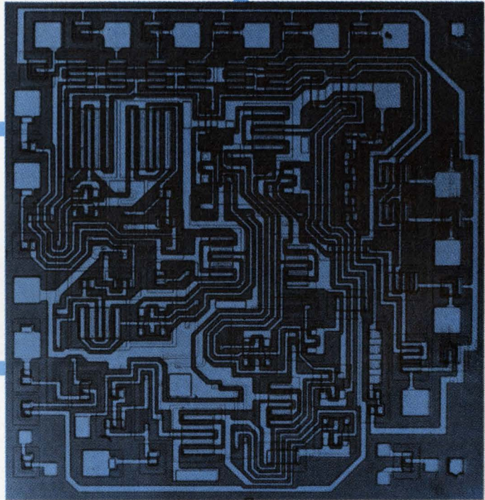
MC7441A
