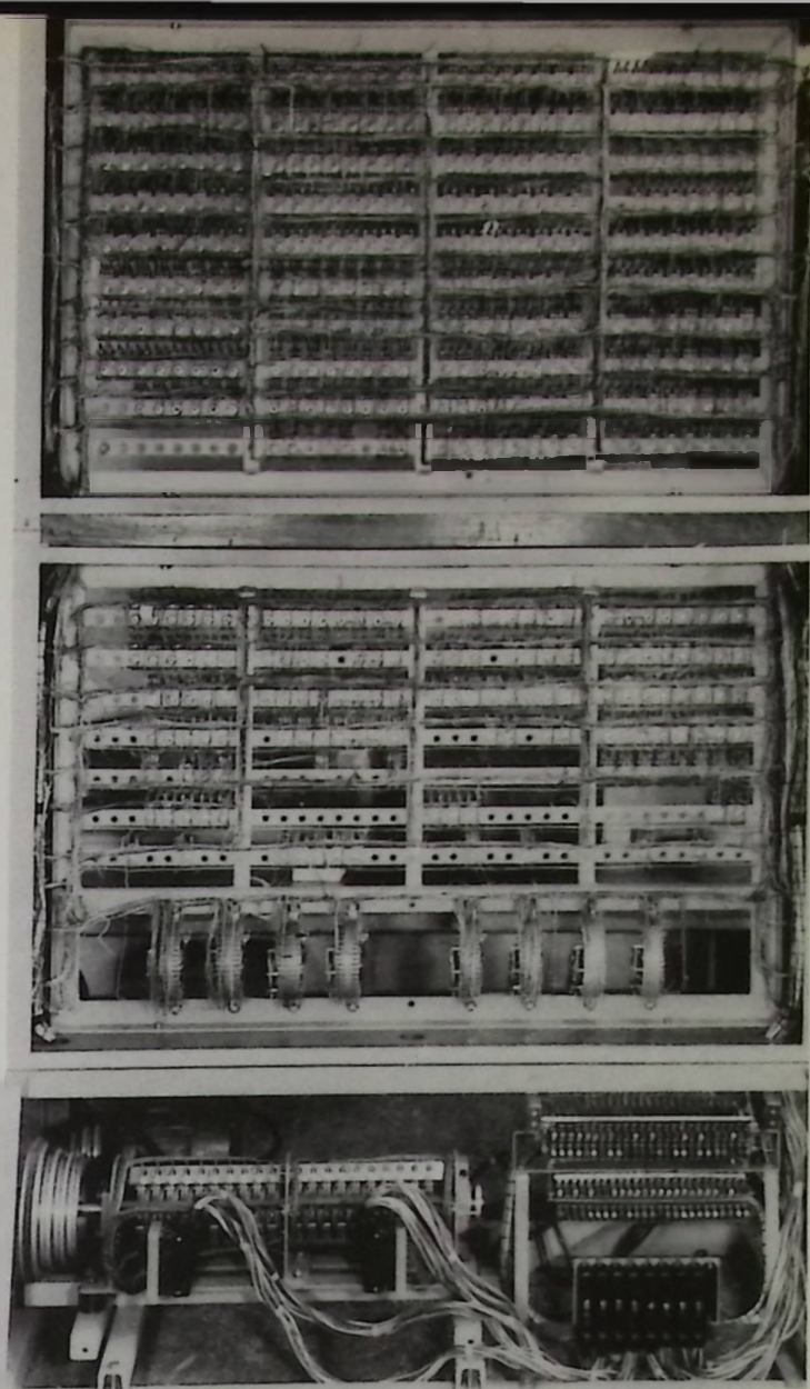
Rechenwerk der ZUSE Z 3, unten die Schaltwalze (Taktgeber)
