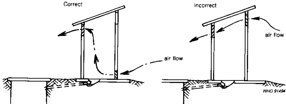
Fig. 7.34. Ventilation In a pour-flush latrine
