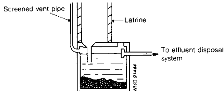
Fig. 6.25. Aqua-privy
