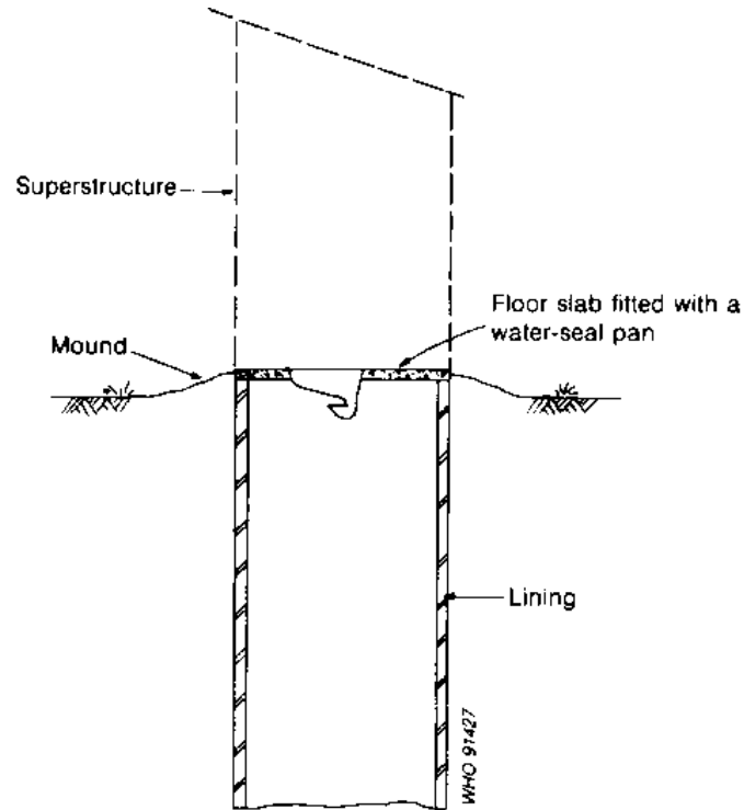
Fig. 6.8. Pour-flush latrine
