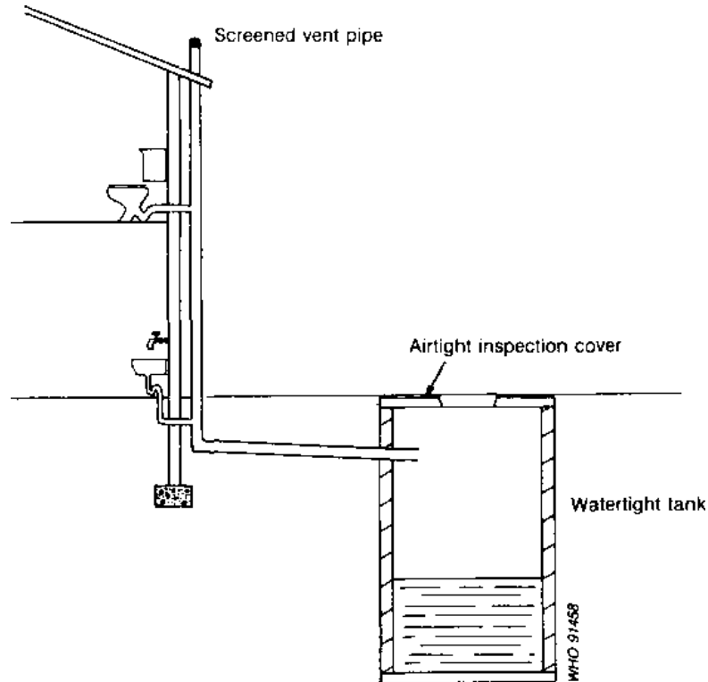
Fig. 6.39. Cesspit
