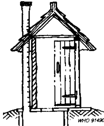
Fig. 7.30. Straight vent pipe
