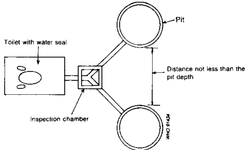
Fig. 6.15. Double-pit offset pour-flush latrine
