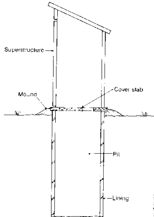
Fig. 6.3. Simple pit latrine
