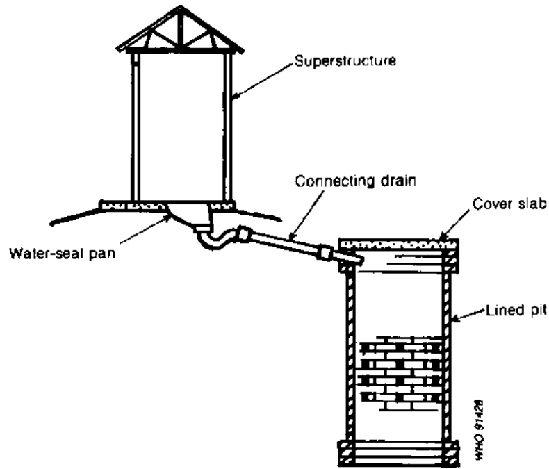
Fig. 6.9. Offset pour-flush latrine
