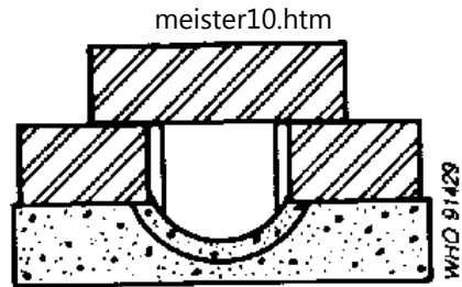
Fig. 6.10. Brick-covered drain
