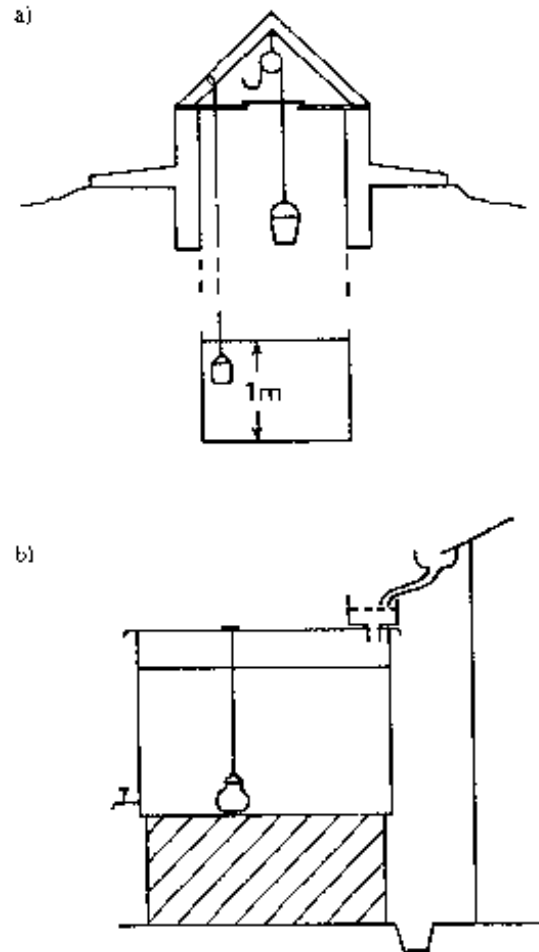
Fig. 31: Diffusion chlorination a) well, b) cistern
