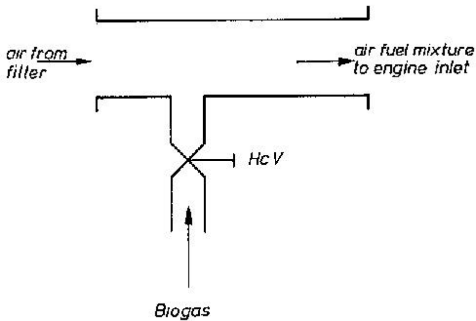
Fig. 5.1: T-joint mixer
