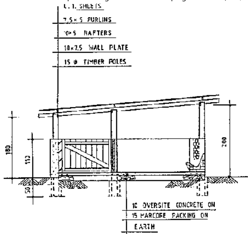
Section A-A
