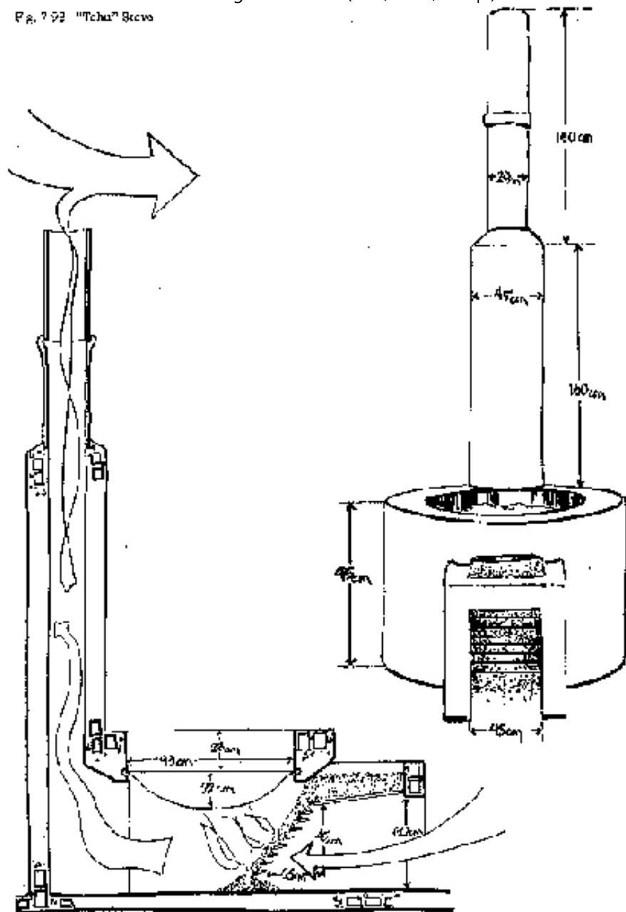
Fig. 7-93: "Tahu" Stove
