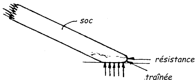
Figure 34 : Un soc émoussé provoque une semelle de labour qui augmente la traction et rend difficile la pénétration dans le sol.
