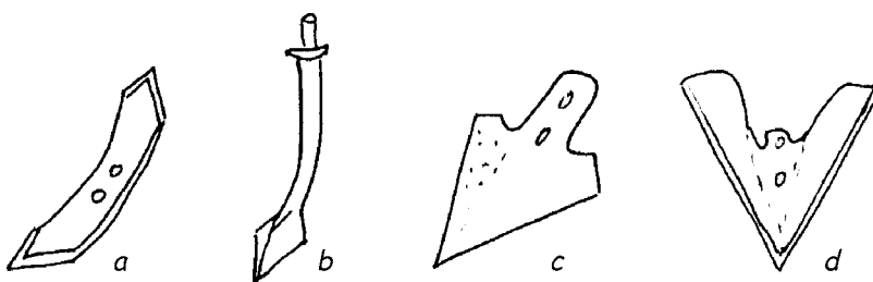
Figure 38 : Quelques exemples de dents de scarificateur: (a) soc réversible permettant de scarifier les sols plus durs. (b) soc rigide. (c) soc patte d'oie utilisé pour scarifier les sols plus légers et pour le désherbage. (d) Le soc sarcleur employé pour le désherbage.
