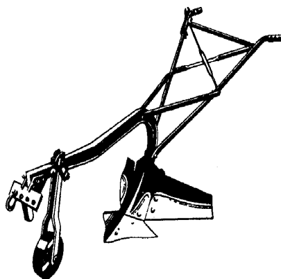
Figure 41 : Billonneur à ailerons «Inkunki», fabriqué au Zimbabwe.
