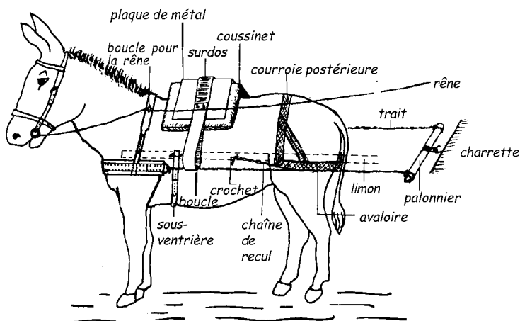
Figure 23 : Disposition de la bricole, de l'avaloire et de la selle permettant de harnacher un âne aux limons d'une charrette à deux roues.
