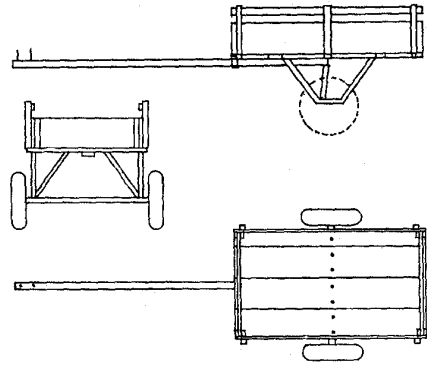
Figure 31 : Type de charrette largement répandu en Afrique de l'Ouest, construite à partir d'un solide essieu fixe en acier, de roulements à billes et de roues et pneus importés.
