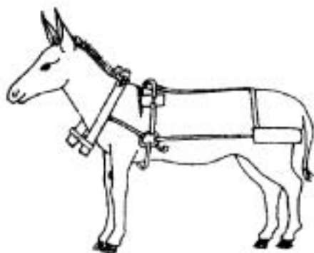
Figure 20 : Harnais à collier sud-africain muni d'attelles droites.
