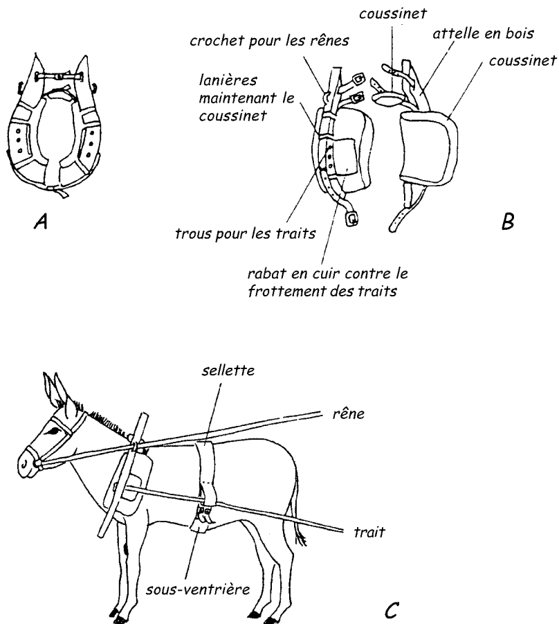
Figure 21 : Harnais à collier à trois coussinets muni d'une sellette et d'une sous-ventrière.
