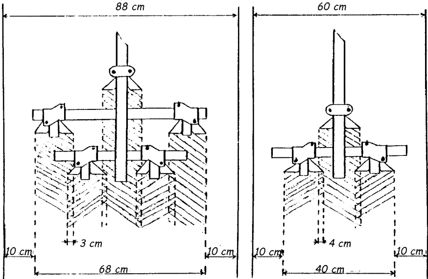
Figure 48 : Disposition pour cinq dents (à gauche) et trois dents (à droite) permettant de travailler en un seul passage dans des rangées de respectivement 90 et 60 cm.
