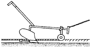
Figure 36 : Réglage vertical (de la profondeur) d'une charrue; les proportions sont exagérées par souci de clarté.
