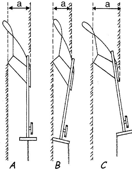
Figure 35 : Réglage horizontal (de la largeur) de la charrue ; on a exagéré les proportions par souci de clarté.
