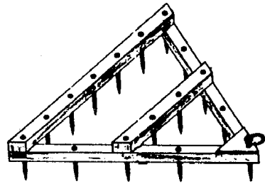
Figure 42 : Dessin d'une simple herse en bois, à pointes.
