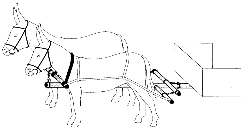
Figure 18 : Bricole rallongée sur deux ânes tirant un char à bœufs. Voir la figure 22 pour les palonniers.
