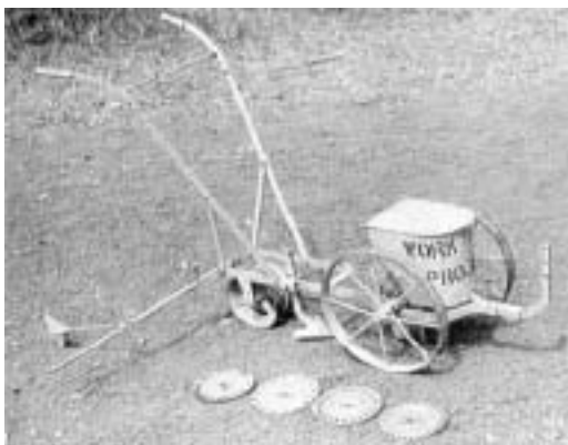
Figure 47 : Semoir Super-Eco et différentes plaques de distribution ainsi que le traceur de sillon.
