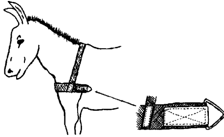
Figure 15 : Bricole à sangles avec lanière de cou.
