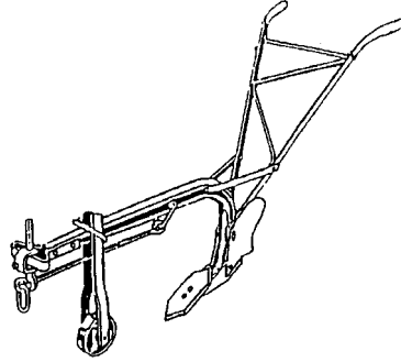
Figure 40 : Rippeur de Magoye fixé sur l'age d'une charrue.
