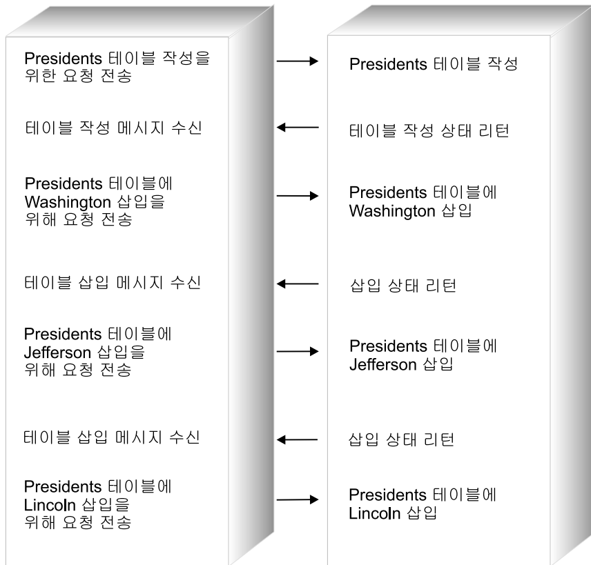
그림 23. 저장 프로시저어(stored procedure)가 없는 입력 SQLDA 샘플
