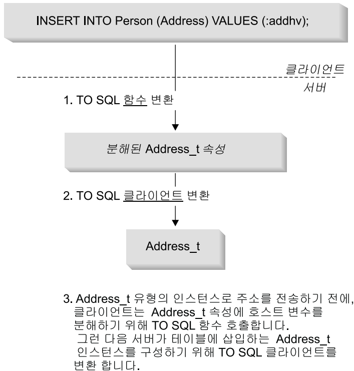
그림 18. 클라이언트에서 구조화 유형으로 바인딩
