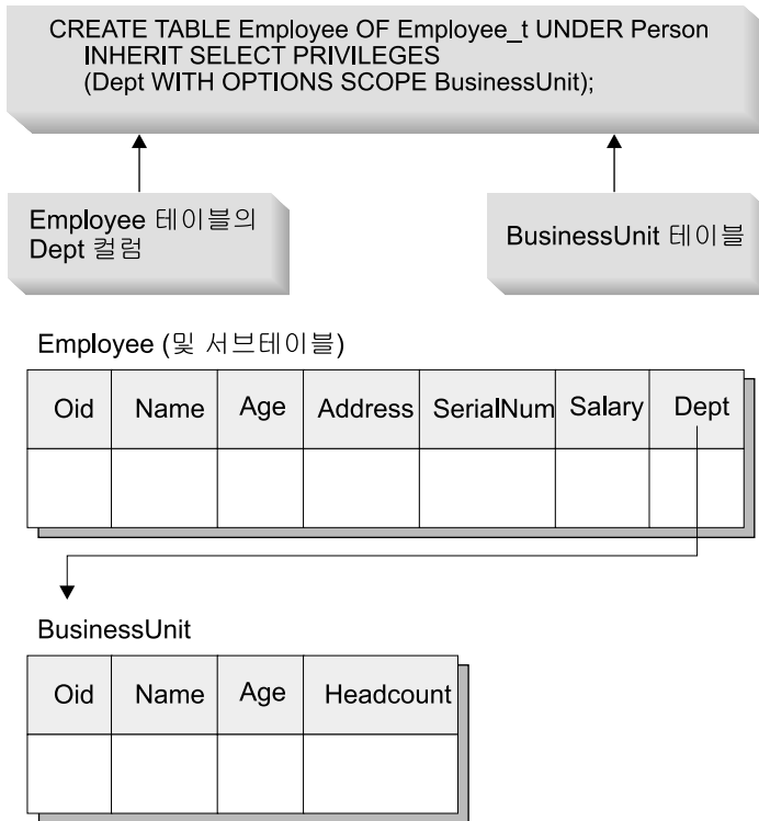
그림 12. BusinessUnit 오브젝트를 참조하는 Dept 속성
