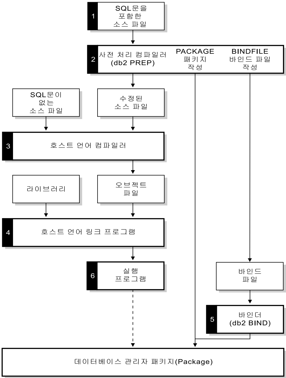
그림 1. 컴파일되는 호스트 언어(host language)로 작성된 프로그램 준비
