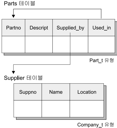
그림 13. 자체 참조 범위의 예
