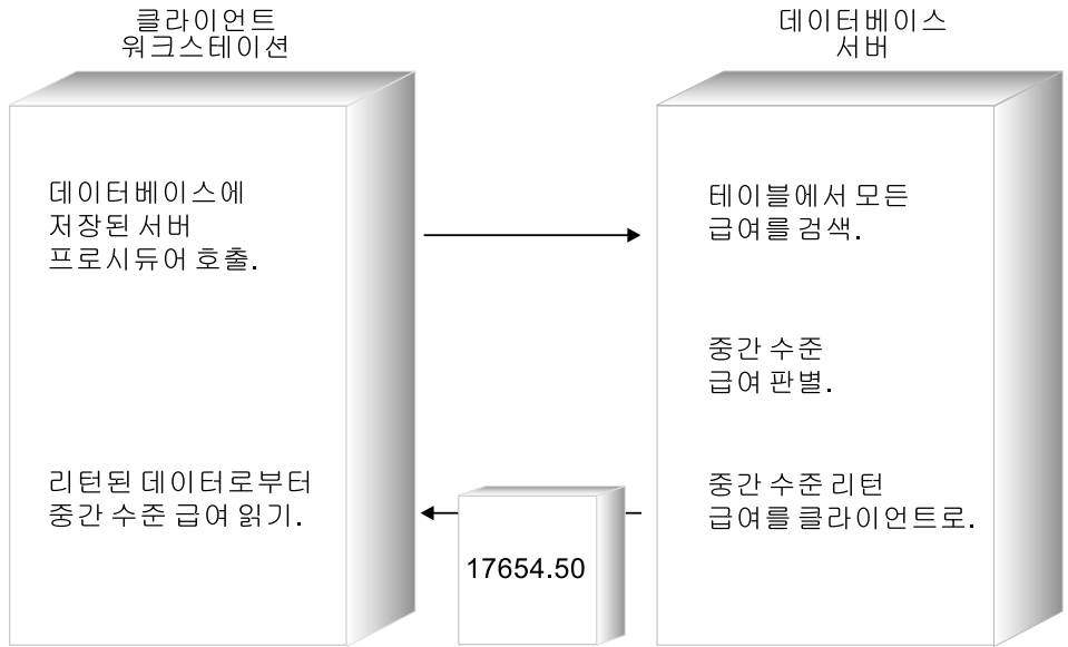
그림 6. 저장 프로시저(stored procedure)를 사용하는 OUT 매개변수 샘플
