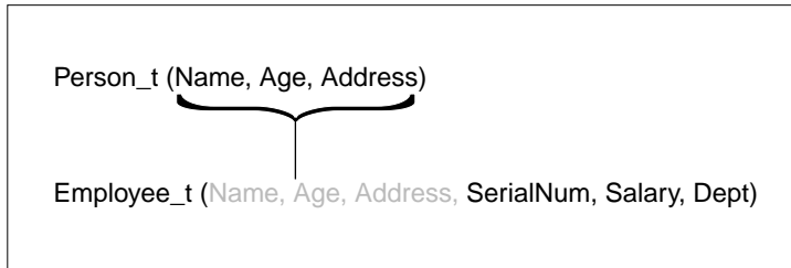
그림 7. 구조화 유형 Employee_t 는 Person_t 에서 상속됩니다.
