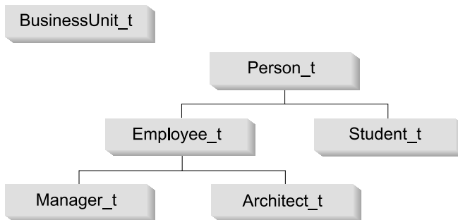
그림 8. 유형 계층(BusinessUnit_t 및 Person_t)
