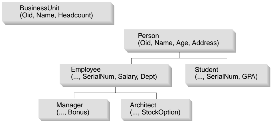
그림 11. 유형지정 테이블 계층
