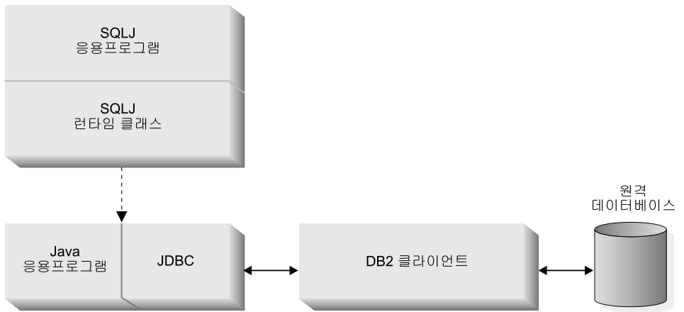
그림 21. DB2 Java 응용프로그램 구현
