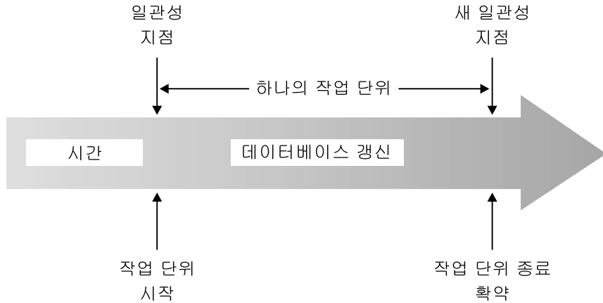
그림 2. 제약 명령문이 있는 작업 단위(UOW)
