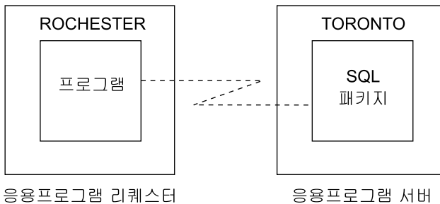
그림 6. 분산 관계형 데이터베이스 환경
