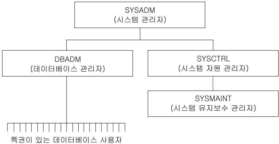
그림 1. 권한 및 특권의 계층
