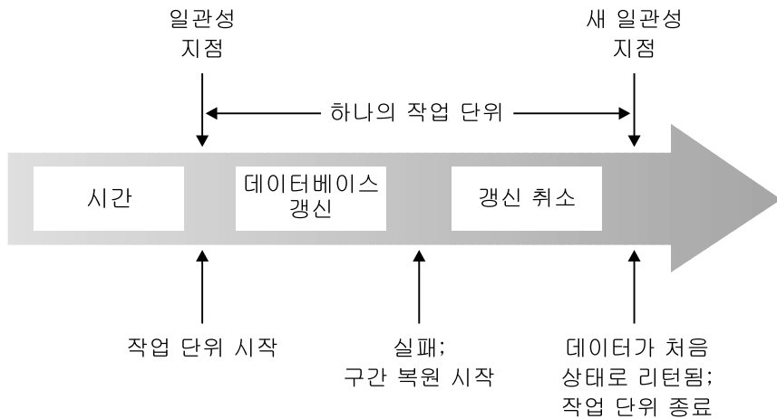
그림 3. 구간 복원 문이 있는 작업 단위(UOW)
