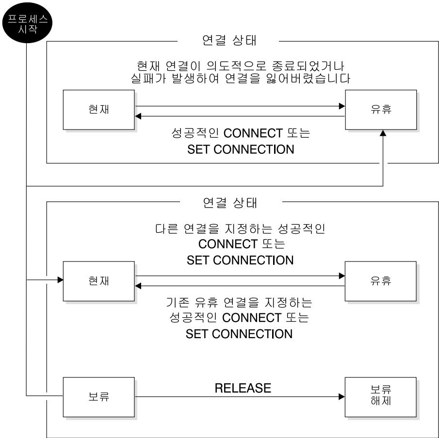
그림 9. 응용프로그램 직접 분산 작업 단위 연결 및 프로세스 연결 상태 전이
