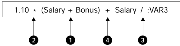
그림 11. 연산 순서
