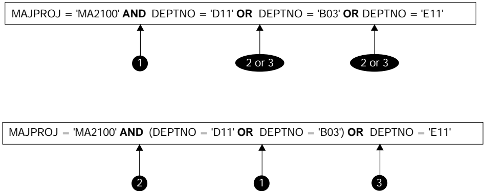
그림 13. 검색 조건 평가 순서
