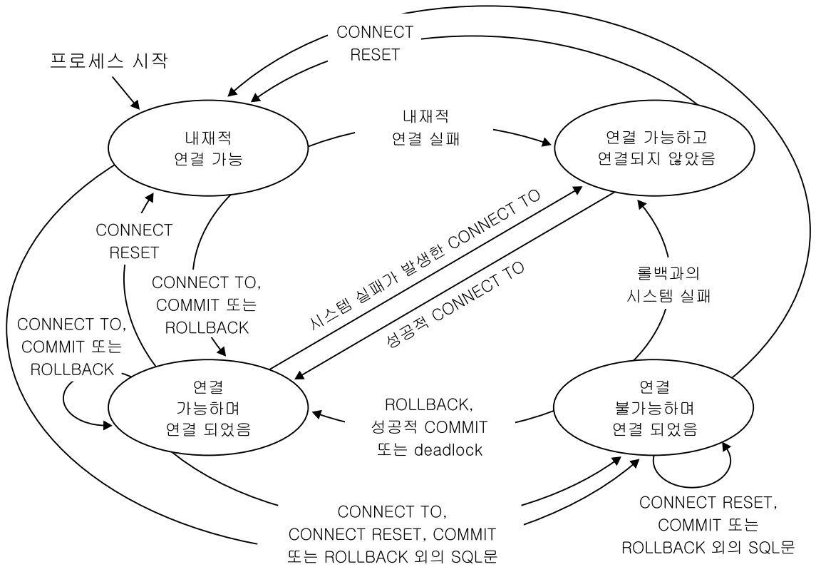
그림 7. 내재 연결을 사용할 수 있는 경우 연결 상태 전이
