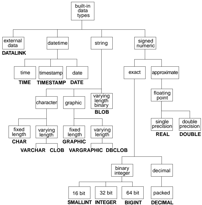
그림 10. 지원되는 내장형 데이터 유형
