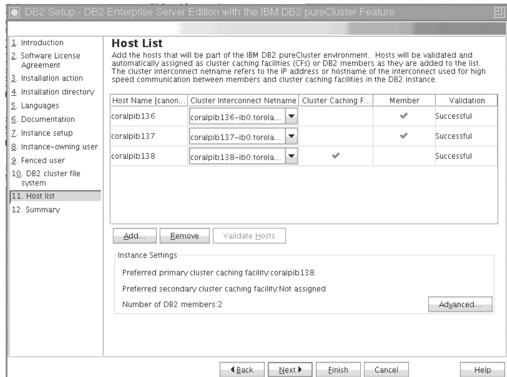
Obrázek 39. Panel Seznam hostitelů se třemi hostiteli (jeden je předem načtený hostitel zahajující instalaci a ostatní dva hostitelé byli přidáni)
