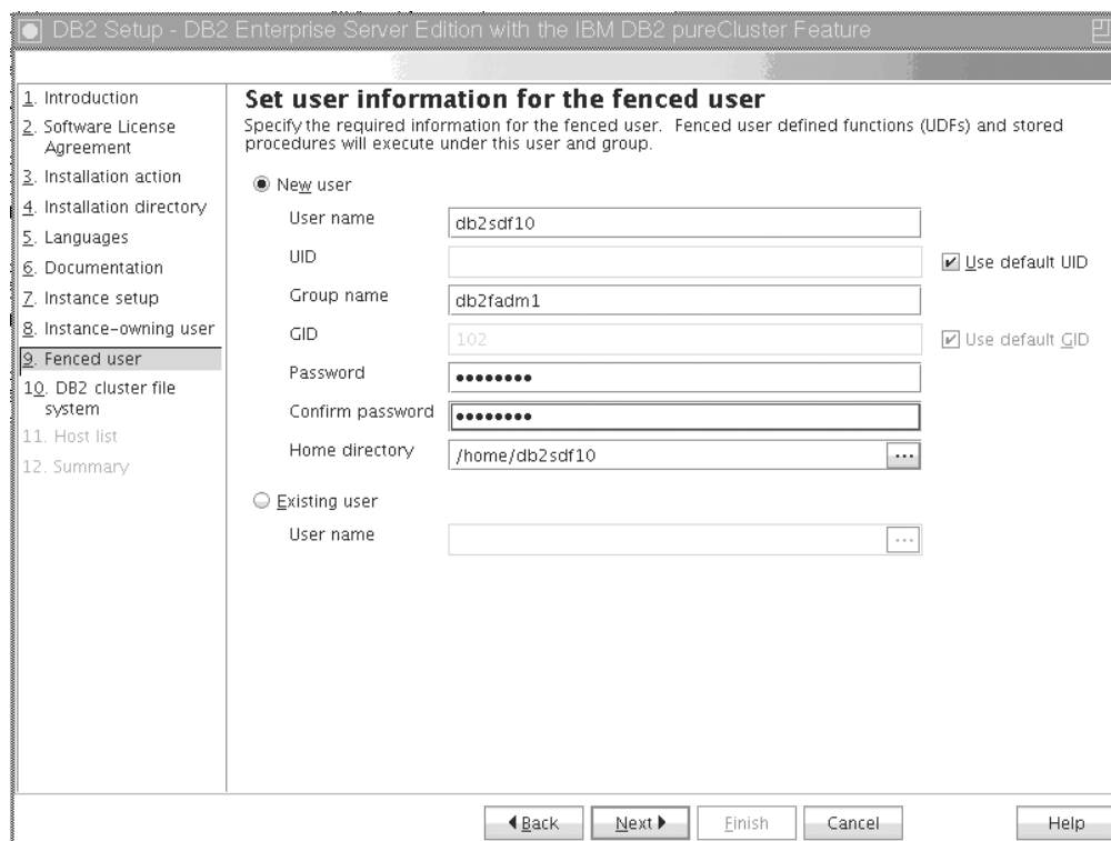
Obrázek 34. Panel Nastavení údajů pro chráněný uživatelský účet
