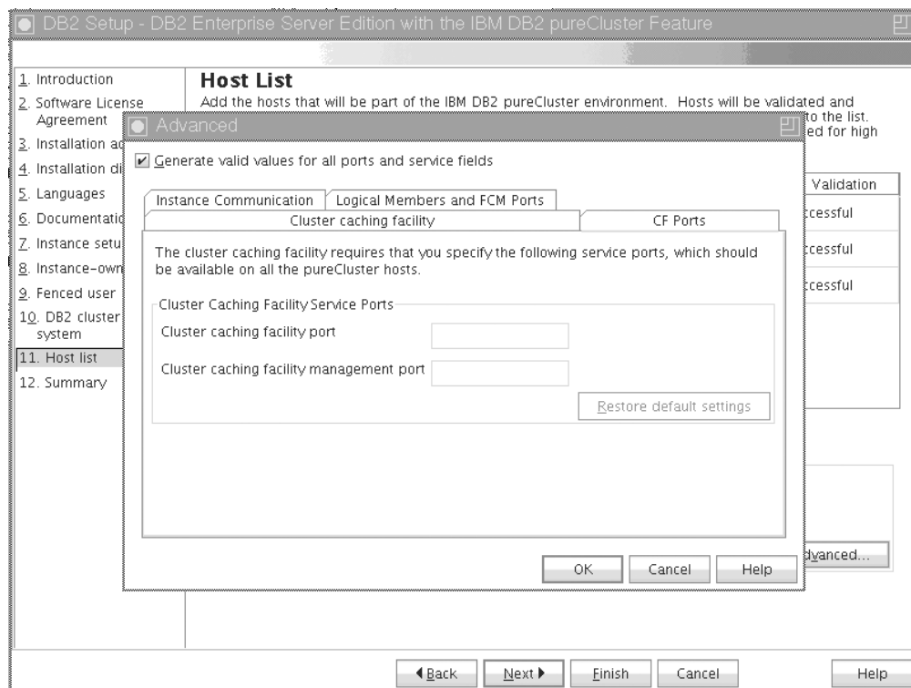
Obrázek 41. Karta Rozšířené nastavení instance - Porty modulu CF
