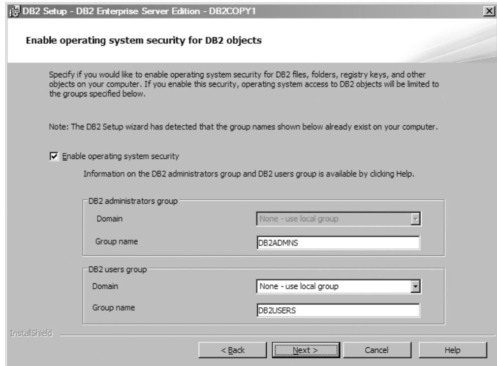
Obrázek 12. Panel Povolení zabezpečení operačního systému pro objekty DB2
