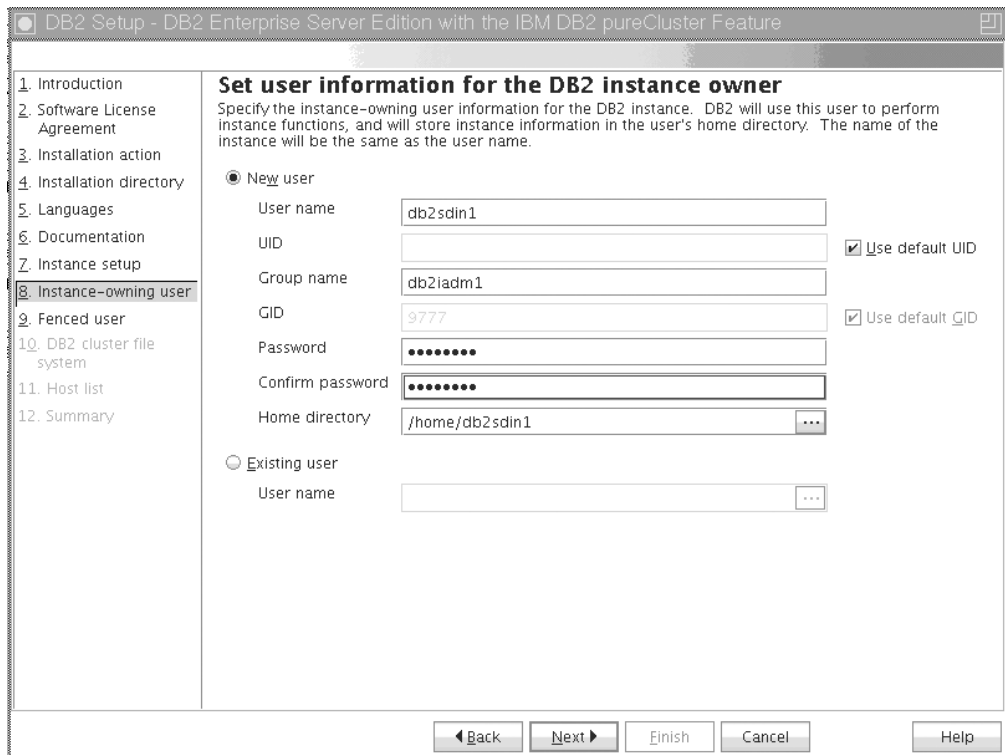
Obrázek 33. Panel Nastavení údajů o uživateli vlastním instancí DB2
