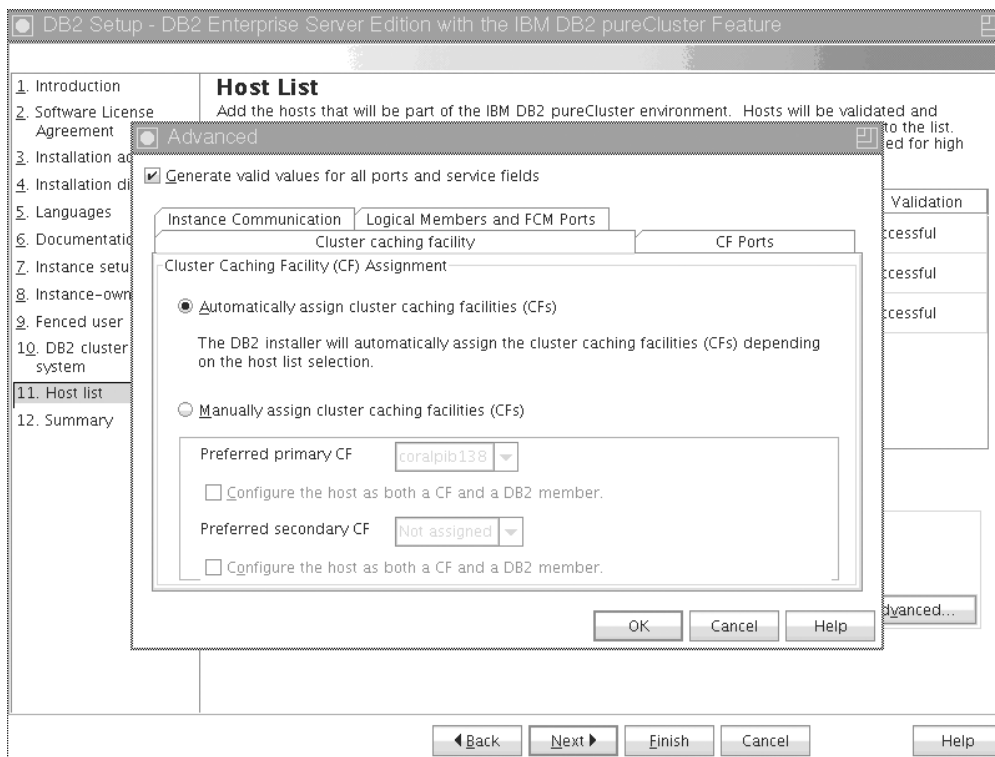
Obrázek 40. Karta Rozšířené nastavení instance - Prostředek mezipaměti klastru
