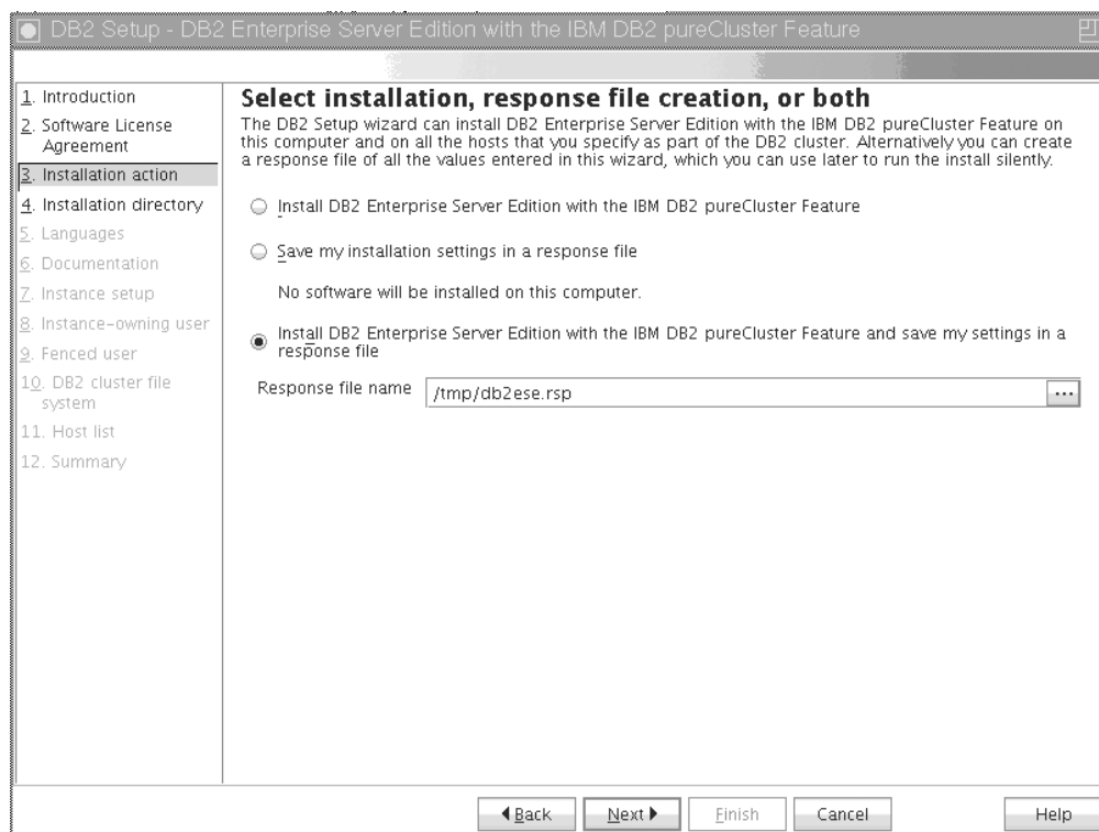
Obrázek 28. Panel Výběr instalace, vytvoření souboru odpovědí, nebo obou voleb
