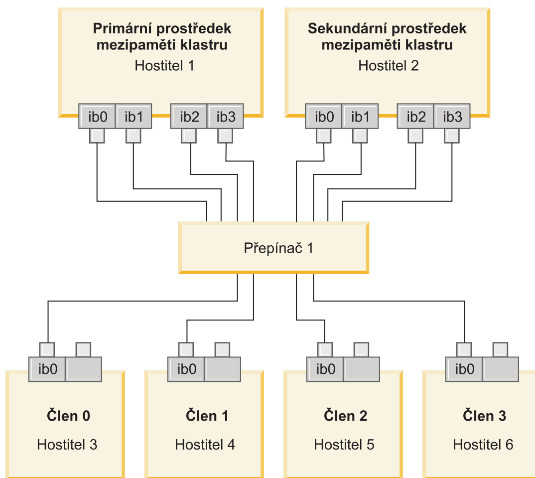
Obrázek 17. Dva moduly CF a čtyři členové se připojují k jednomu přepínači.
