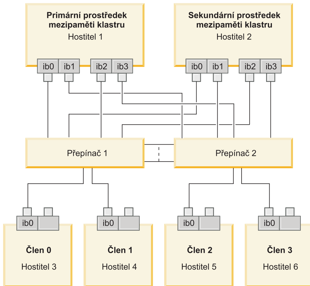
Obrázek 18. Dva moduly CF a čtyři členové se připojují ke dvěma přepínačům.
