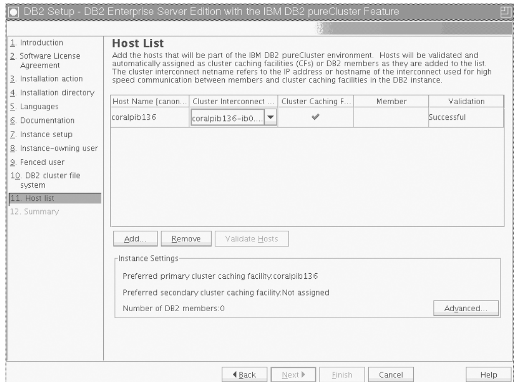
Obrázek 36. Panel Seznam hostitelů
