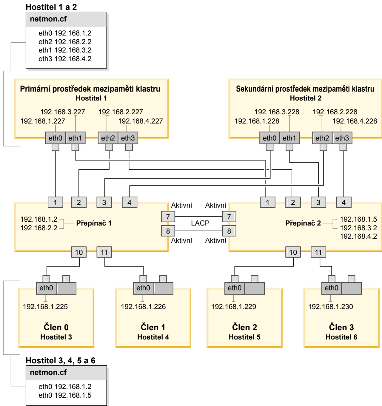
Obrázek 21. Dva moduly CF a čtyři členové se připojují ke dvěma přepínačům.
