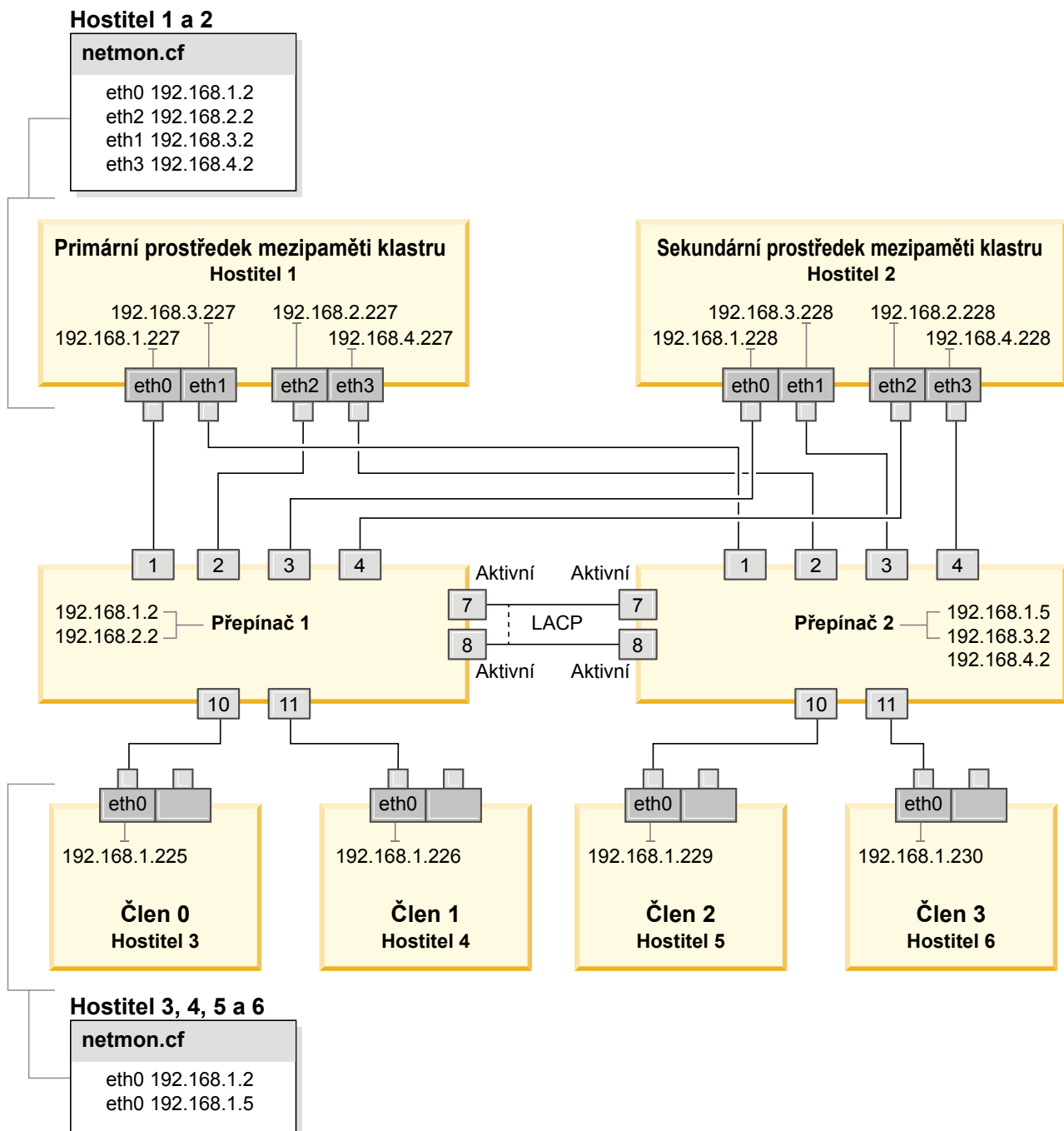
Obrázek 23. Dva moduly CF a čtyři členové se připojují ke dvěma přepínačům.
