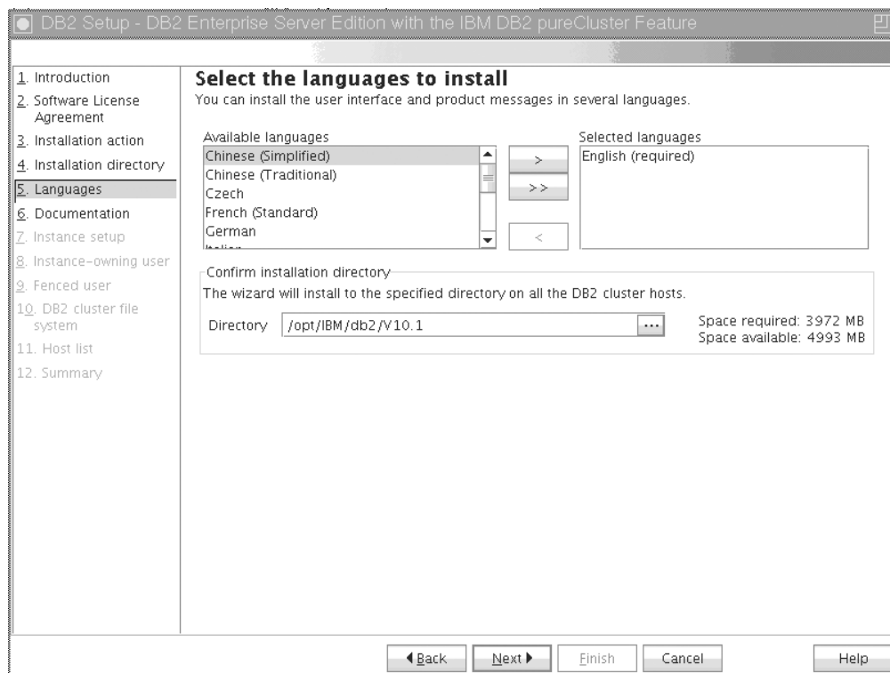
Obrázek 30. Panel Výběr instalovaných jazyků
