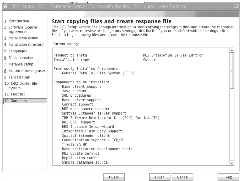
Obrázek 44. Panel Souhrn
