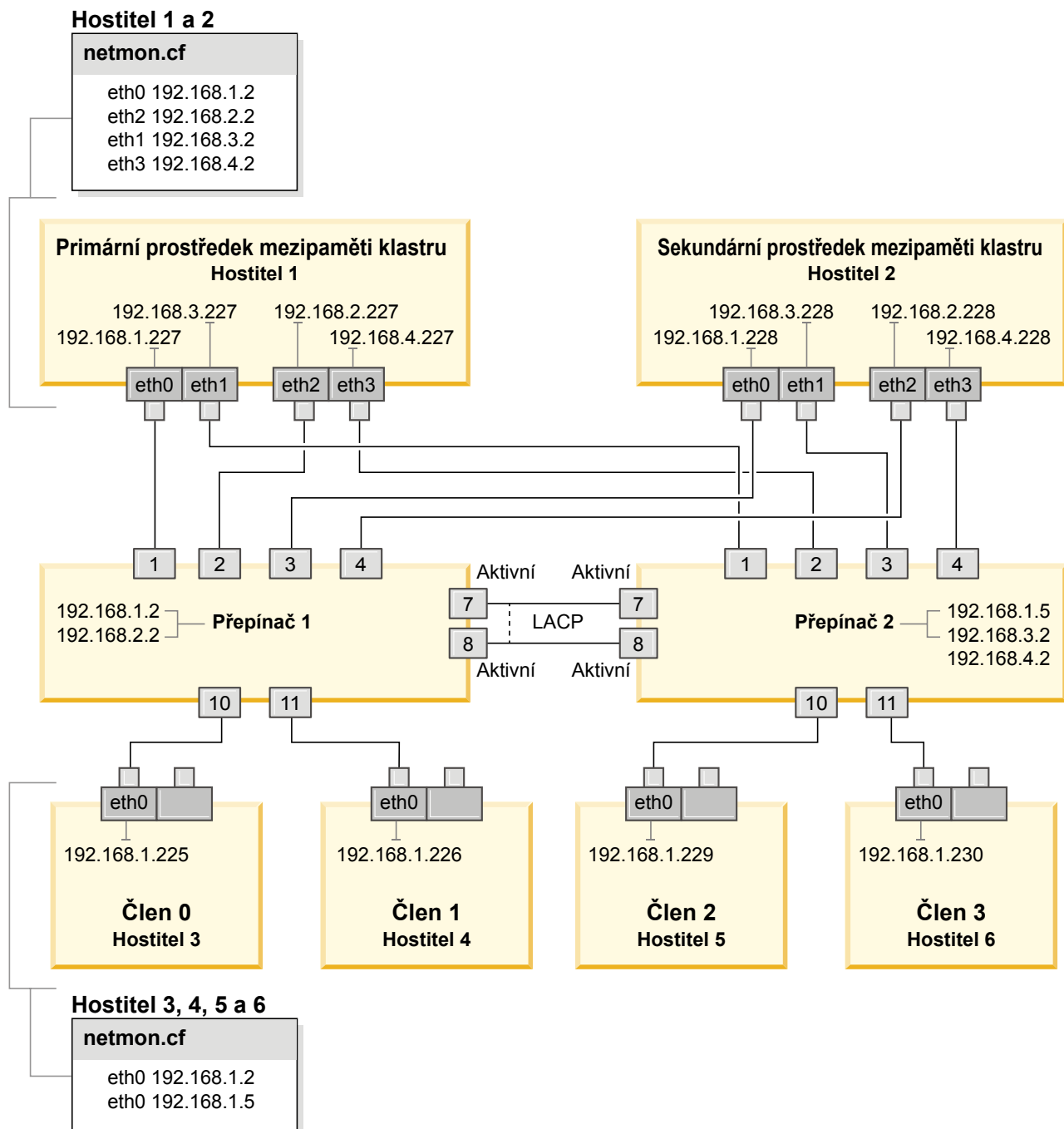
Obrázek 22. Dva moduly CF a čtyři členové se připojují ke dvěma přepínačům.
