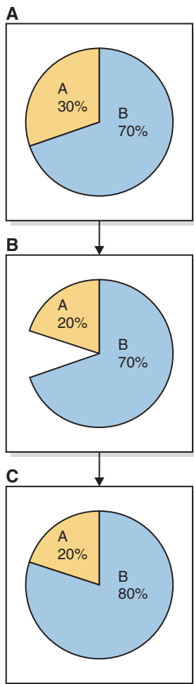
Figura 35. Límite de CPU y varias superclases: Escenario 1
