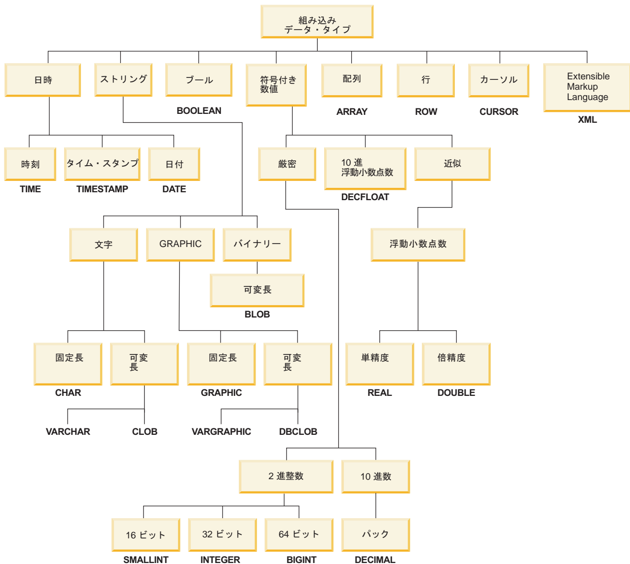
図 34. 組み込みデータ・タイプ
