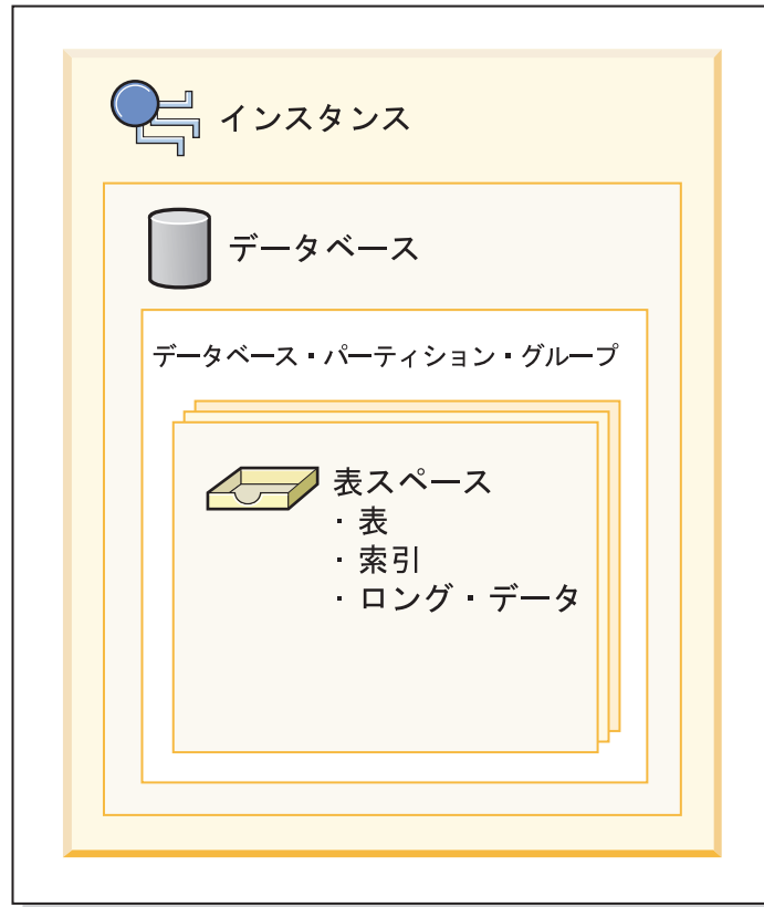
図 42. 一部のデータベース・オブジェクトの相互関係
