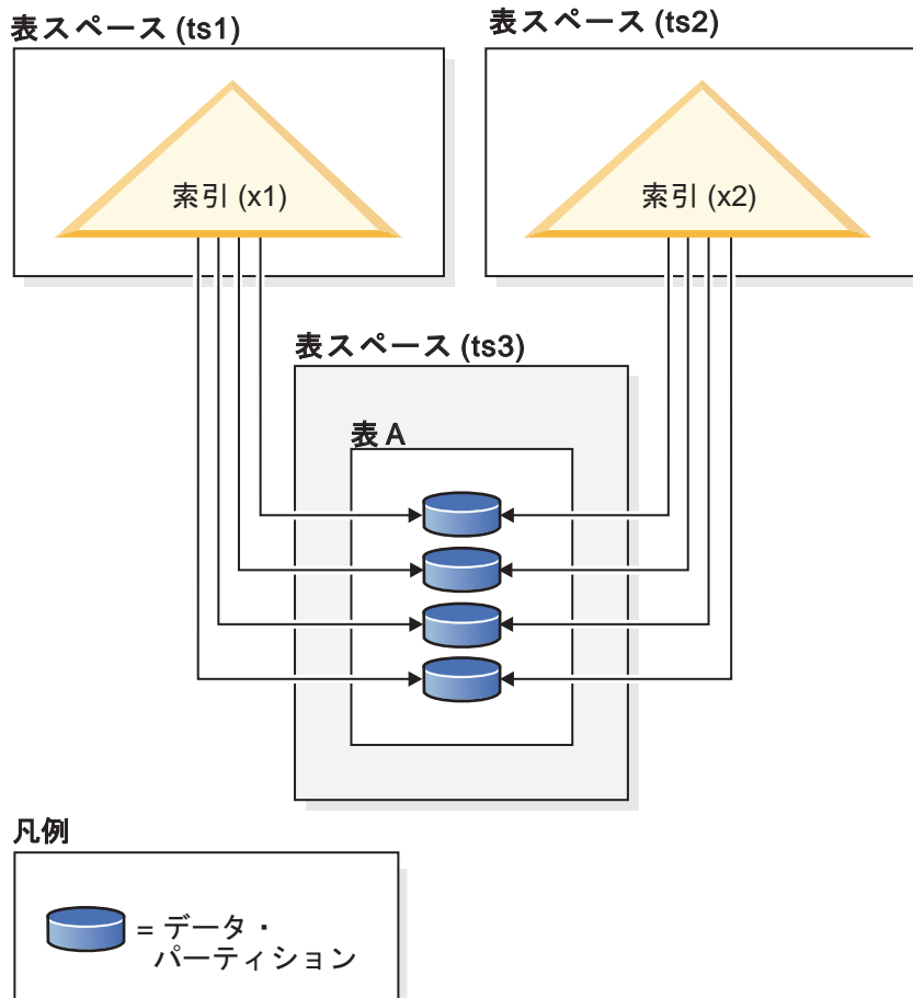
図 44. それぞれ独自表スペースに索引があるパーティション表の非パーティション索引
