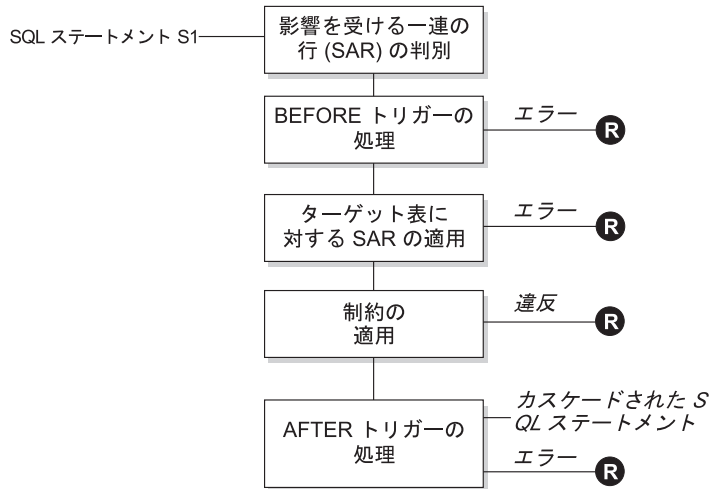
図 50. 関連するトリガーと制約を伴うステートメントの処理
