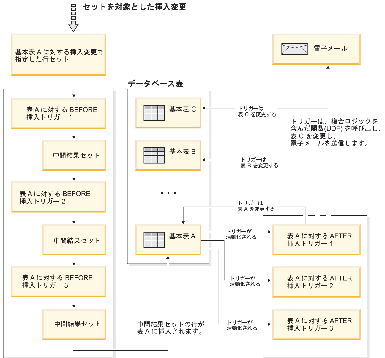
図 49. トリガー実行モデル
