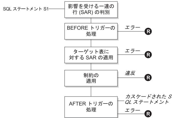
図 40. 関連するトリガーと制約を伴うステートメントの処理
