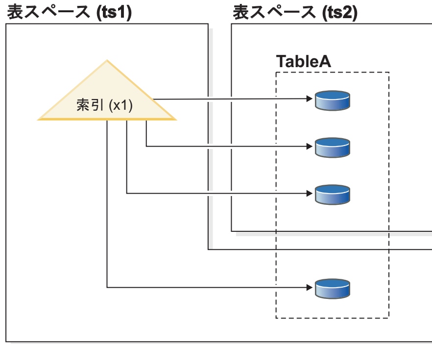
図 43. パーティション表の非パーティション索引
