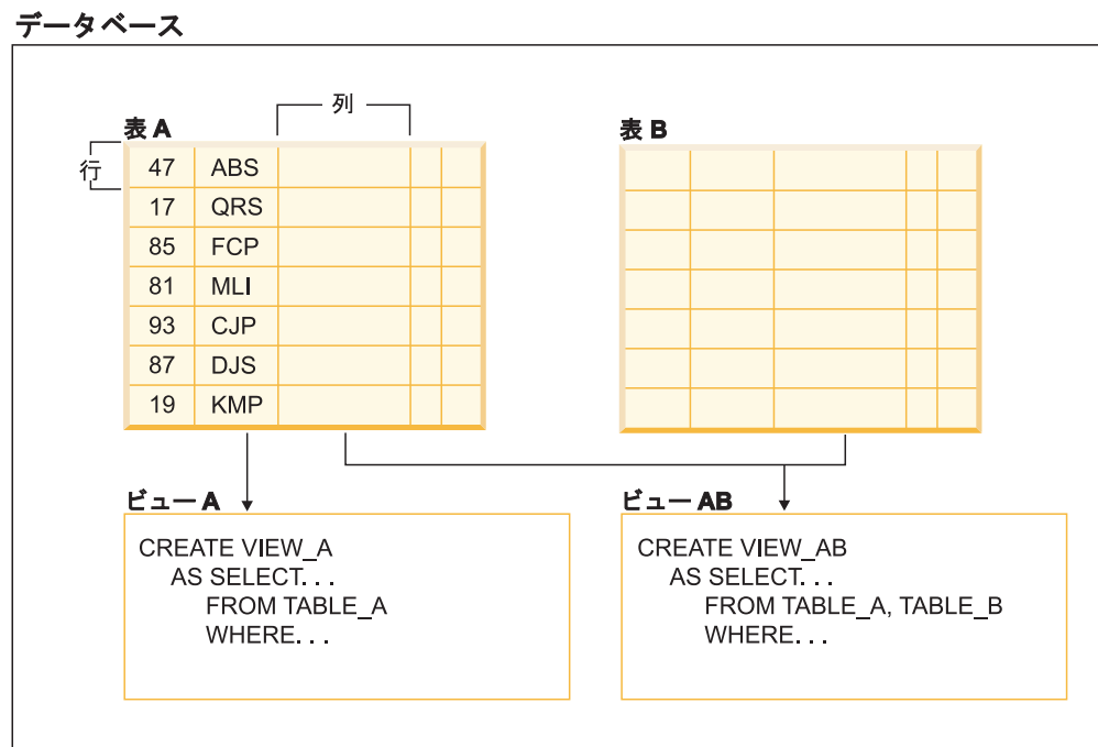
図 51. 表とビューの関係
