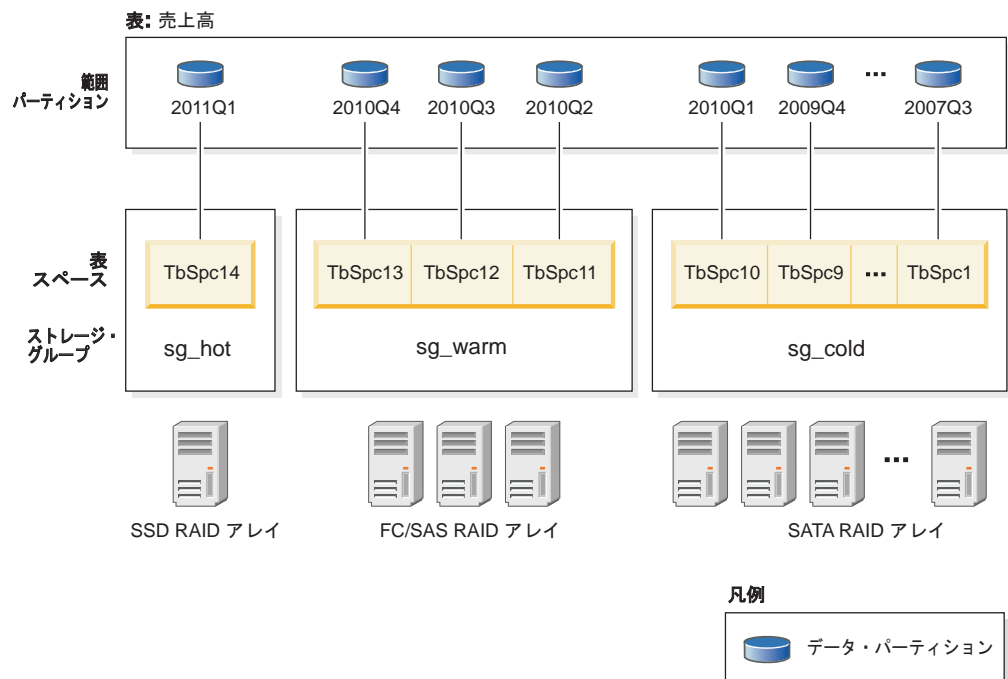
図 32. Multi-Temperature Data Storage を使った販売データの管理
