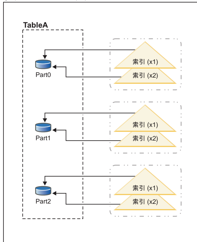
図 45. 1 つの表のデータ・パーティションと表スペースを共有するパーティション索引
