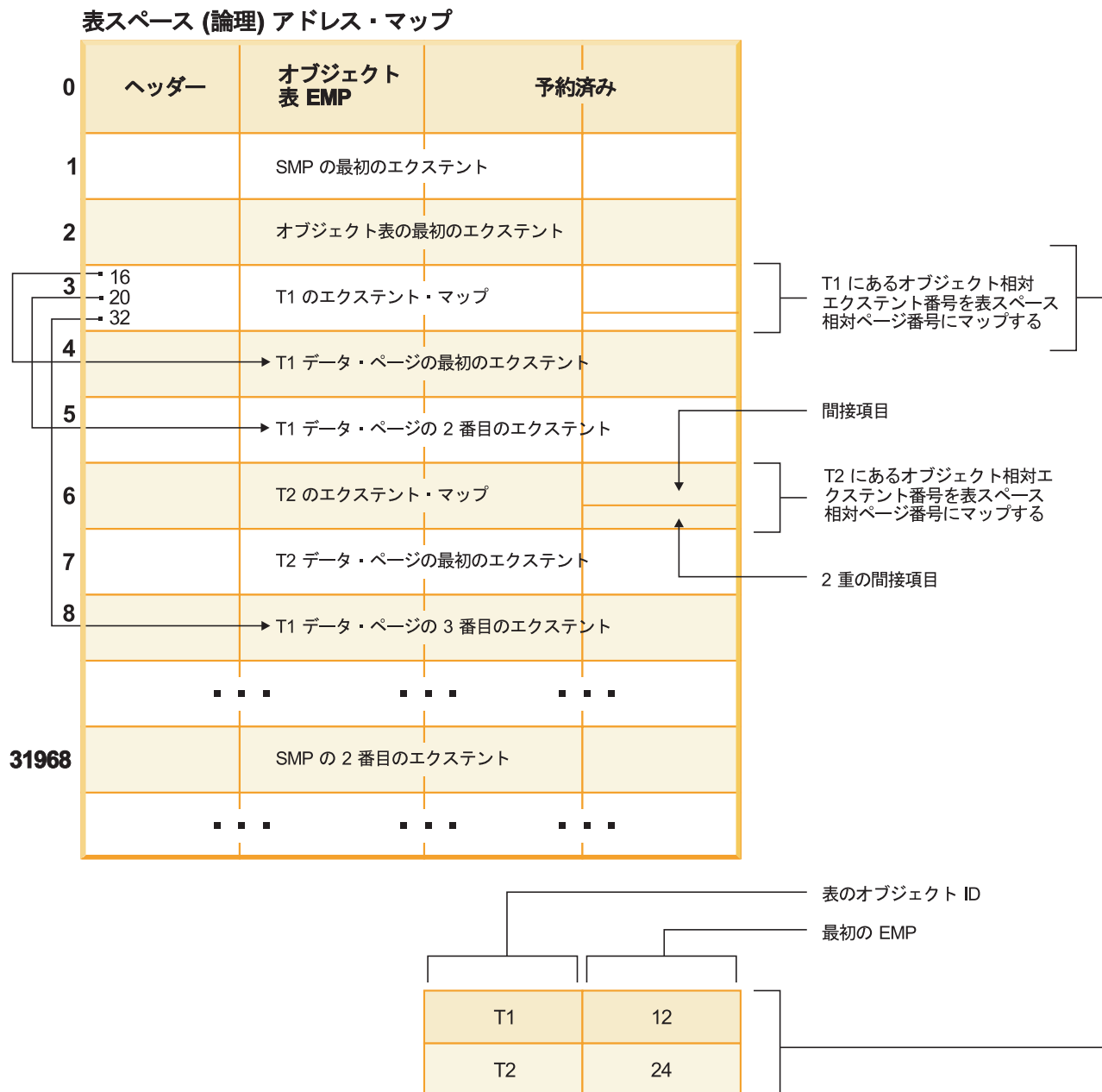
図 10. DMS 表スペース
