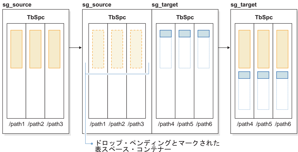
図 31. 新規ストレージ・グループへの表スペースの移動
