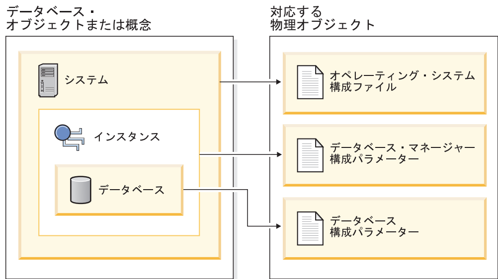
図 52. データベース・オブジェクトと構成ファイルの関係
