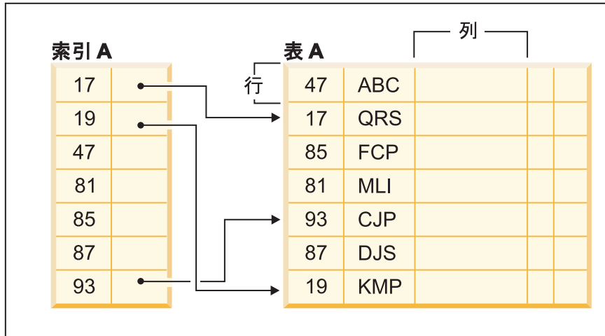
図 41. 索引と表の関係
