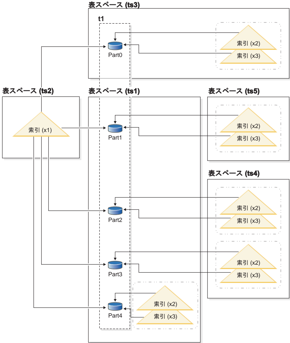
図 47. パーティション表の非パーティション索引とパーティション索引の組み合わせ
