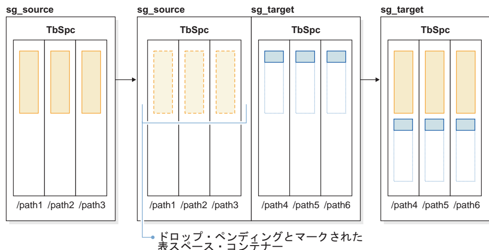
図 33. 新規ストレージ・グループへの表スペースの移動
