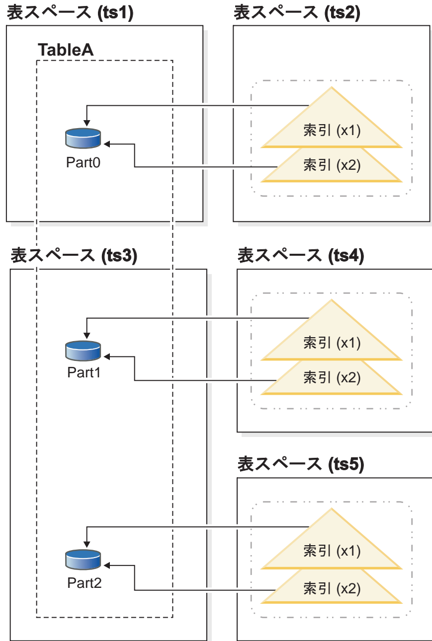
図 46. データ・パーティションと索引パーティションが異なる表スペースにあるパーティション索引
