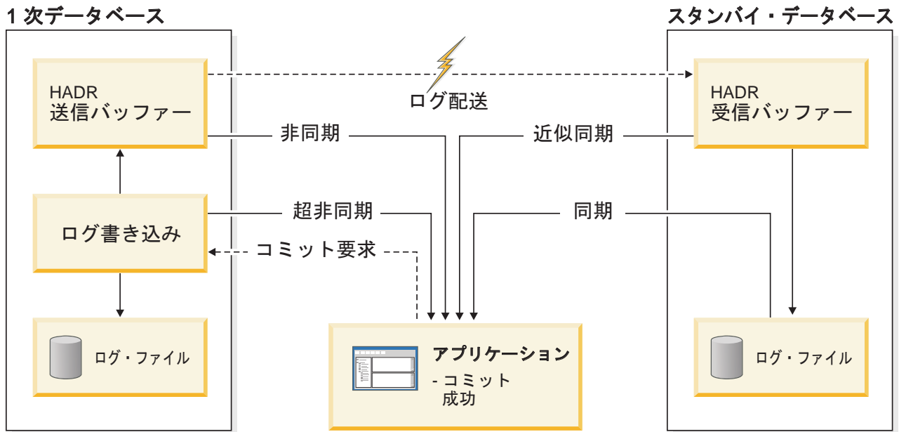
図 53. 高可用性災害時リカバリー (HADR) 用の同期モード
