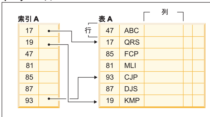
図 1. 索引と表の関係
