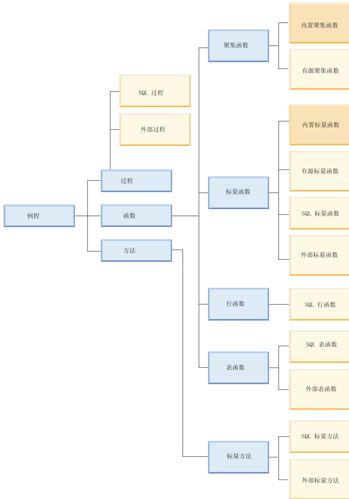
图 1. 例程分类
