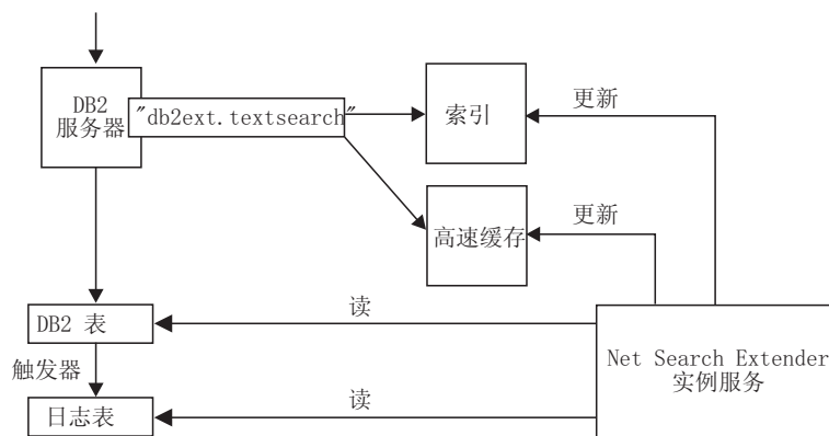
图 5. 使用存储过程搜索
