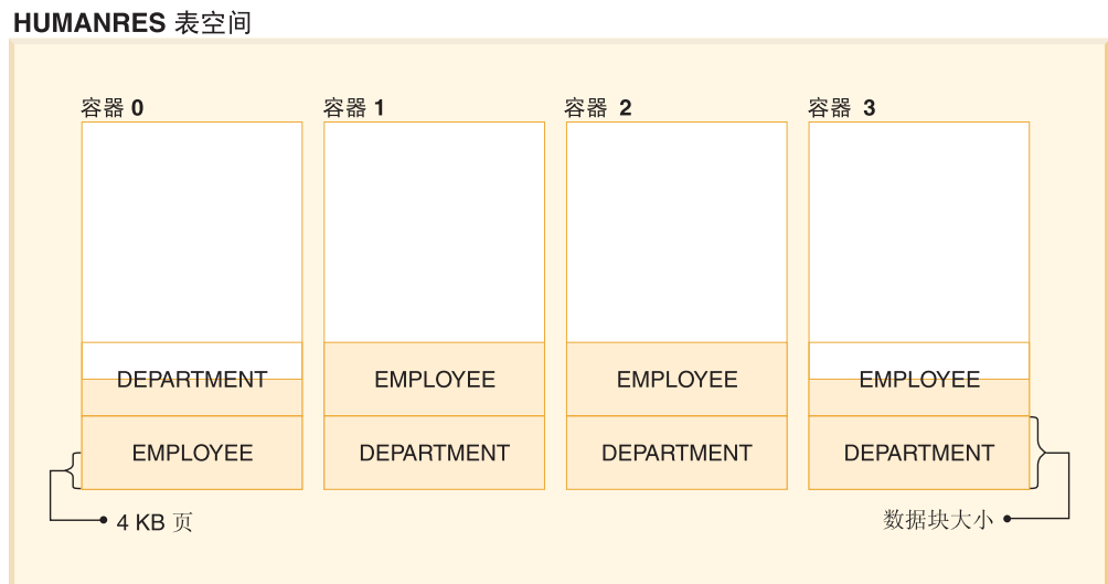
图 28. 表空间中的容器和扩展数据块
