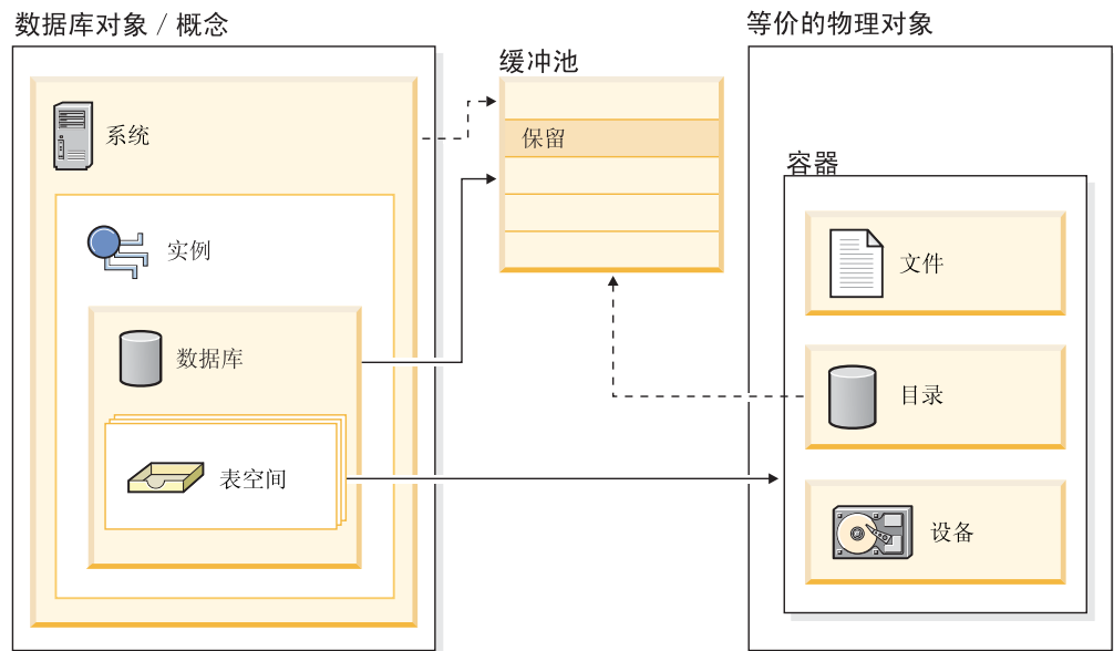
图 8. 缓冲池与容器之间的关系
