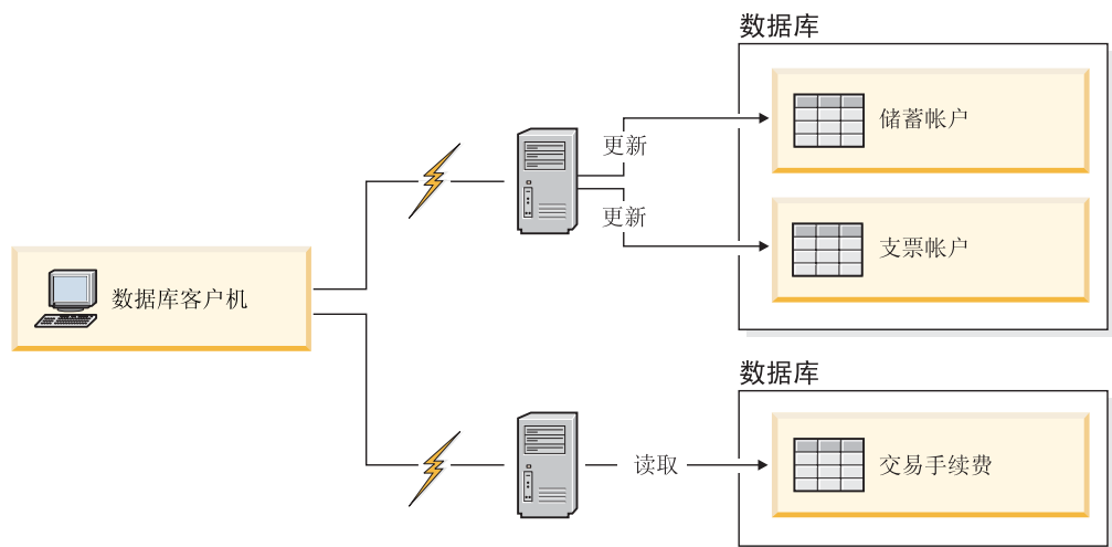
图 59. 在单个事务中使用多个数据库
