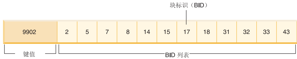
图 46. “YearAndMonth” 的维块索引中的键
