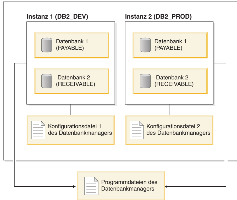
Abbildung 3. Hierarchische Beziehung zwischen DB2-Systemen, -Instanzen und -Datenbanken
