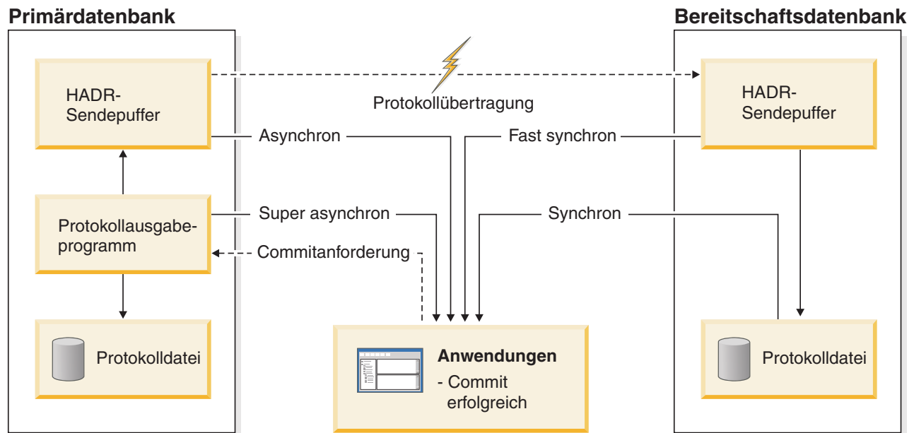
Abbildung 49. Synchronisationsmodi für HADR (High Availability and Disaster Recovery)
