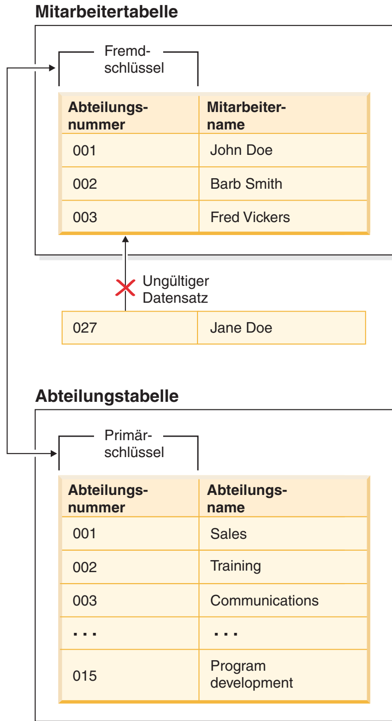
Abbildung 36. Integritätsbedingungen über Fremd- und Primärschlüssel
