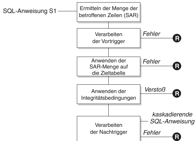
Abbildung 37. Verarbeitung einer Anweisung mit definierten Triggern und Integritätsbedingungen
