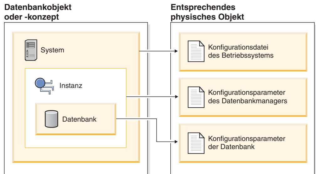
Abbildung 48. Beziehung zwischen Datenbankobjekten und Konfigurationsdateien
