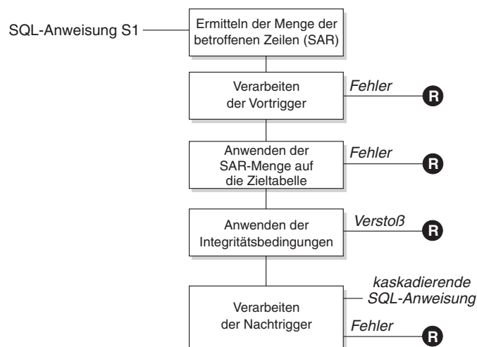
Abbildung 46. Verarbeitung einer Anweisung mit definierten Triggern und Integritätsbedingungen
