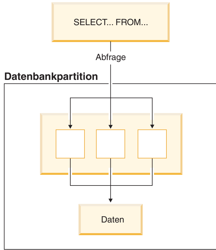
Abbildung 28. Partitionsinterne Parallelität
