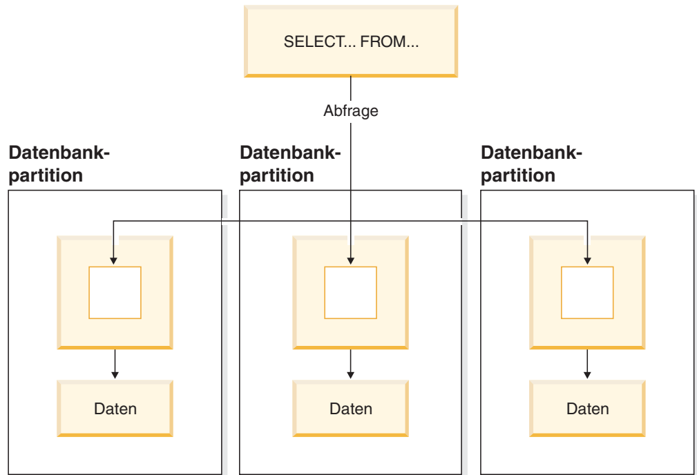
Abbildung 29. Partitionsübergreifende Parallelität
