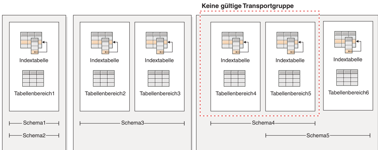
Abbildung 25. Tabellenbereichs- und Schemagruppen
