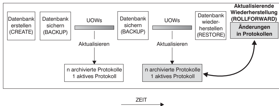
Abbildung 20. Aktualisierende Recovery einer Datenbank. Im Falle einer lange laufenden Transaktion kann es mehr als ein aktives Protokoll geben.
