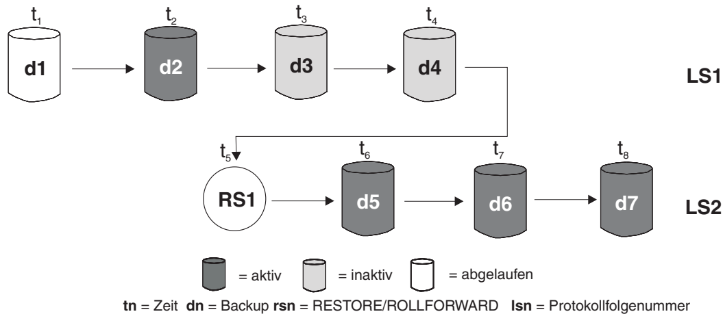
Abbildung 16. Gemischte aktive, inaktive und abgelaufene Datenbankbackups
