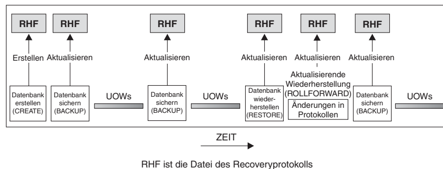
Abbildung 12. Erstellen und Aktualisieren der Datei des Recoveryprotokolls
