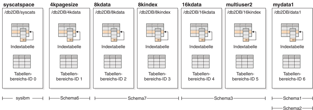
Abbildung 28. Datenbank TARGETDB nach dem Transport
