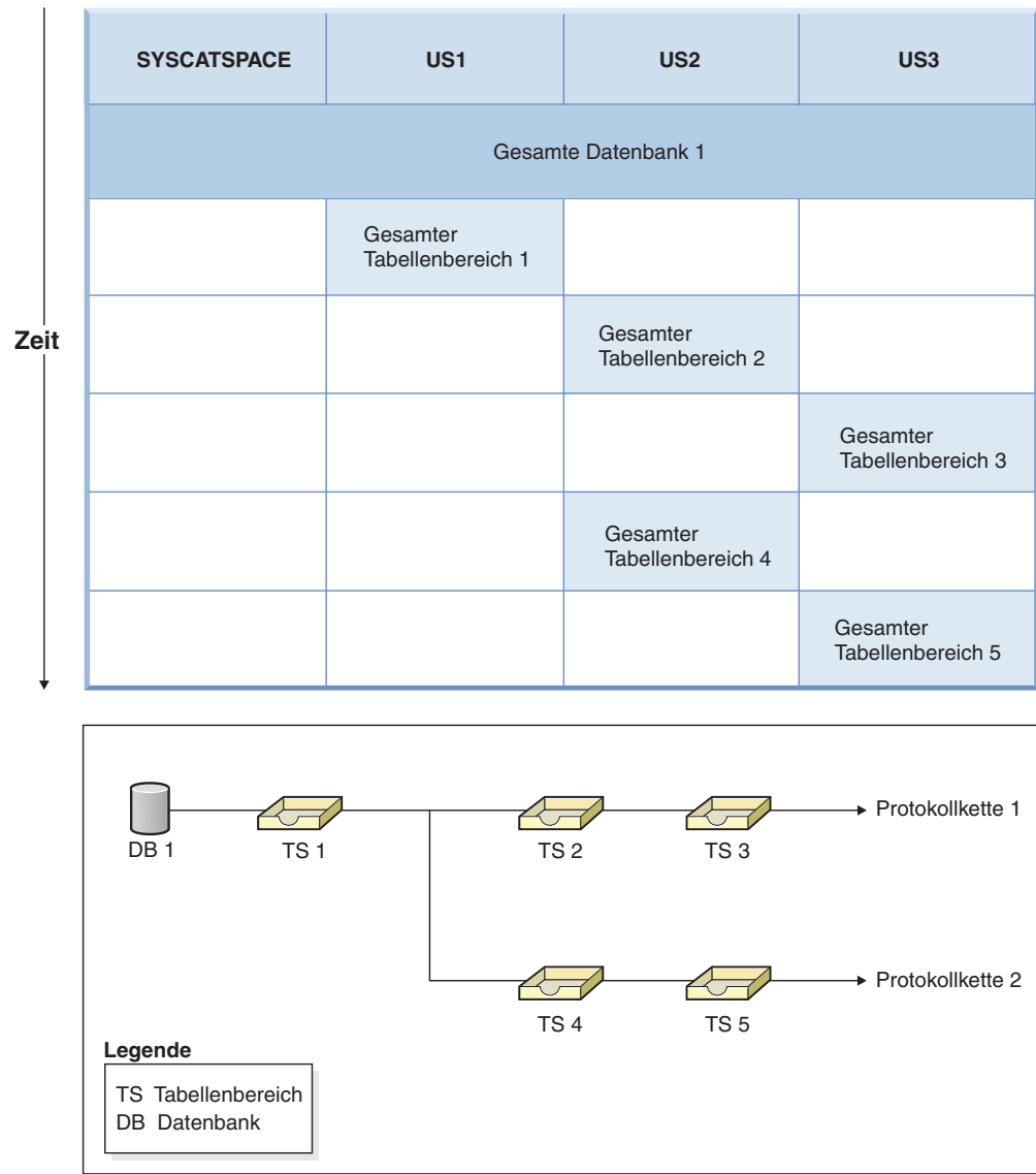
Abbildung 22. Backups auf Datenbank- und Tabellenbereichsebene der Datenbank SAMPLE
