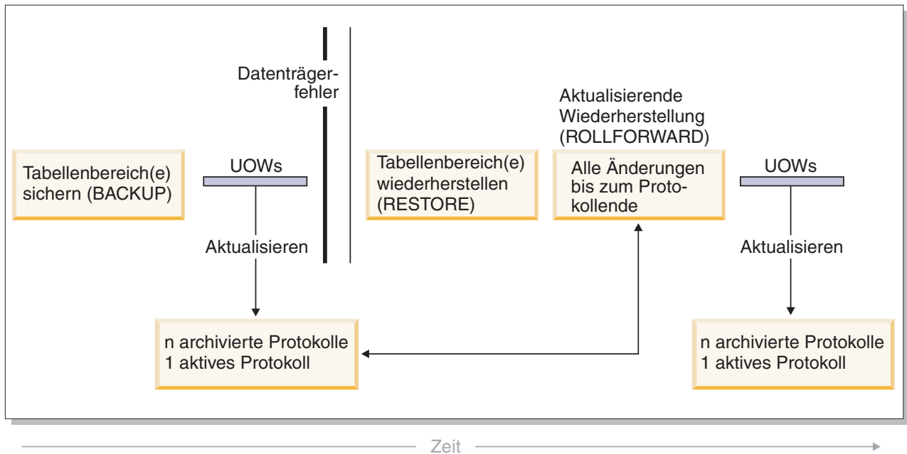
Abbildung 21. Aktualisierende Recovery von Tabellenbereichen. Im Falle einer lange laufenden Transaktion kann es mehr als ein aktives Protokoll geben.
