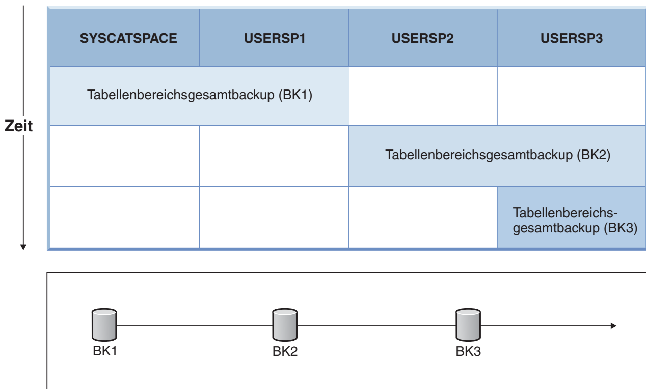
Abbildung 24. Für die Datenbank SAMPLE verfügbare Backup-Images
