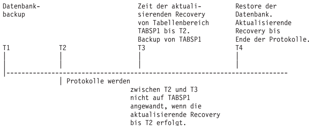
Abbildung 29. Backup-Anforderung für Tabellenbereiche
