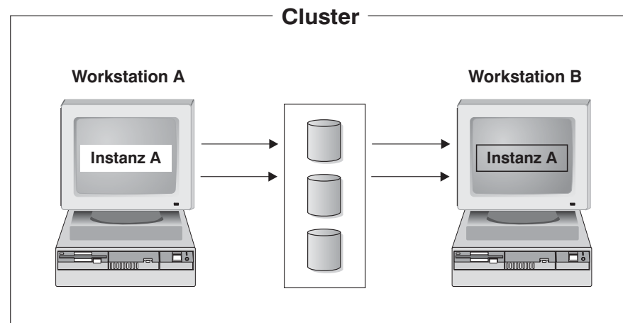
Abbildung 5. Aktive/Passive Konfiguration
