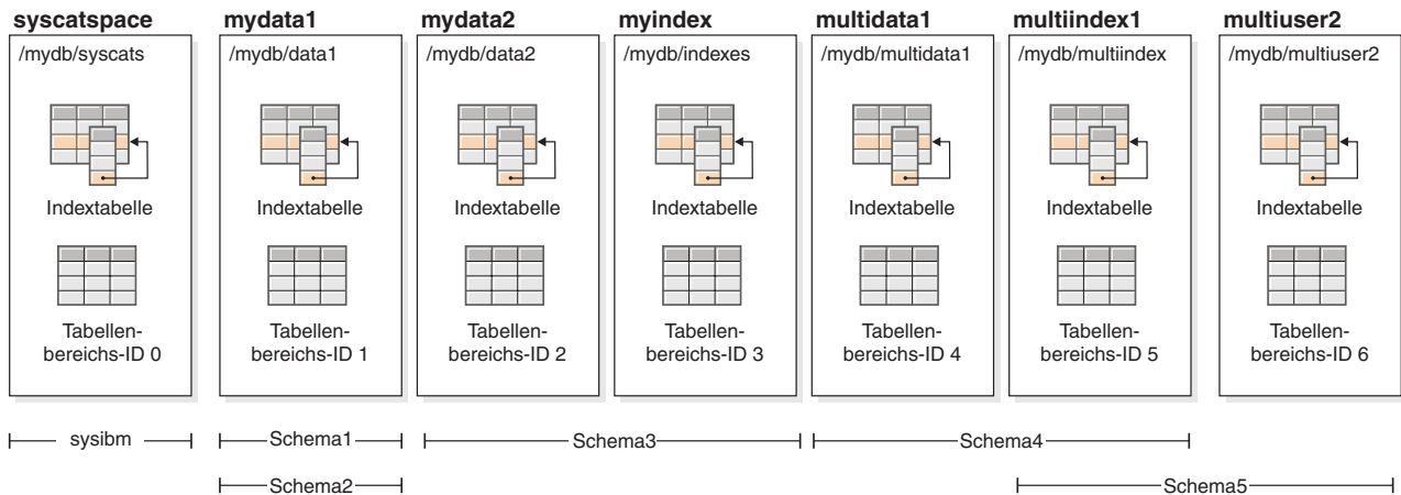
Abbildung 26. Datenbank ORIGINALDB
