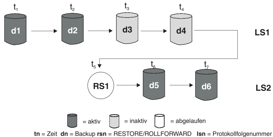
Abbildung 14. Inaktive Datenbankbackups
