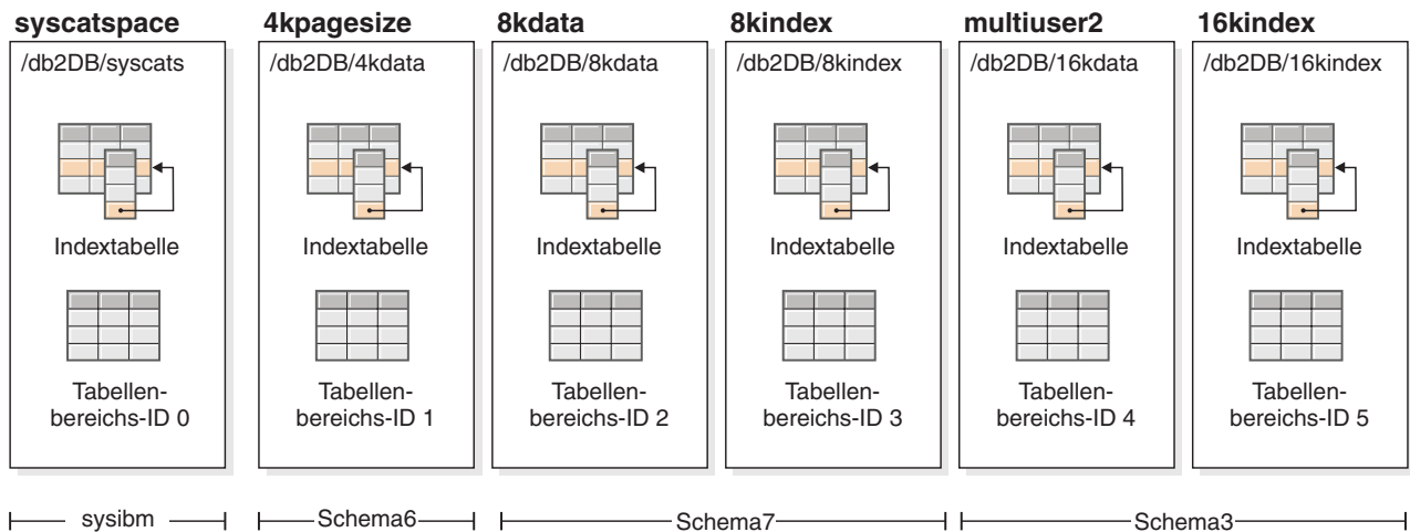
Abbildung 27. Datenbank TARGETDB
