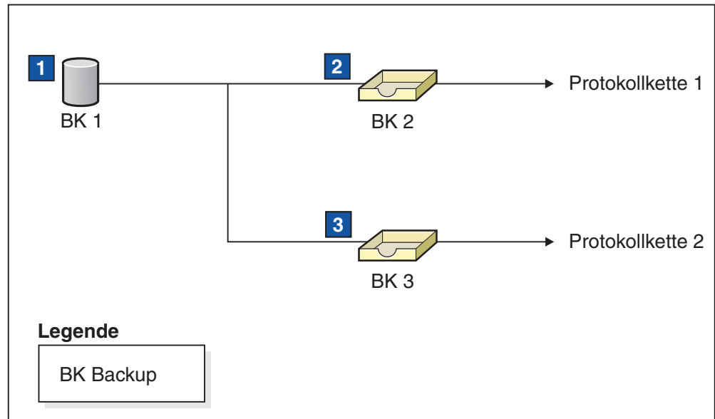
Abbildung 23. Backup-Protokollkette für die Datenbank SAMPLE2
