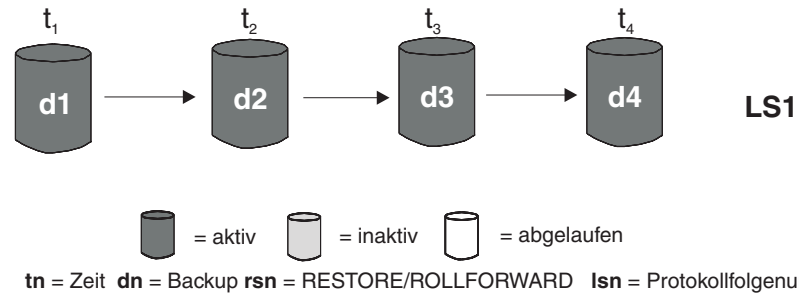
Abbildung 13. Aktive Datenbankbackups. Der Wert von num_db_backups wurde auf vier gesetzt.
