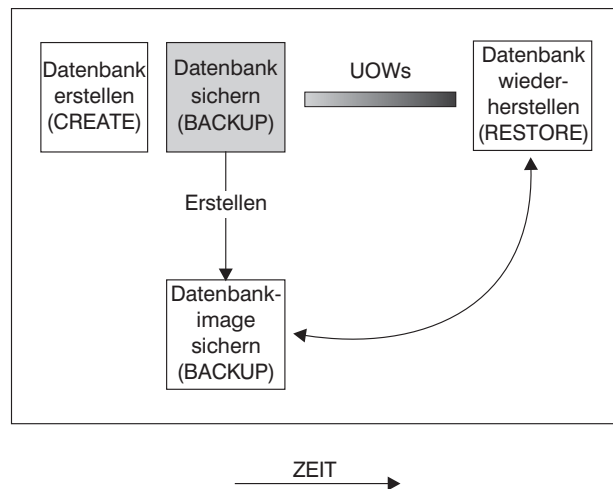
Abbildung 19. Versionsrecovery . Zeigt an, dass alle UOWs verloren gehen, die vom Zeitpunkt des Backups ausgehend bis zum Eintreten des Fehlers ausgeführt wurden.
