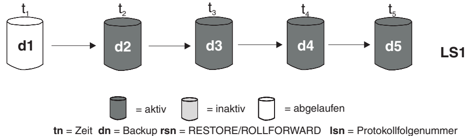
Abbildung 15. Abgelaufene Datenbankbackups
