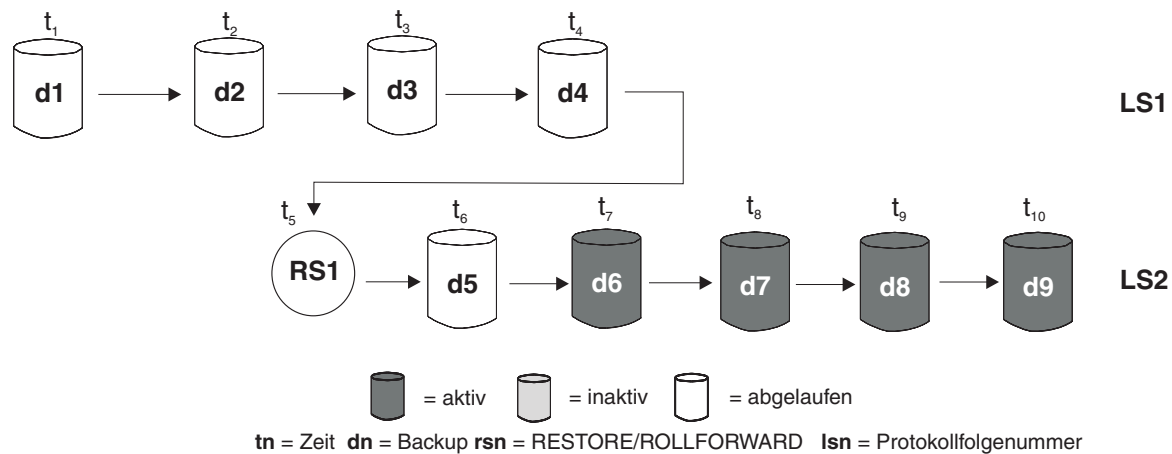
Abbildung 17. Abgelaufene Protokollfolge
