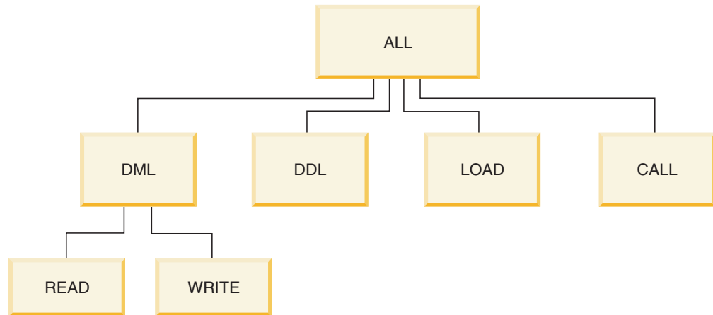
Abbildung 8. Arbeitstypschlüsselwörter
