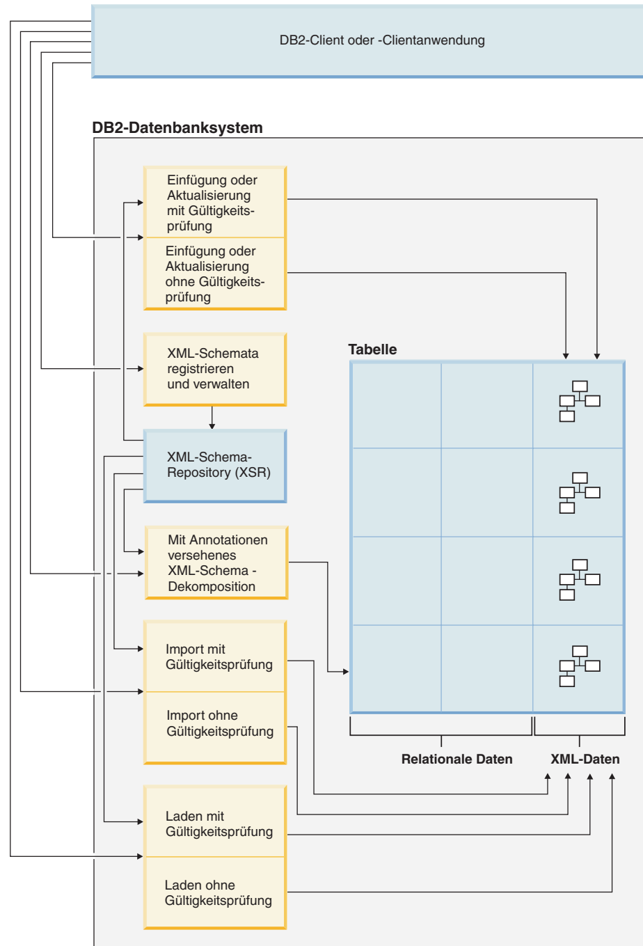
Abbildung 1. Methoden zur Eingabe von XML-Daten
