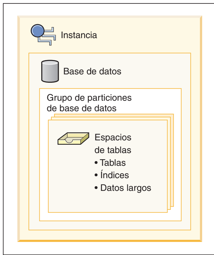
Figura 2. Relaciones entre objetos de base de datos seleccionados
