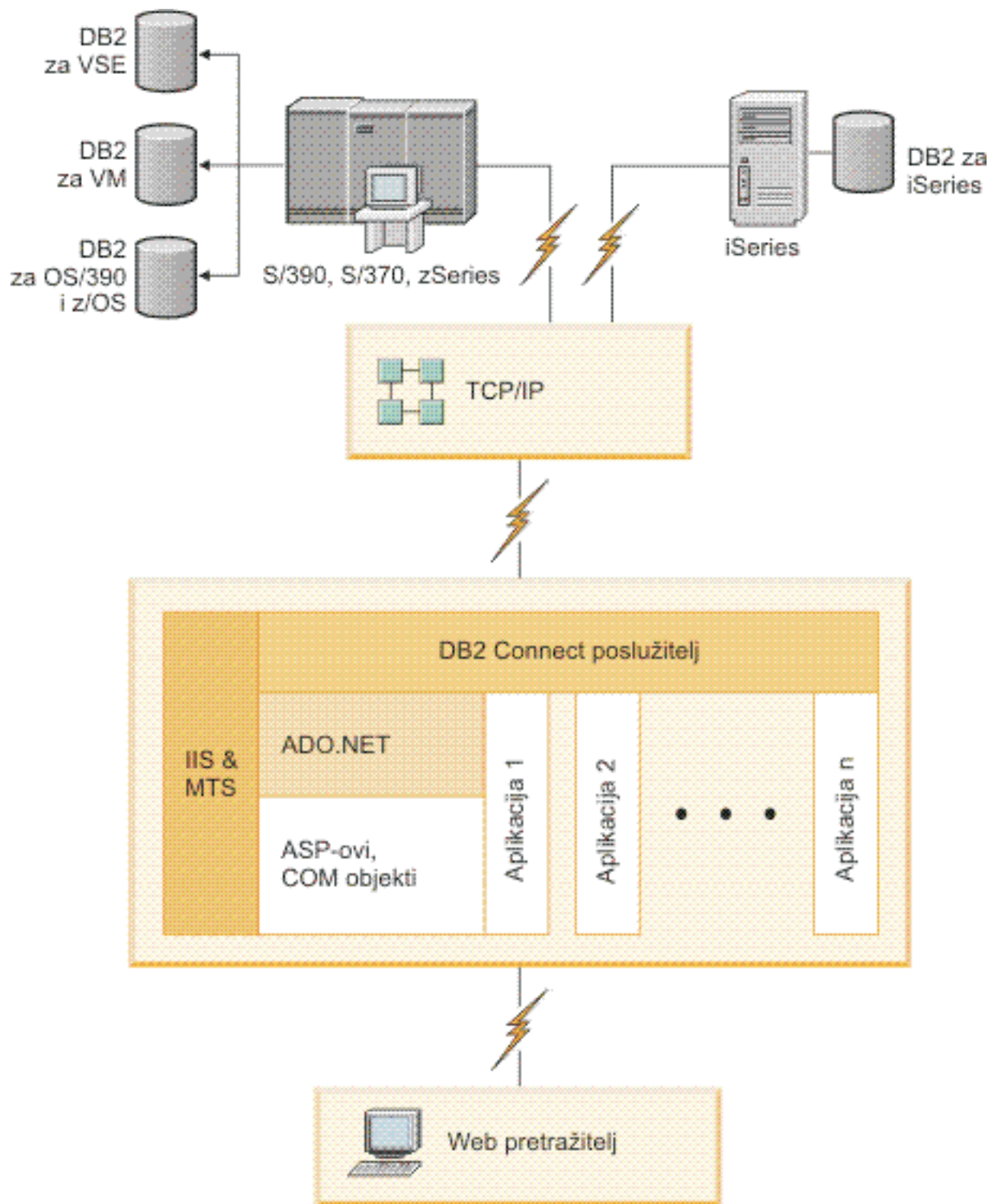
Slika 5. DB2 Connect koji radi s poslužiteljem Microsoft Internetkih informacija (IIS)
