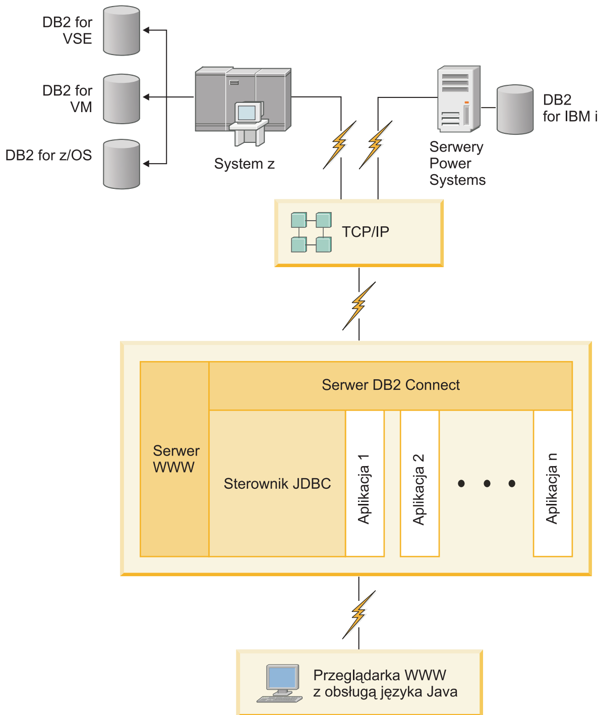
Rysunek 1. JDBC i DB2 Connect
