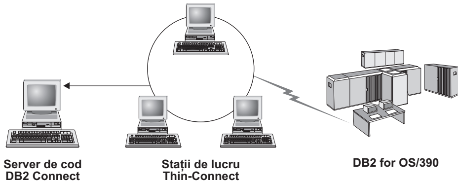
Figura 3. O topologie tipică de client subțire folosind DB2 Connect Personal Edition
