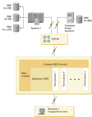
Рисунок 1. JDBC и DB2 Connect
