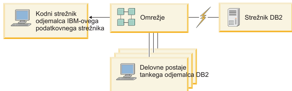
Slika 2. Značilna topologija tankega odjemalca, s pomočjo odjemalca IBM-ovega podatkovnega strežnika
