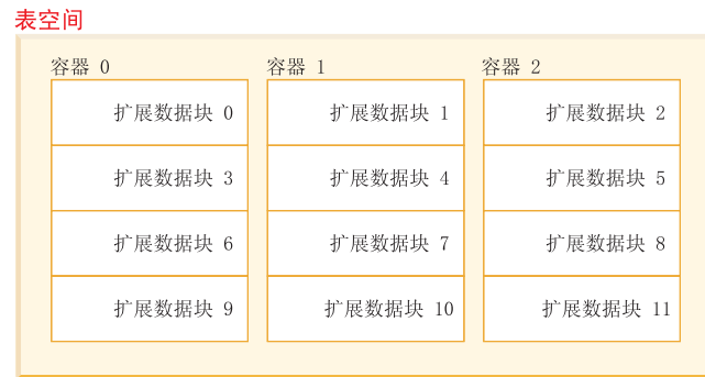
图 11. 带有三个容器和 12 个扩展数据块的表空间
