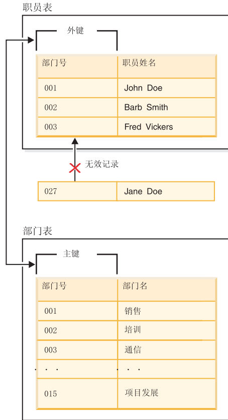
图 36. 外键和主键约束
