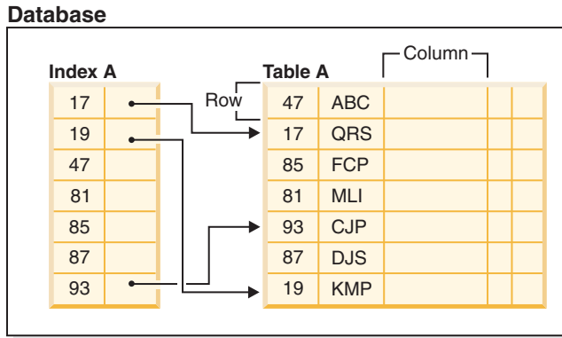
图 38. 索引与表之间的关系
