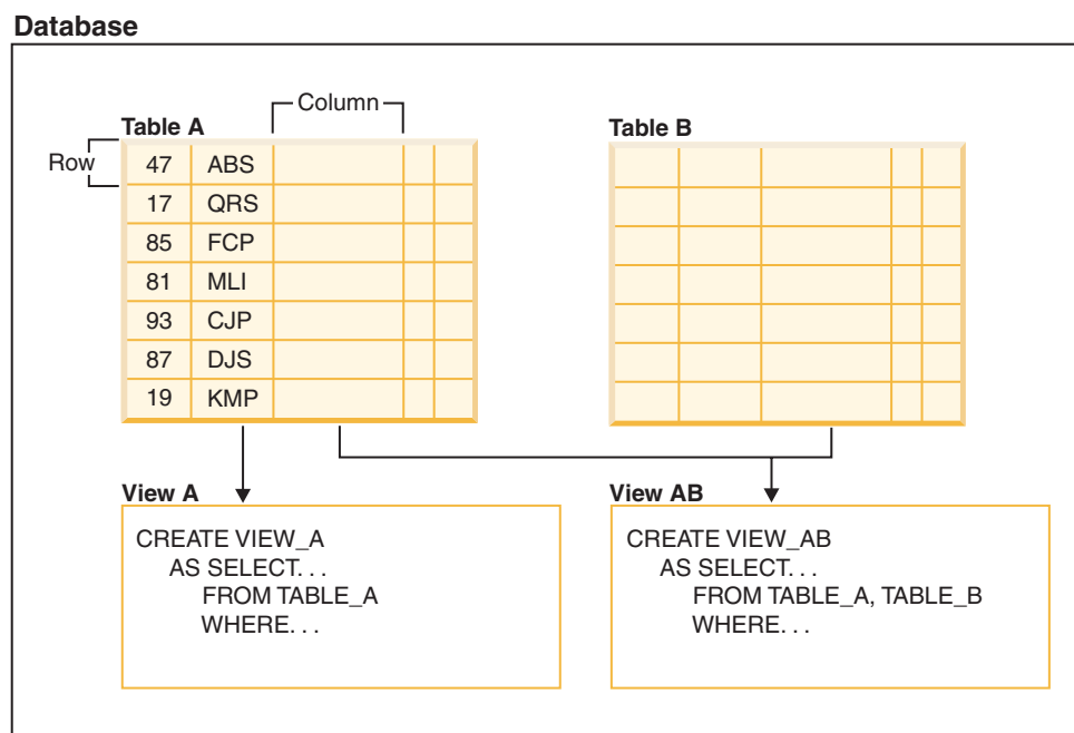
图 47. 表与视图之间的关系
