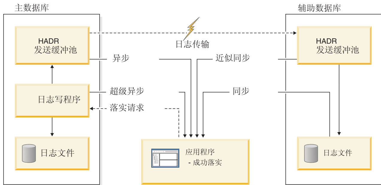
图 49. 高可用性和灾难恢复 (HADR) 的同步方式
