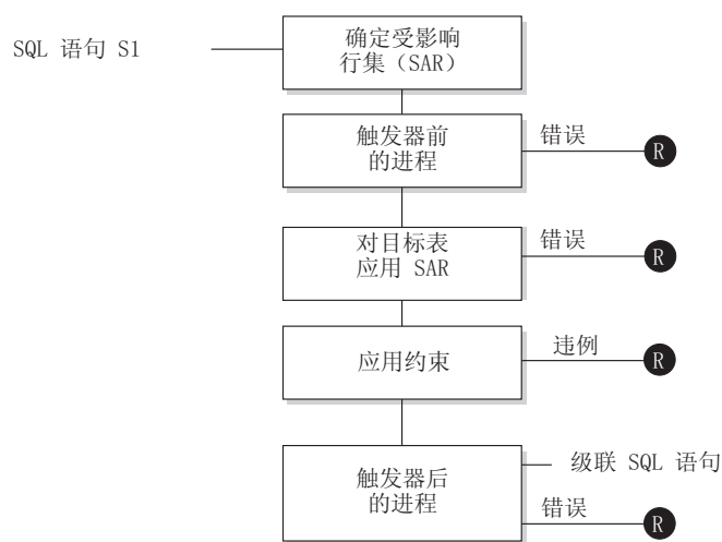
图 37. 处理包含相关触发器和约束的语句
