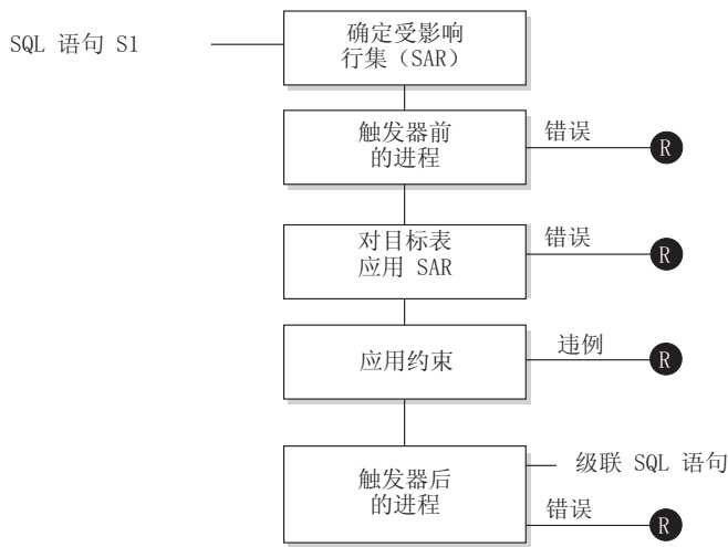
图 46. 处理包含相关触发器和约束的语句
