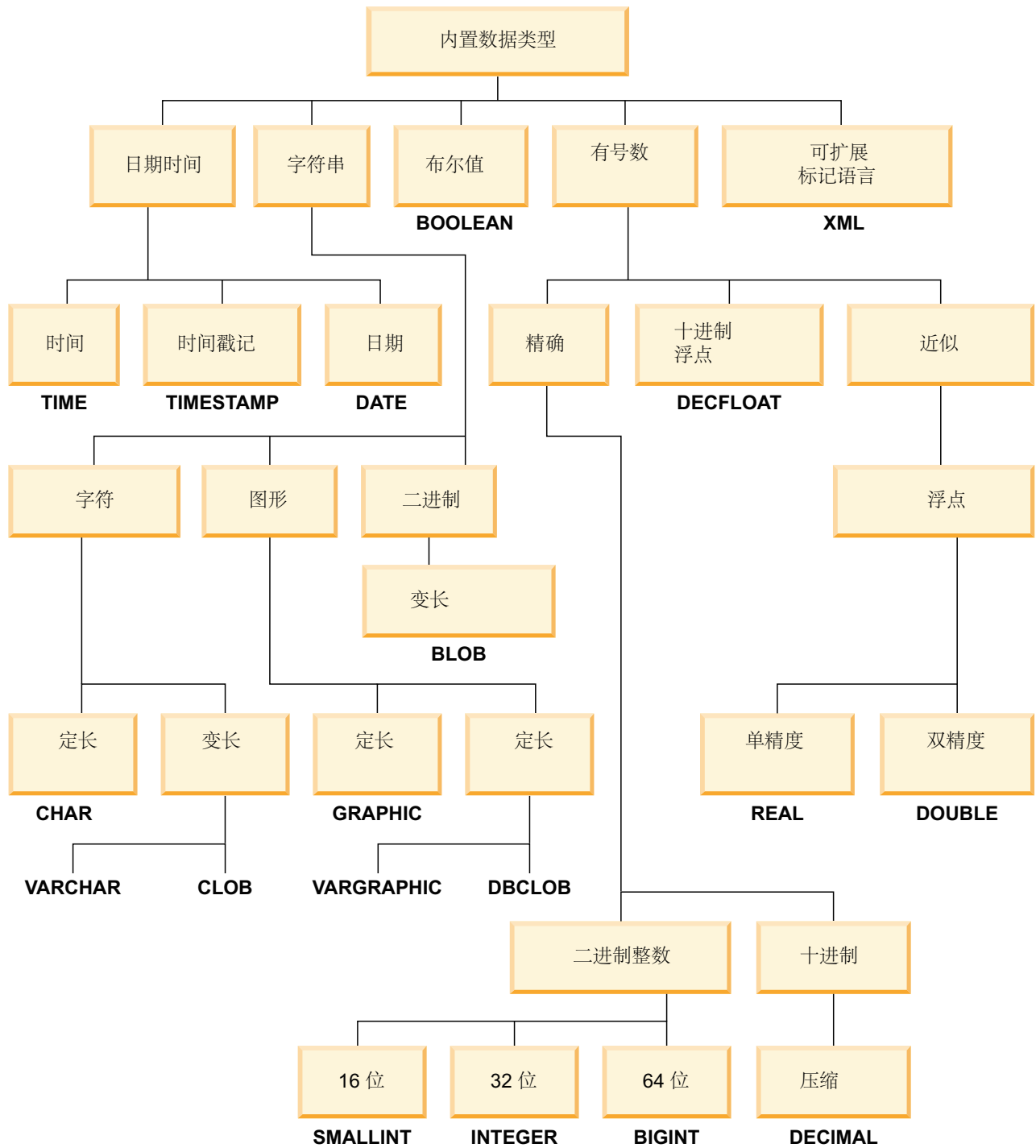
图 31. 内置数据类型
