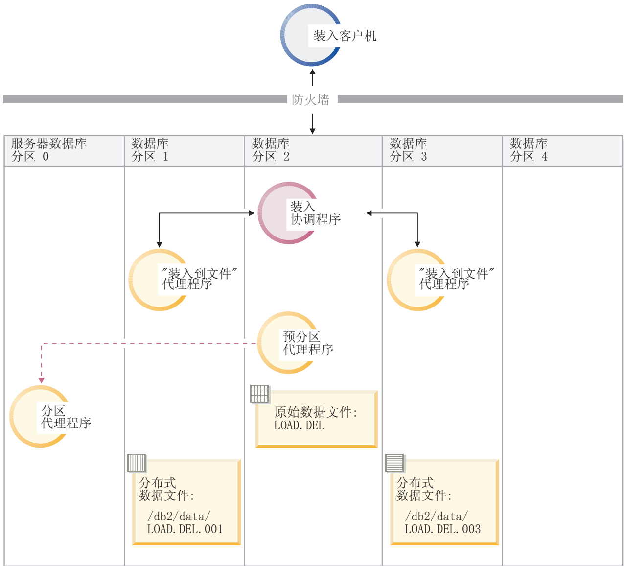
图 15. 使用一个分区代理程序将数据装入到数据库分区 1 和 3 中。此图说明发出以上命令后产生的行为。使用数据库分区 0 上运行的 1 个分区代理程序，将数据装入到数据库分区 1 和 3 中。
