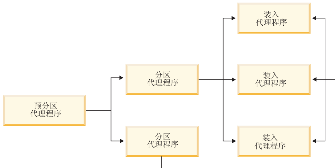
图 13. 分区数据库 load 概述. 预分区代理程序读取源数据，然后向两个分区代理程序中的每个分区代理程序各发送接近一半的数据，这两个分区代理程序分布数据并将该数据发送给三个数据库分区中的一个数据库分区。每个数据库分区上的装入代理程序装入数据。
