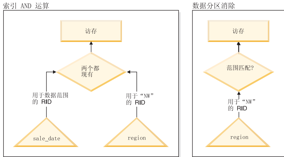
图 49. 用于进行表分区和索引“与”(AND) 操作的优化器决策路径
