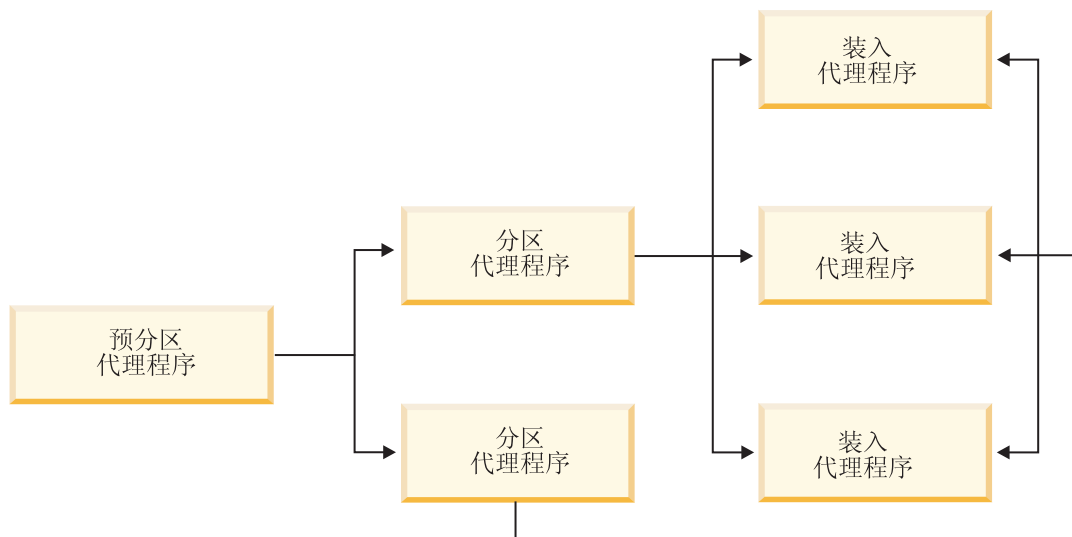
图 39. 分区数据库 load 概述. 预分区代理程序读取源数据，然后向两个分区代理程序中的每个分区代理程序各发送接近一半的数据，这两个分区代理程序分布数据并将该数据发送给三个数据库分区中的一个数据库分区。每个数据库分区上的装入代理程序装入数据。
