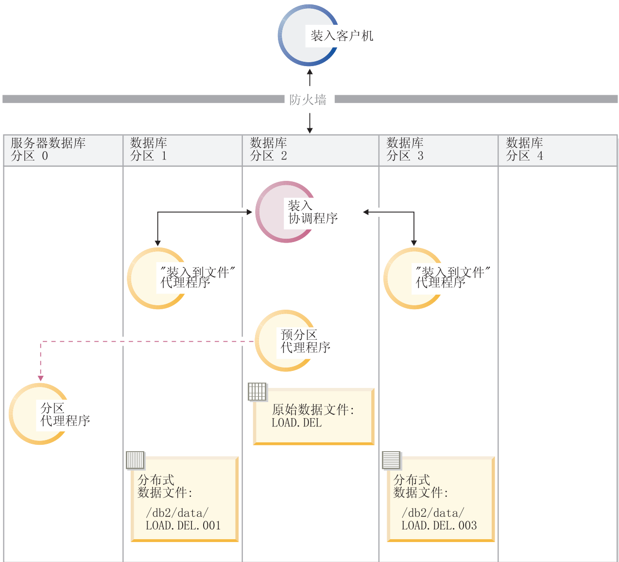
图 41. 使用一个分区代理程序将数据装入到数据库分区 1 和 3 中。此图说明发出以上命令后产生的行为。使用数据库分区 0 上运行的 1 个分区代理程序，将数据装入到数据库分区 1 和 3 中。
