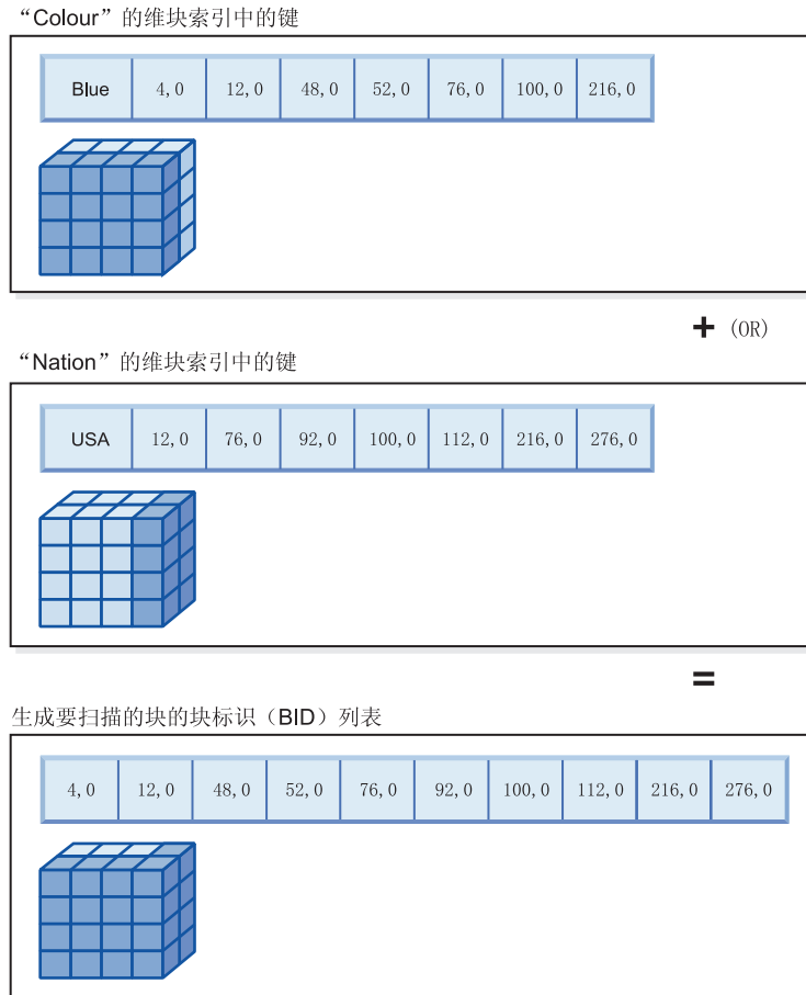
图 21. 可以如何对块索引使用逻辑 OR 运算
