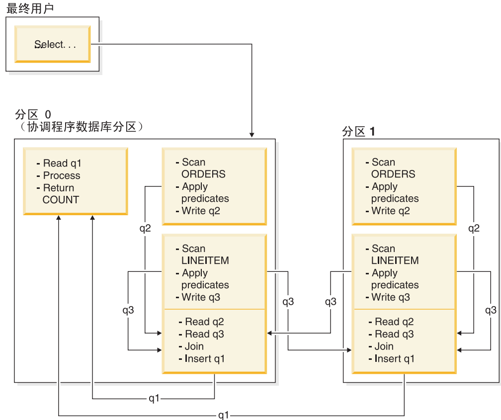
LINEITEM 表被发送到所有包含 ORDERS 表的数据库分区。表队列 q3 被广播至外表的所有数据库分区。 图 57. 广播内表连接示例
