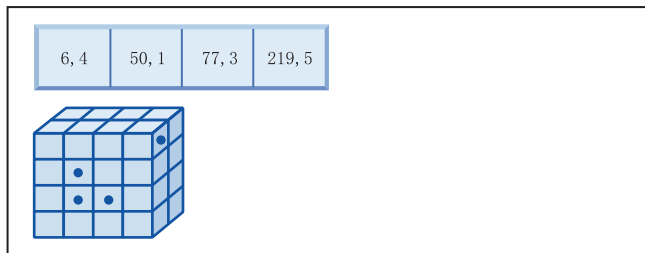
图 10. 对块索引和行标识 (RID) 索引使用逻辑 AND 运算的查询请求
