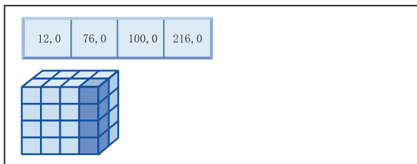
图 9. 对两个块索引使用逻辑 AND 运算的查询请求。
