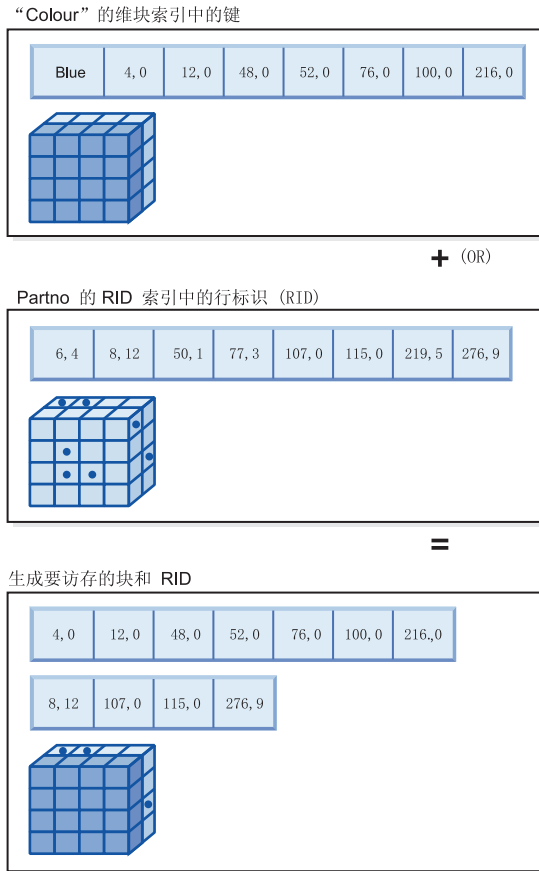
图 11. 使用逻辑 OR 运算的块索引和行标识的工作方式
