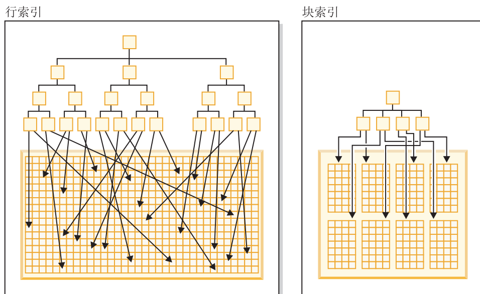
图 13. 行索引与块索引的区别
