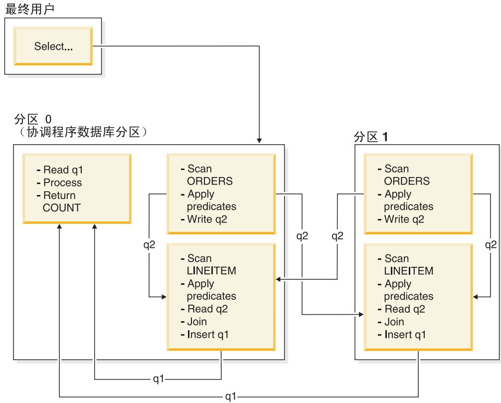
图 28. 广播外表连接示例
