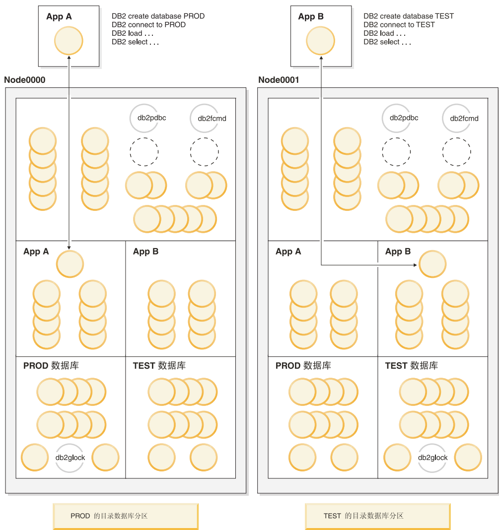
图 7. 多数据库分区的进程技术模型
