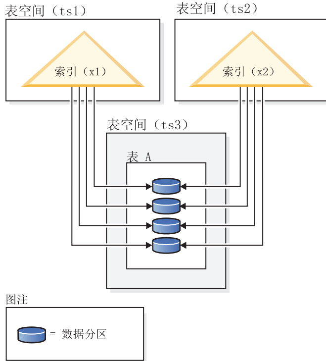
图 12. 分区表的非分区索引
