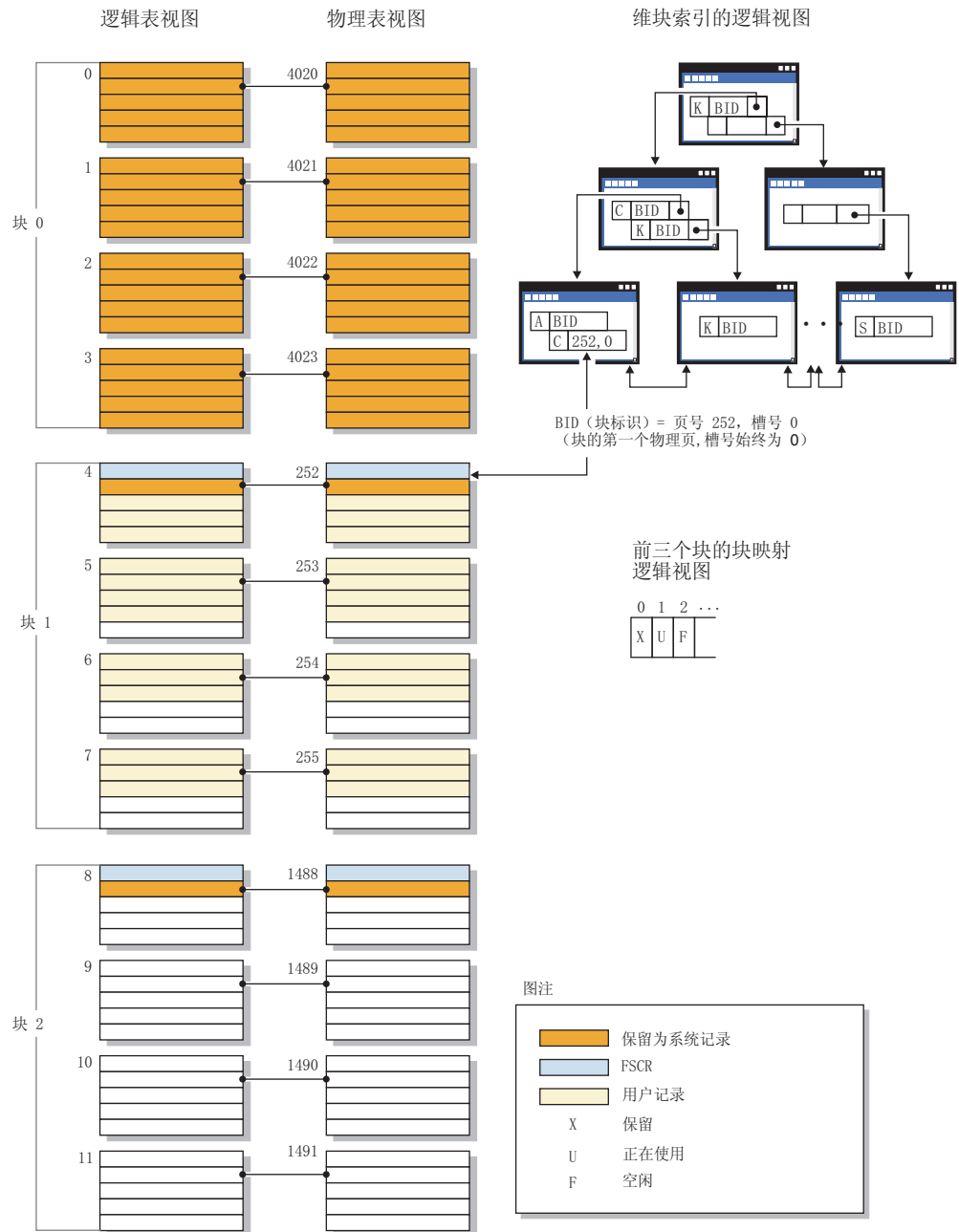
图 10. MDC 表的逻辑表、记录和索引结构
