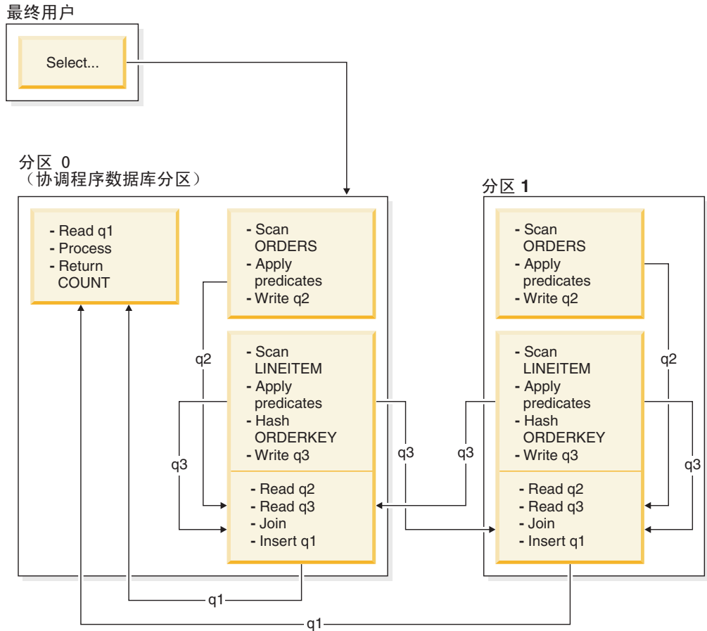
ORDERS 表根据 ORDERKEY 列进行分区。LINEITEM 表根据另一个列进行分区。LINEITEM 表将进行散列并被发送到 ORDERS 表的正确数据库分区。在此示例中，假定连接谓词为： orders.orderkey = lineitem.orderkey 。 图 32. 定向内表连接示例
