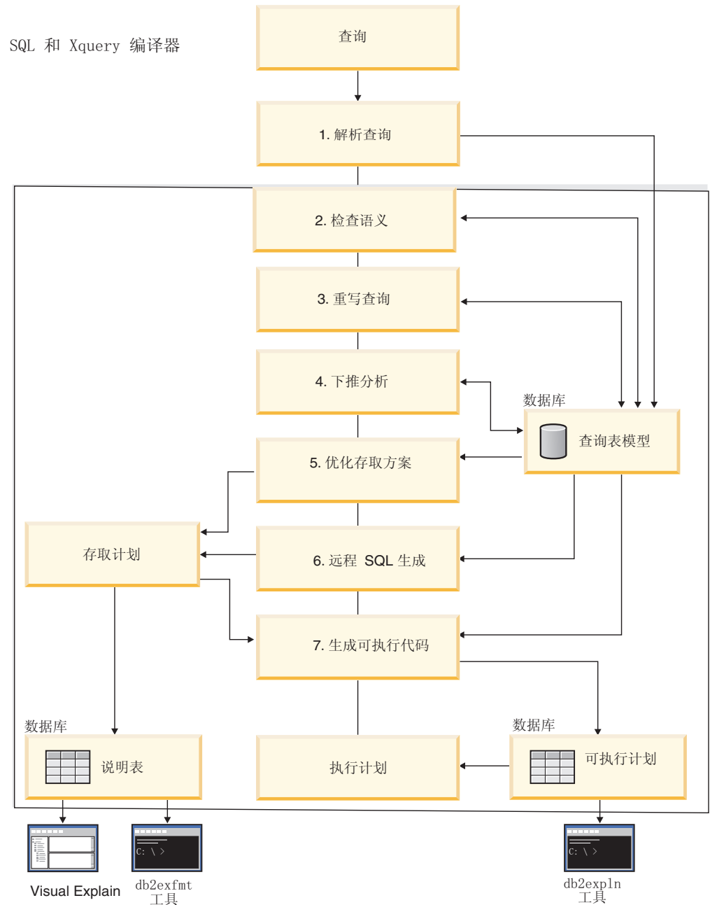
图 24. SQL 和 XQuery 编译器执行的步骤
