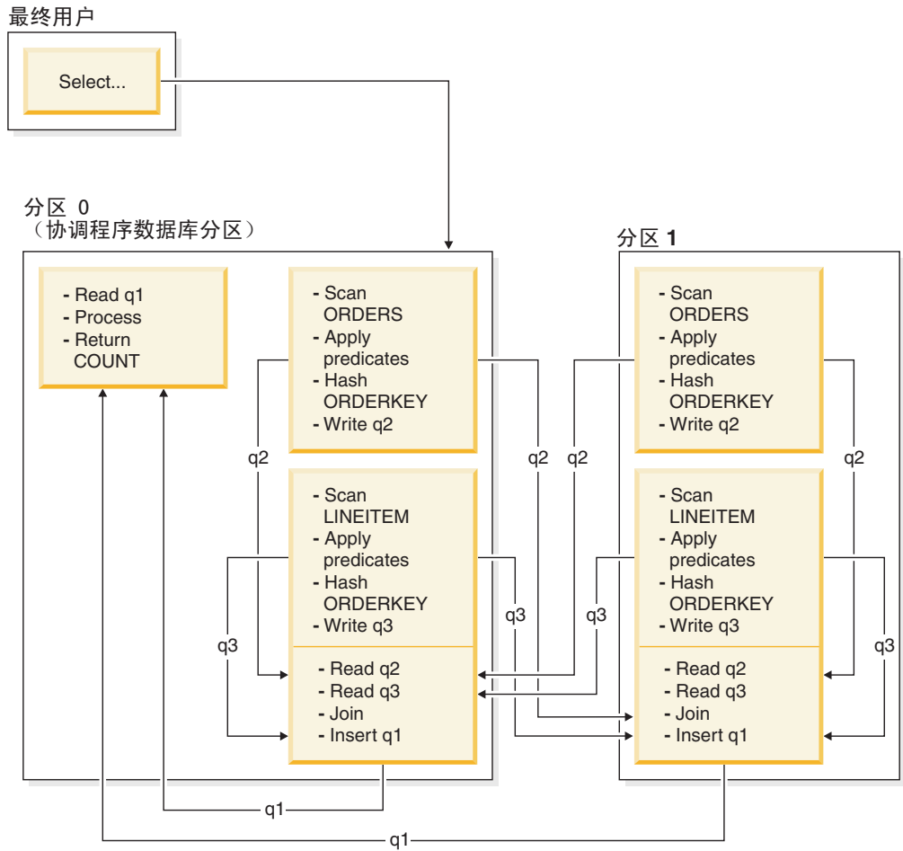
图 30. 定向内表和外表连接示例
