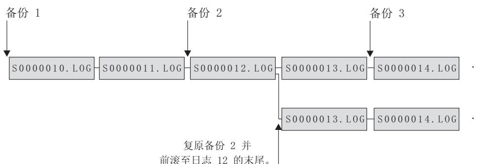
图 9. 复用日志文件名
