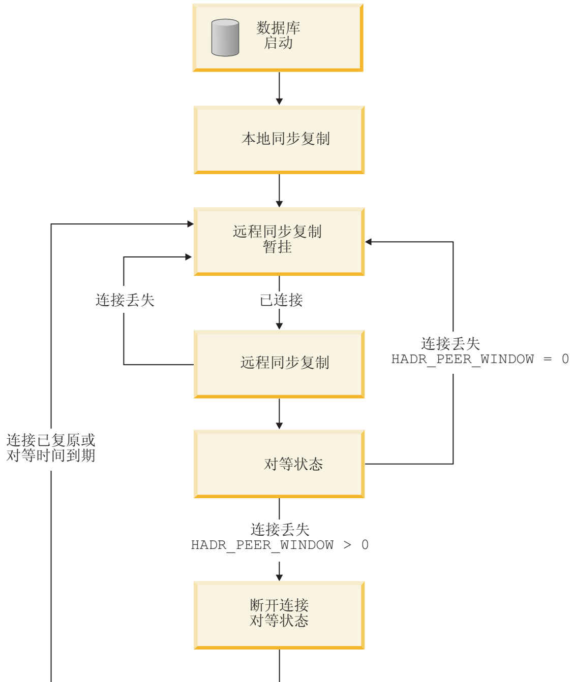
图 10. 备用数据库的状态
