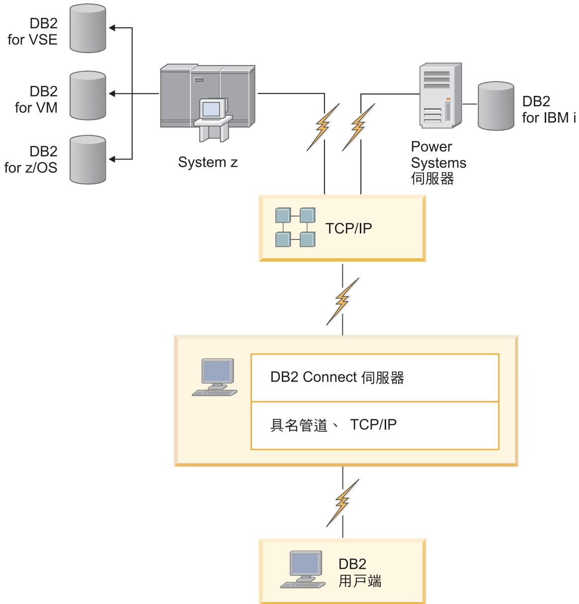
圖 2. 使用 DB2 Connect，將用戶端連接至 IBM 大型主機資料伺服器
