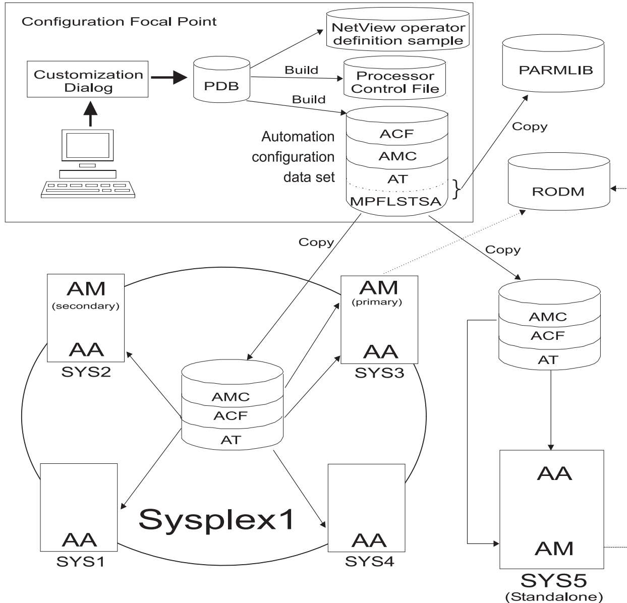
Figure 243. SA z/OS Automation Configuration
