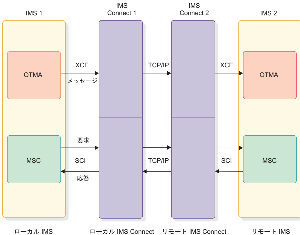
図 16. IMS 間 TCP/IP 接続の構成例
