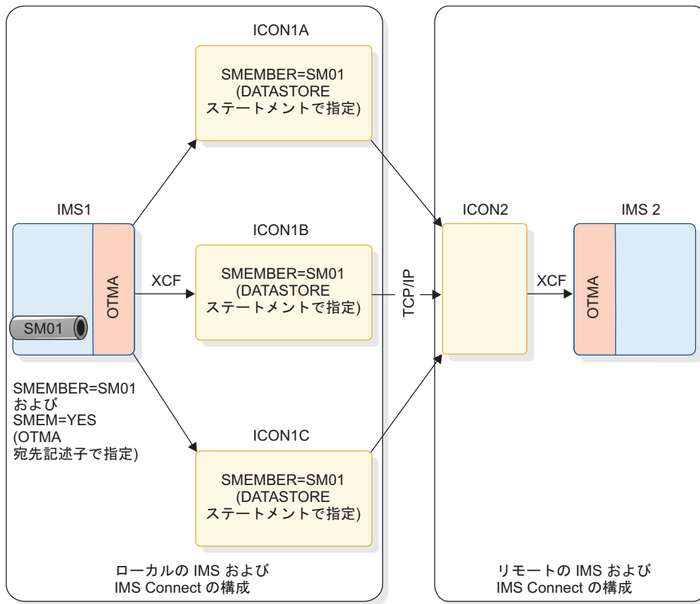
図 19. OTMA IMS 間 TCP/IP 接続でのスーパー・メンバー・グループの使用
