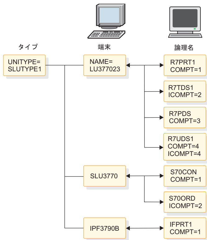
図 29. 2 次論理装置タイプ 1 VTAM 端末
