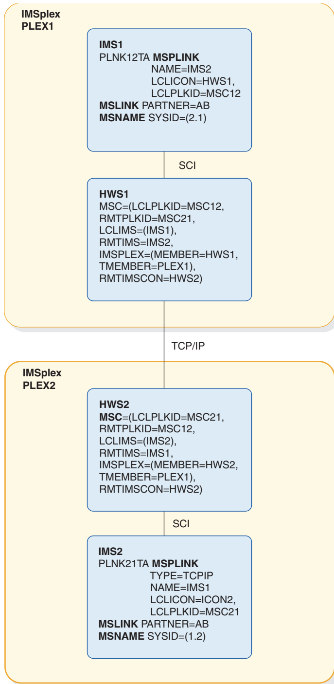
図 17. MSC TCP/IP リンク構成の例
