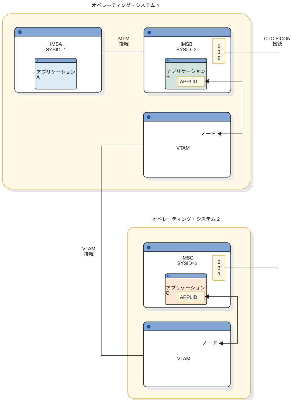
図 34. 複数システム結合機能の例
