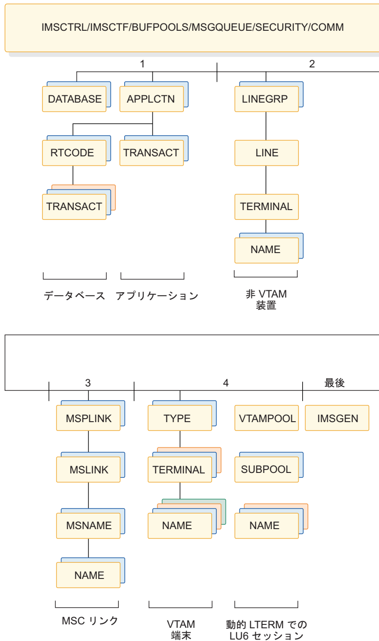
図 1. ステージ 1 のシステム定義マクロの階層
