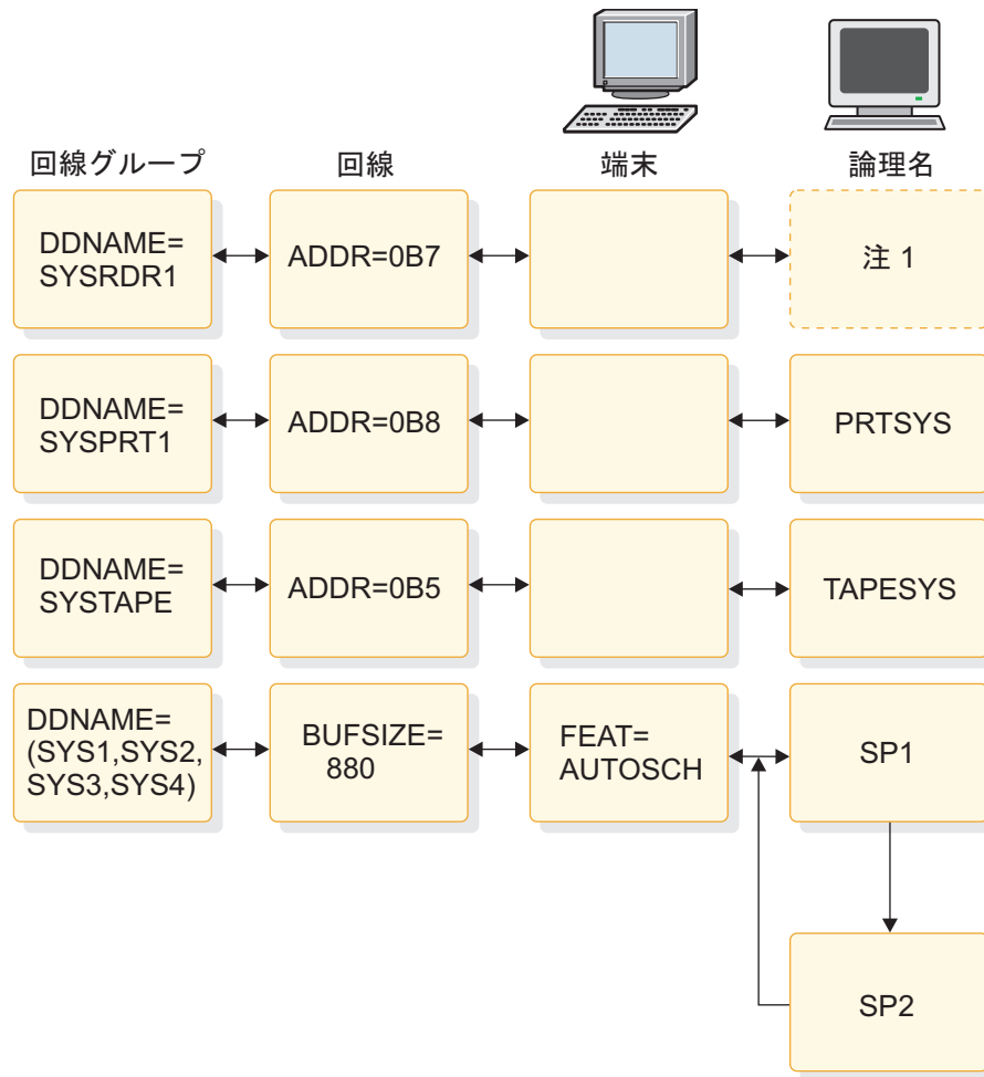
図 25. ローカル SYSOUT 回線グループ
