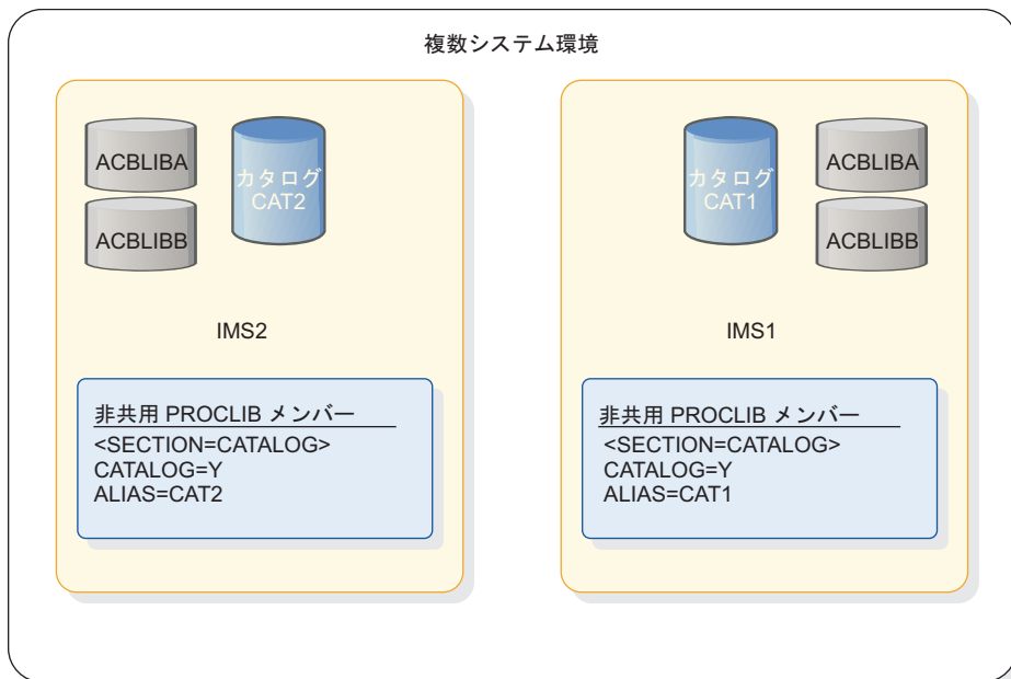
図 15. 複数システム環境で、独立したカタログ・データベースと独立した IMS.PROCLIB メンバーを使用する 2 つの IMS システム
