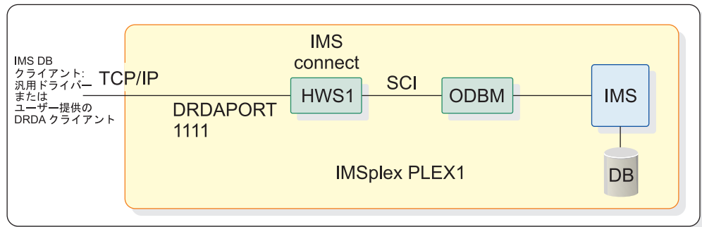
図 52. IMS DB サポート用の簡単な IMS Connect システム構成
