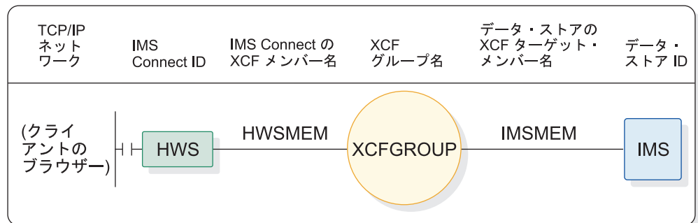
図 50. IMS TM サポート用の簡単な IMS Connect システム構成
