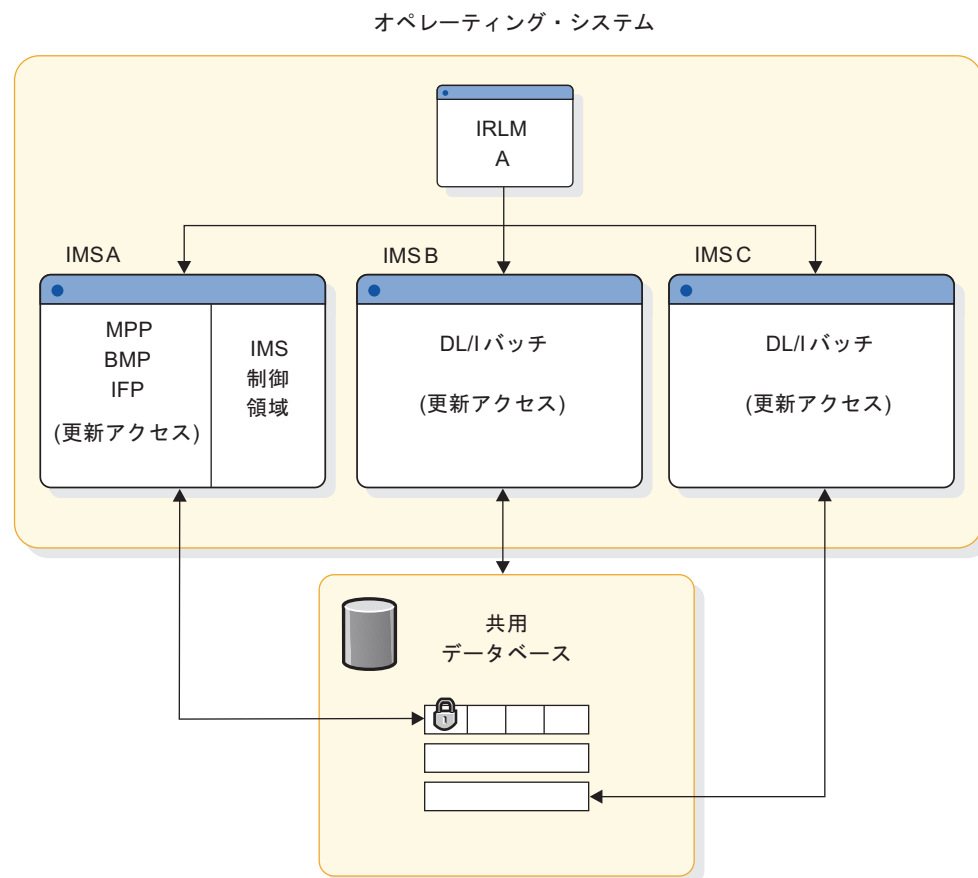
図 37. CPC 内ブロック・レベル・データ共有
