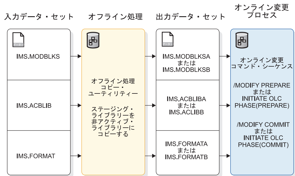
図 5. IMS リソースのオンライン変更プロセス
