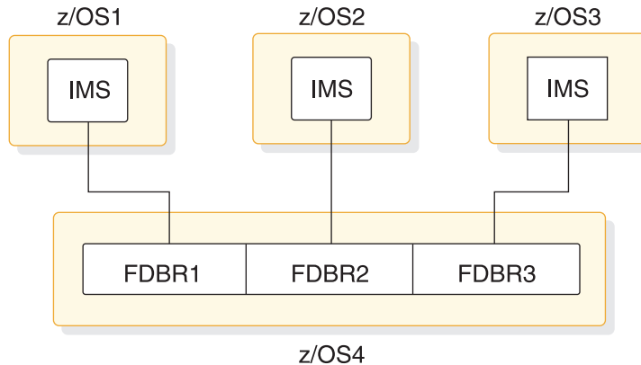
図 10. FDBR による 3 つの IMS サブシステムの追跡のシステム構成 2
