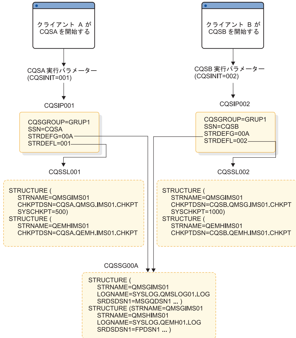
図 49. IMS および CQS パラメーターの指定
