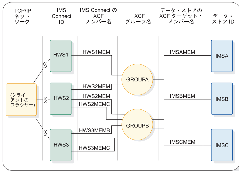
図 51. IMS TM サポート用の複雑な IMS Connect システム構成
