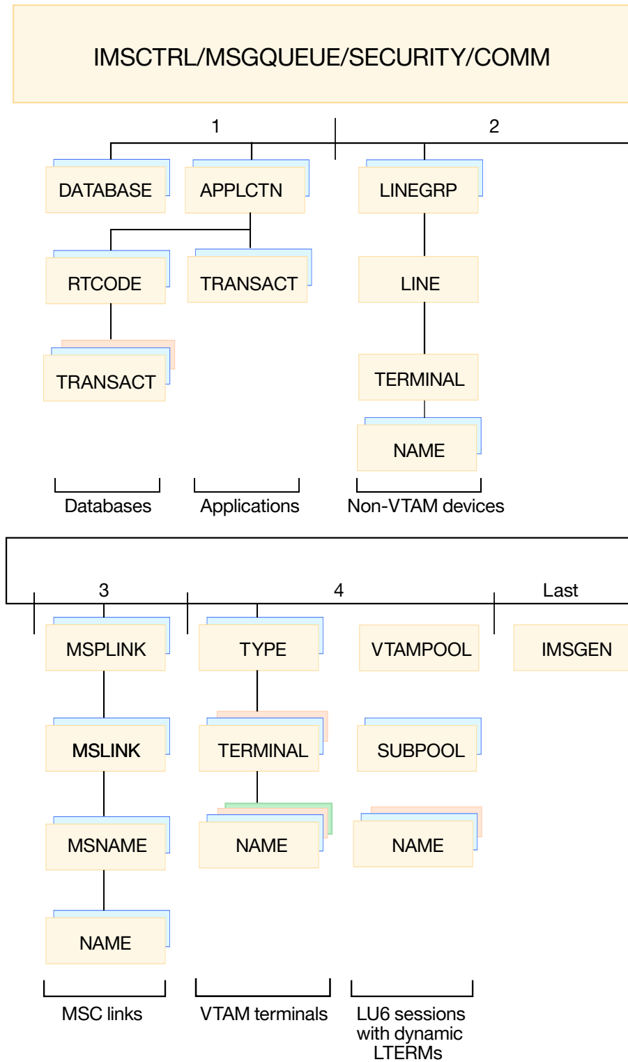
図 1. ステージ 1 のシステム定義マクロの階層
