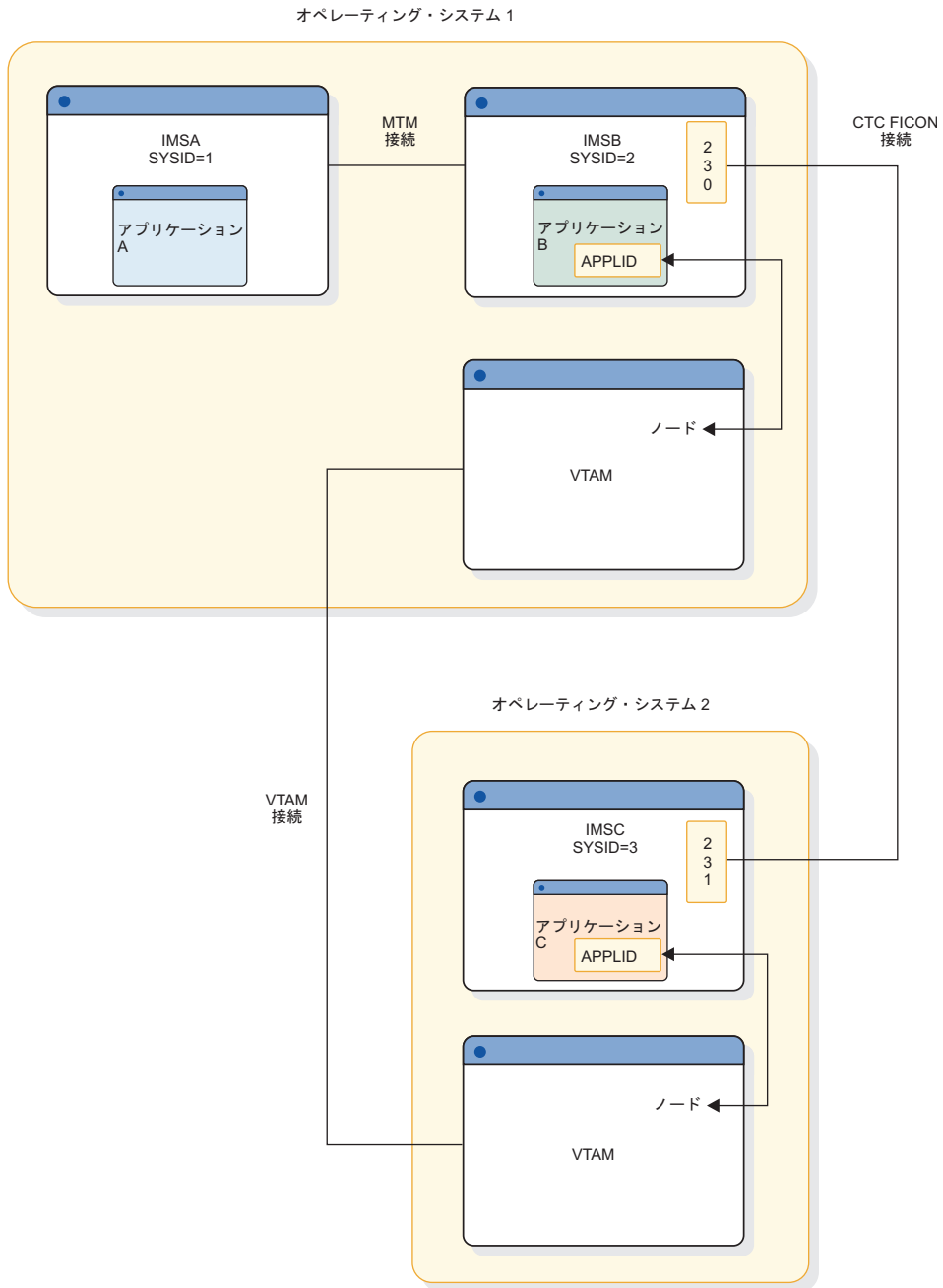
図 38. 複数システム結合機能の例
