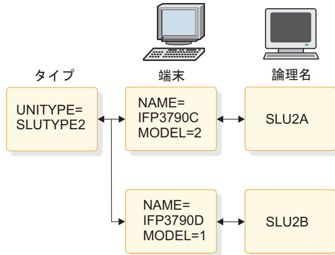
図 35. 2 次論理装置タイプ 2 VTAM 端末
