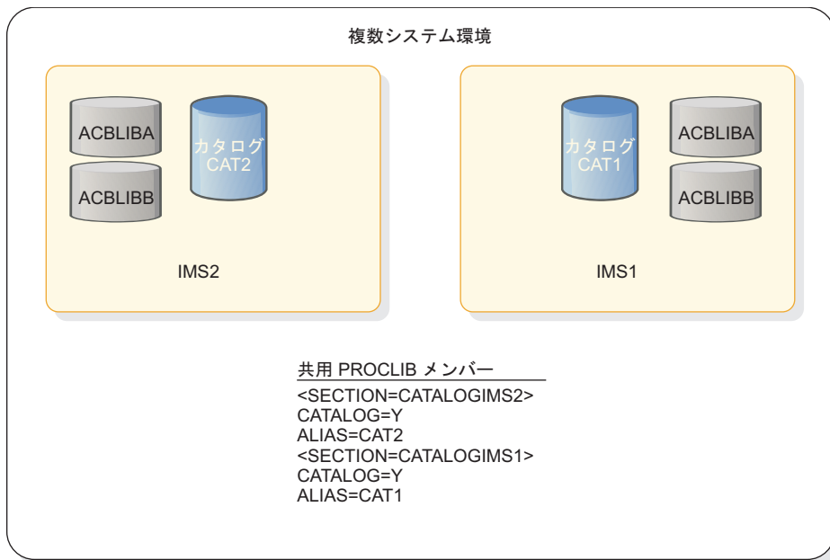
図 16. 複数システム環境で独立したカタログ・データベースを使用する 2 つの IMS システム
