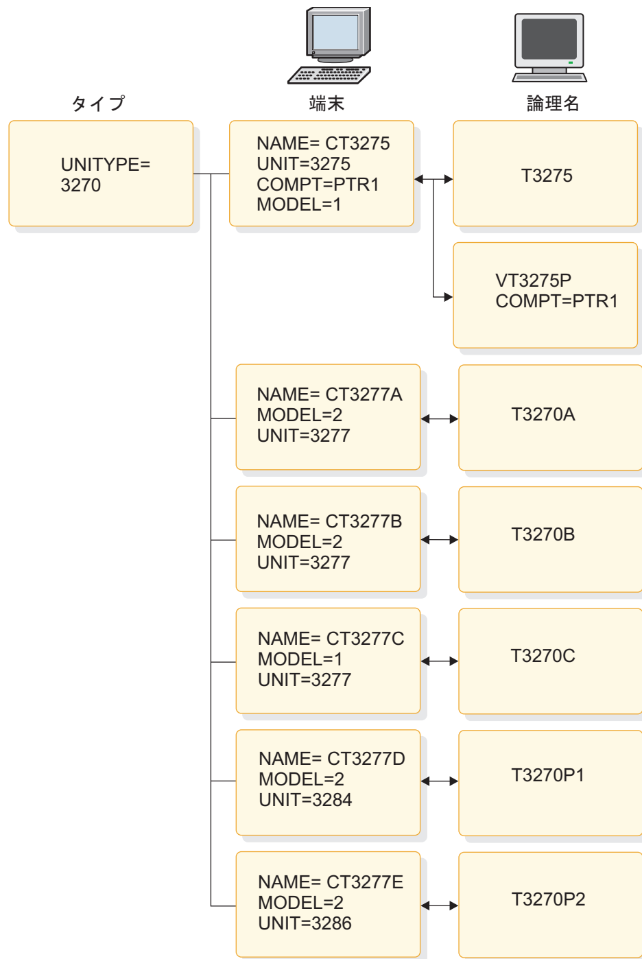
図 8. 3270 VTAM 端末の構成
