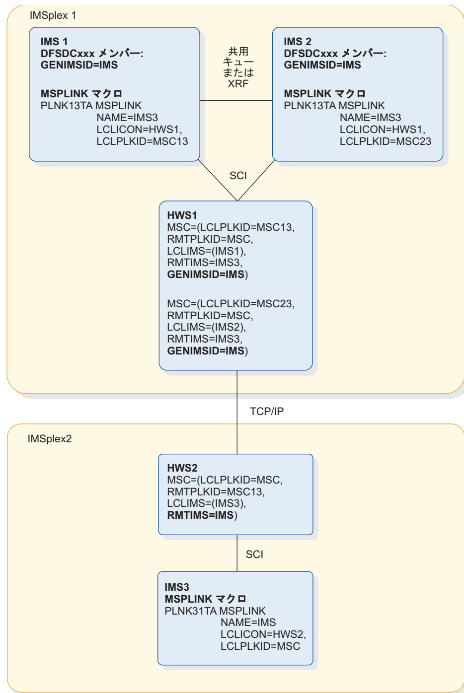
図 22. MSC TCP/IP 汎用リソース・グループのシステム定義ステートメントの例
