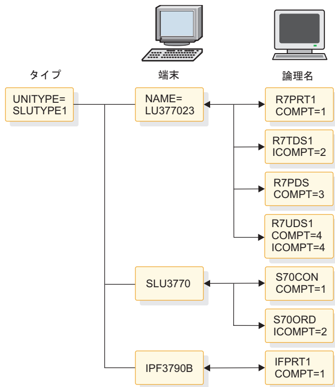
図 33. 2 次論理装置タイプ 1 VTAM 端末
