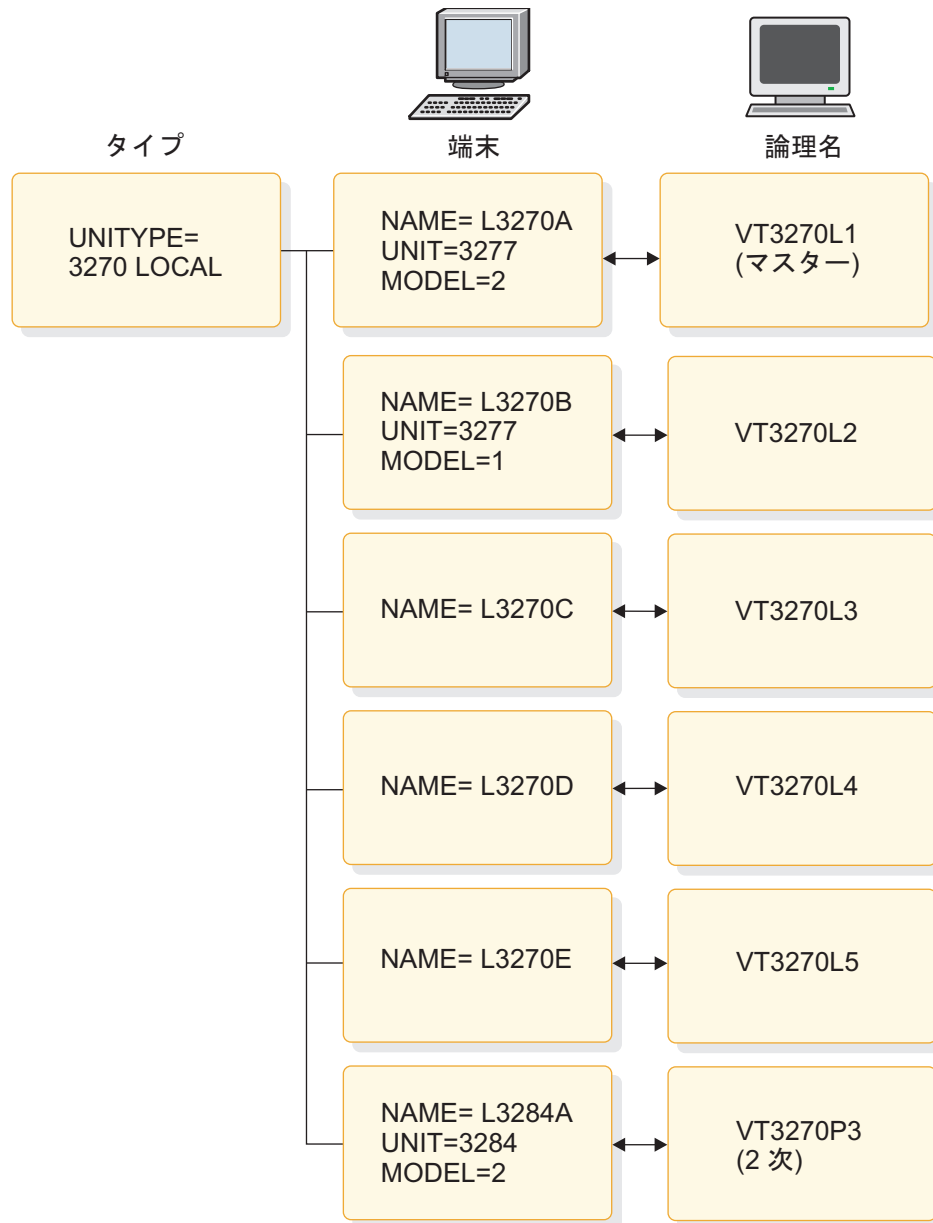
図 9. マスター端末の構成
