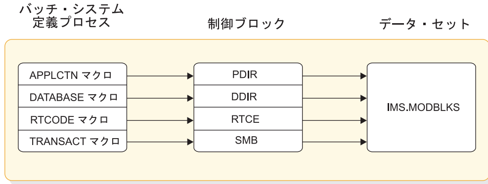
図 4. MODBLKS リソースの制御ブロック生成プロセス
