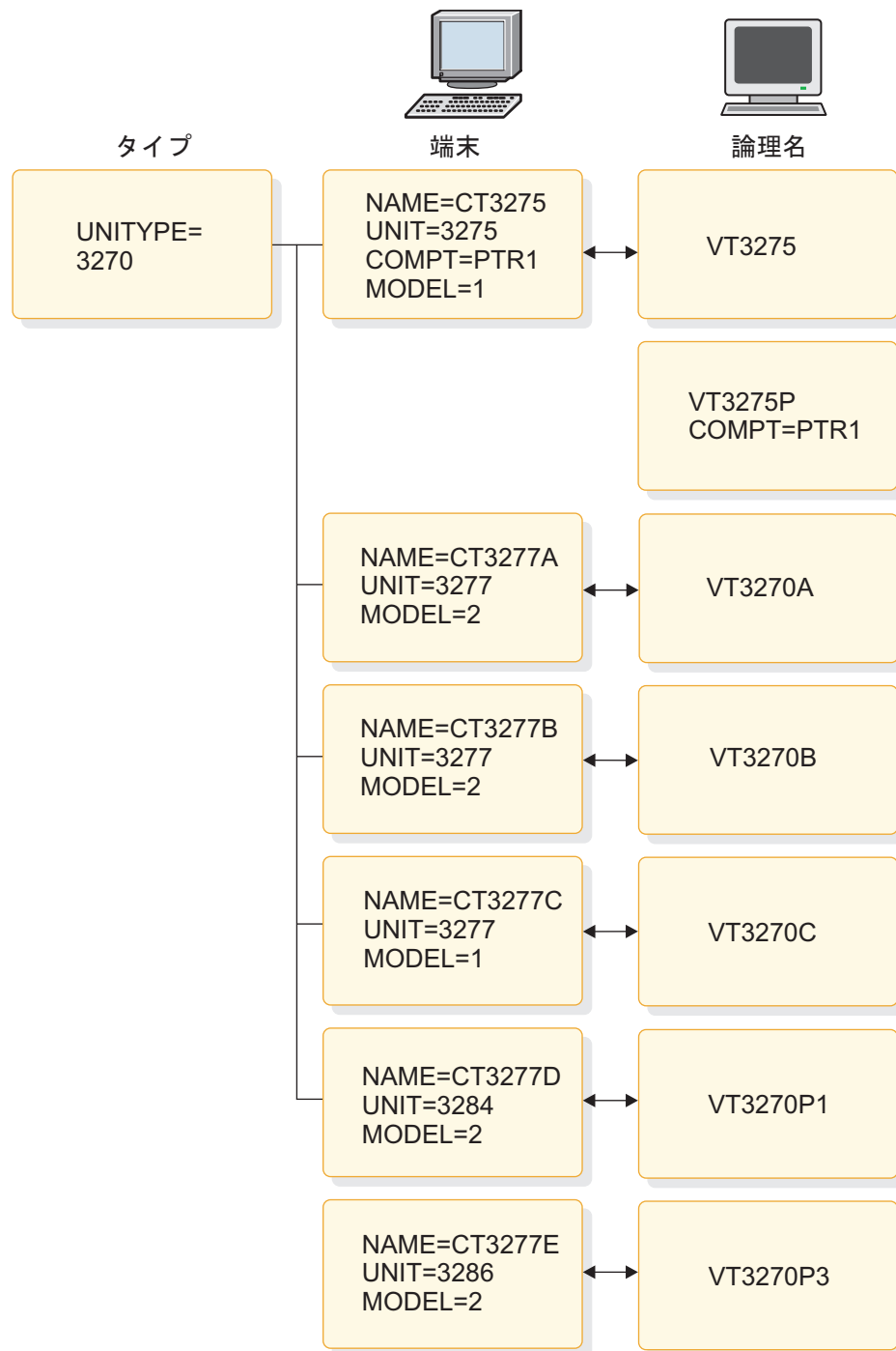
図 31. リモート 3270 VTAM 端末
