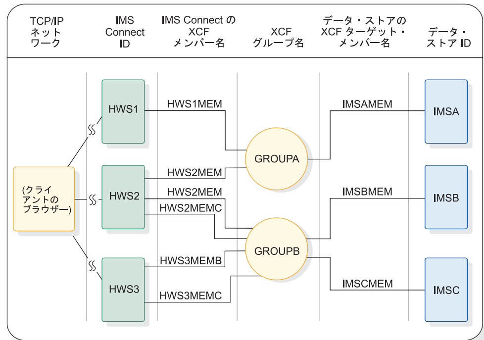
図 55. IMS TM サポート用の複雑な IMS Connect システム構成
