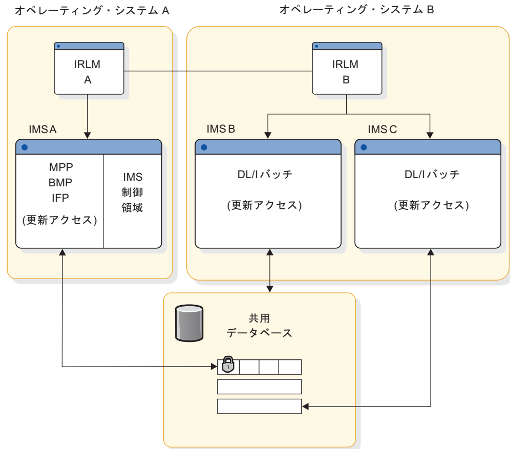
図 42. CPC 間ブロック・レベル・データ共有
