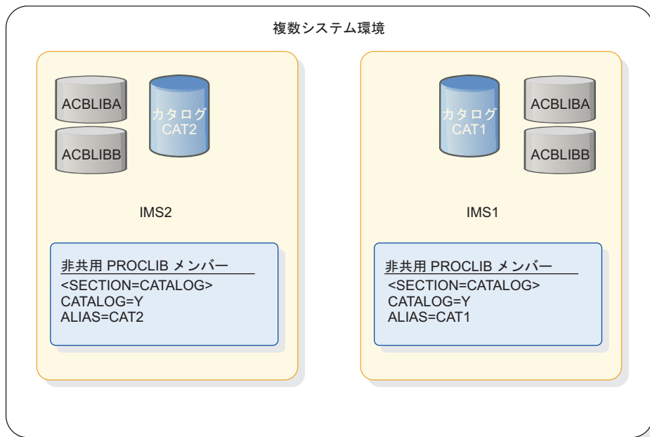
図 17. 複数システム環境で、独立したカタログ・データベースと独立した IMS.PROCLIB メンバーを使用する 2 つの IMS システム
