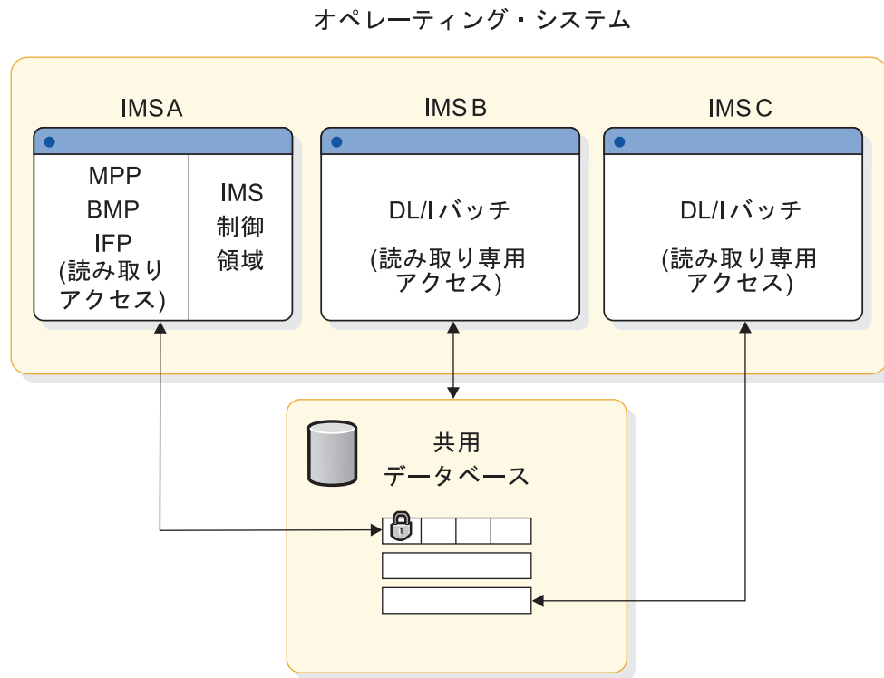
図 40. 読み取りアクセスを伴う、データベース・レベルのデータ共有
