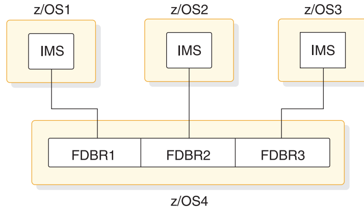
図 11. FDBR による 3 つの IMS サブシステムの追跡のシステム構成 2
