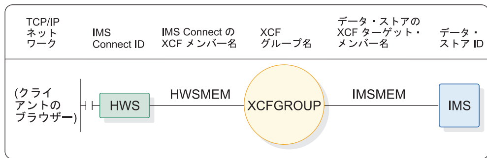
図 54. IMS TM サポート用の簡単な IMS Connect システム構成
