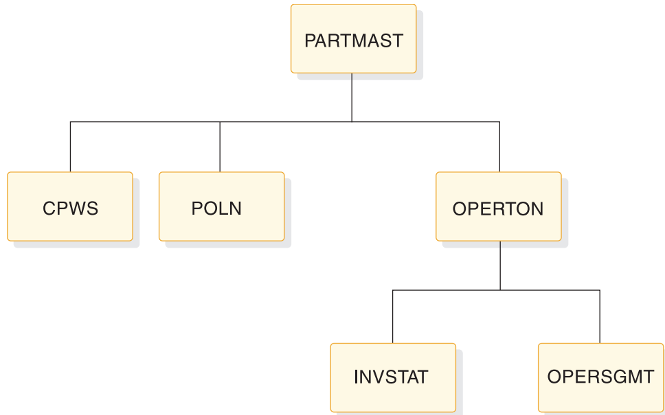
図 15. 階層データ構造の例
