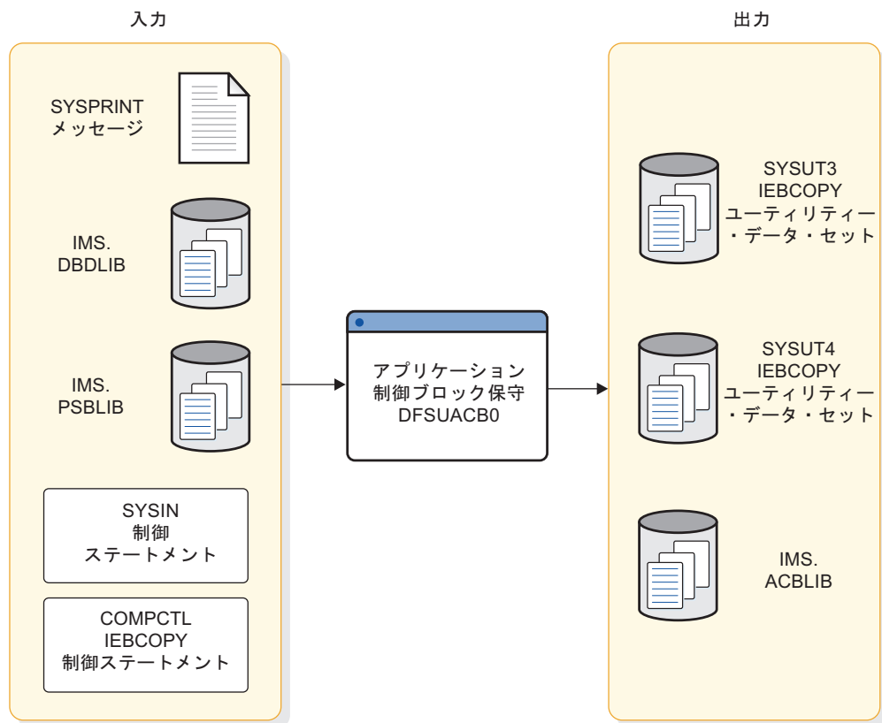
図 1. ACB 保守ユーティリティの入力と出力
