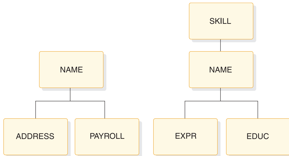
図 6. 給与計算インベントリーおよびスキル・インベントリーのデータ構造
