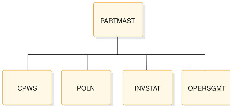
図 19. DL/I データベースの PCB ステートメントを定義する際に使用される PSBGEN PCB ステートメント (例 3)
