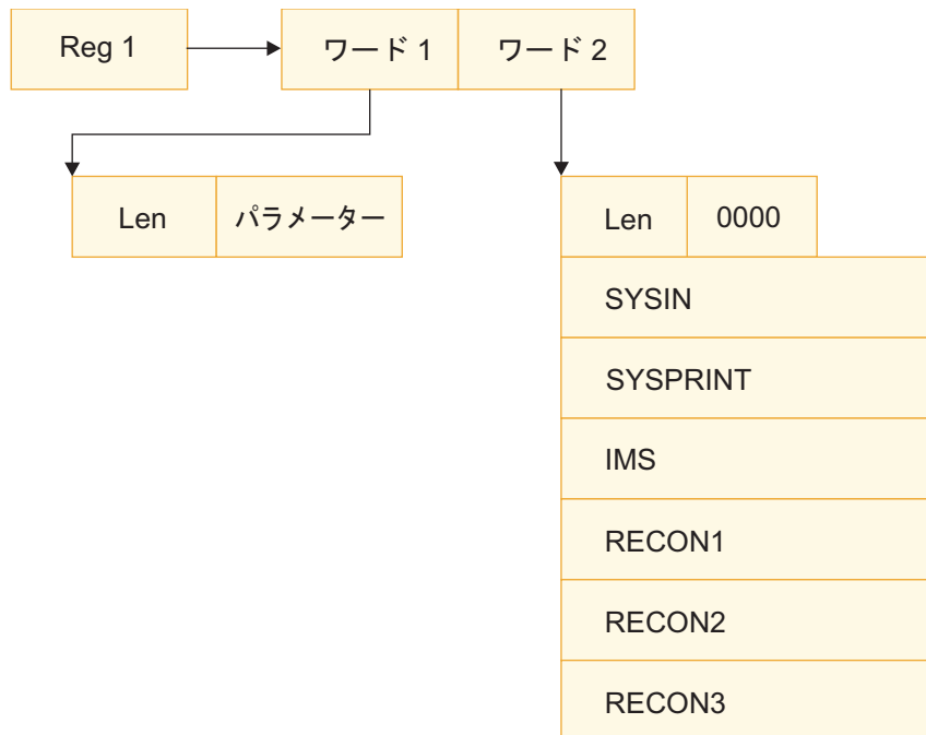
図 40. データベース・リカバリー管理ユーティリティを呼び出すために必要なレジスターとオペランド・リストの内容
