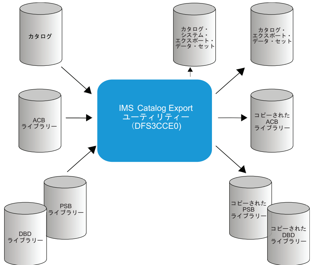
図 33. エクスポートでの IMS Catalog Export ユーティリティの入力と出力
