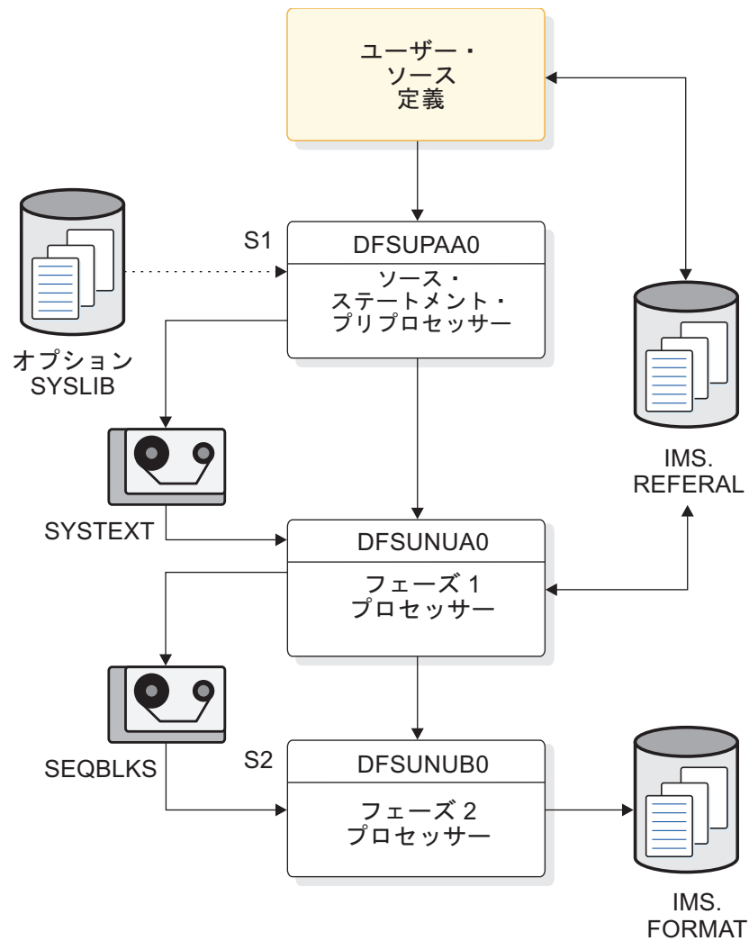
図 10. MFSUTL プロシージャラーの全体のフロー
