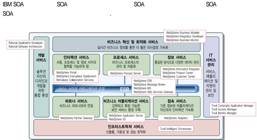
6_ IBM SOA
