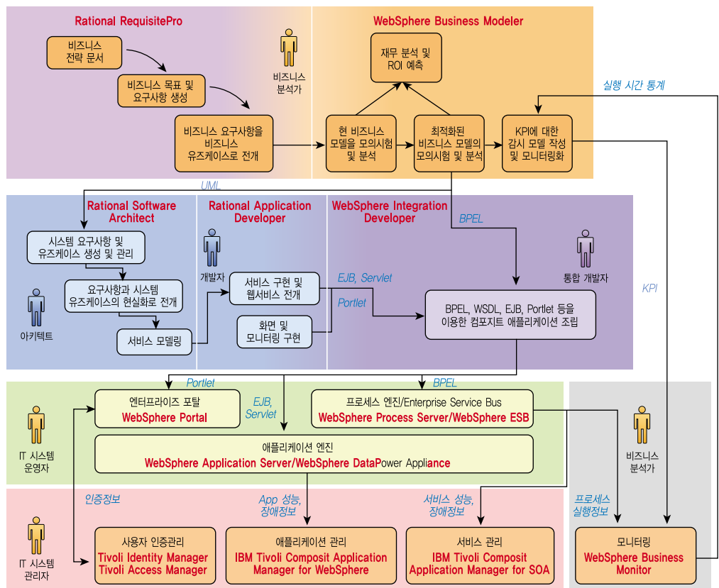
8 IBM SOA
