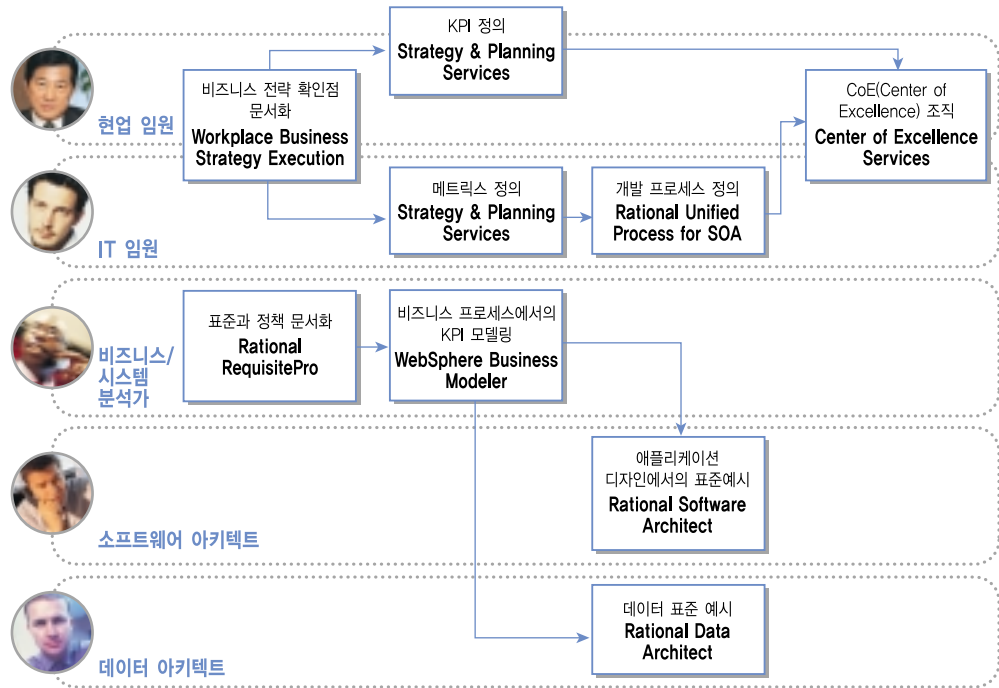
12_SOA
