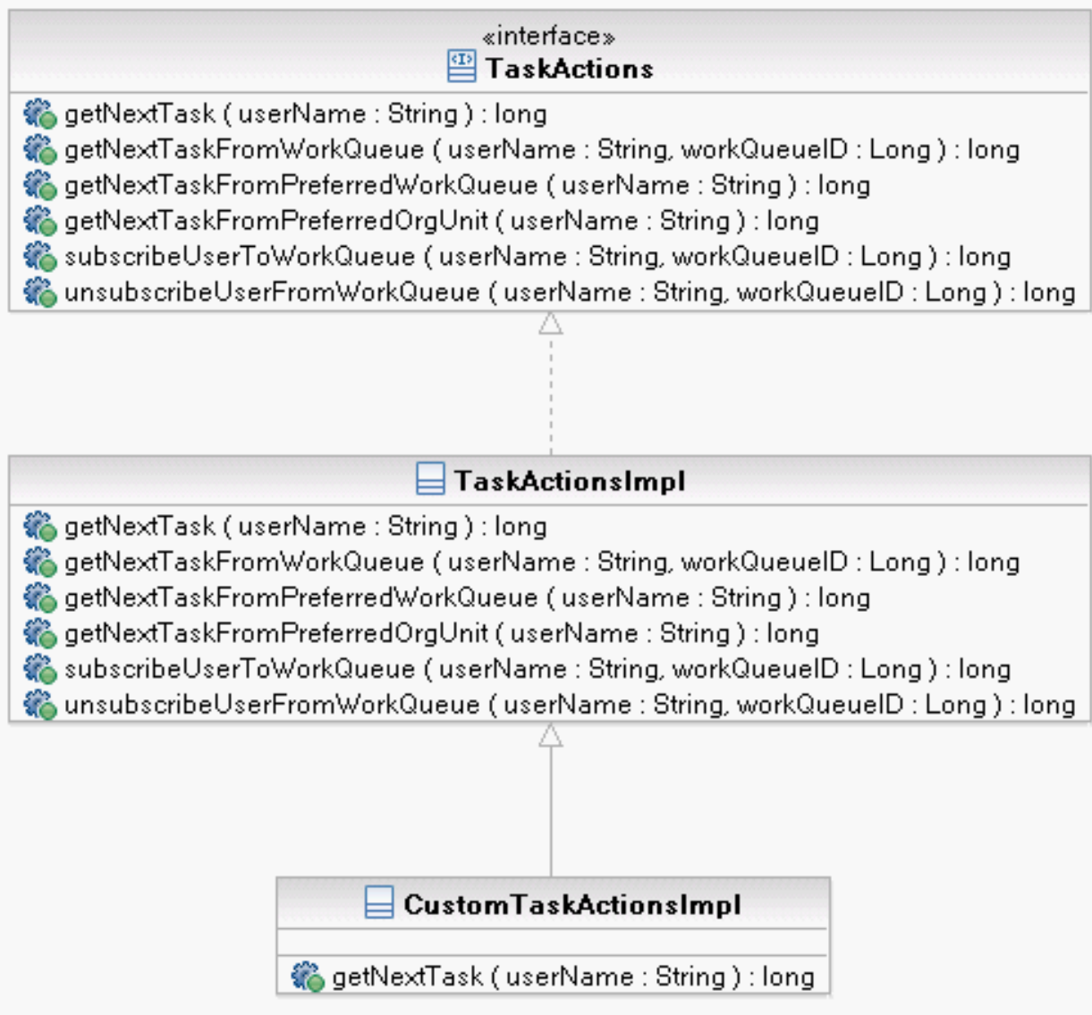
Abbildung 5. Anpassungsklassendiagramm
