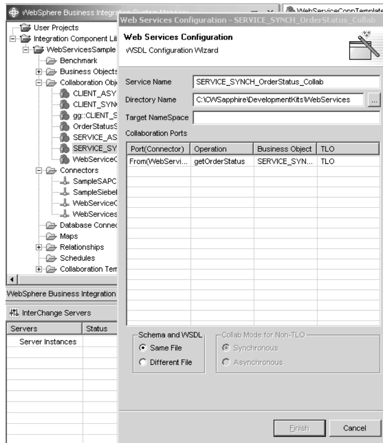
図 57. WSDL 構成ウィザード
