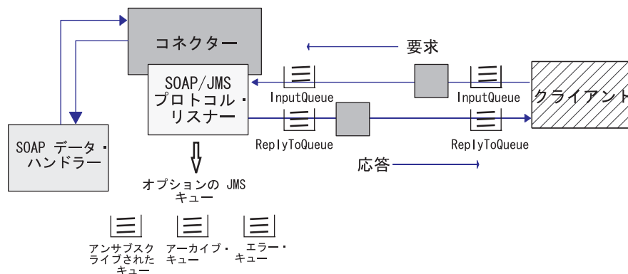
図 26. SOAP/JMS プロトコル・リスナー: 同期イベント処理
