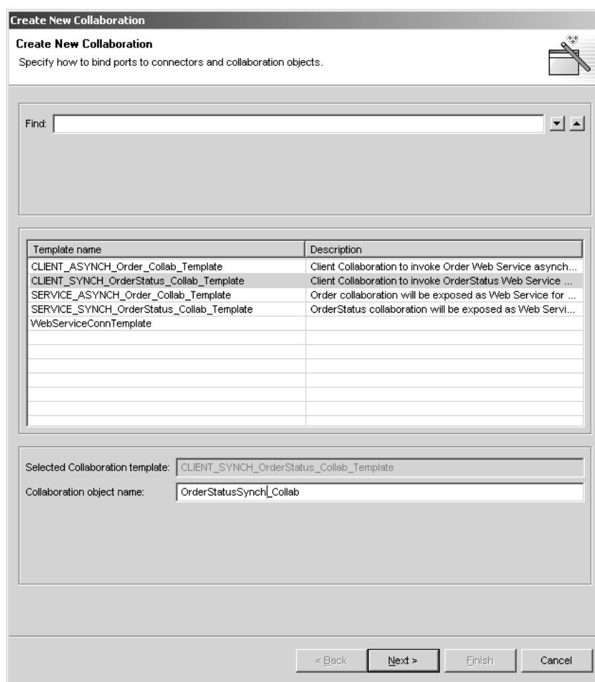
図 54. 「新規コラボレーションの作成 (Create New Collaboration)」ウィンドウ
