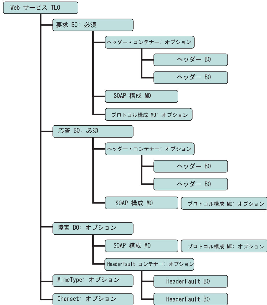
図4. 同期イベント処理のためのビジネス・オブジェクト階層
