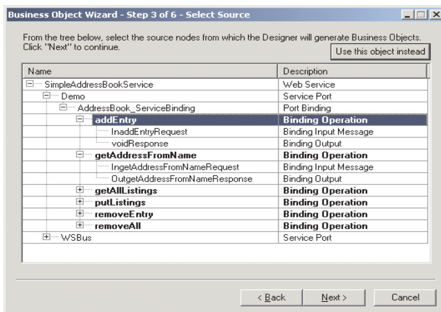
図 64. 「ソースの選択」ウィンドウ
