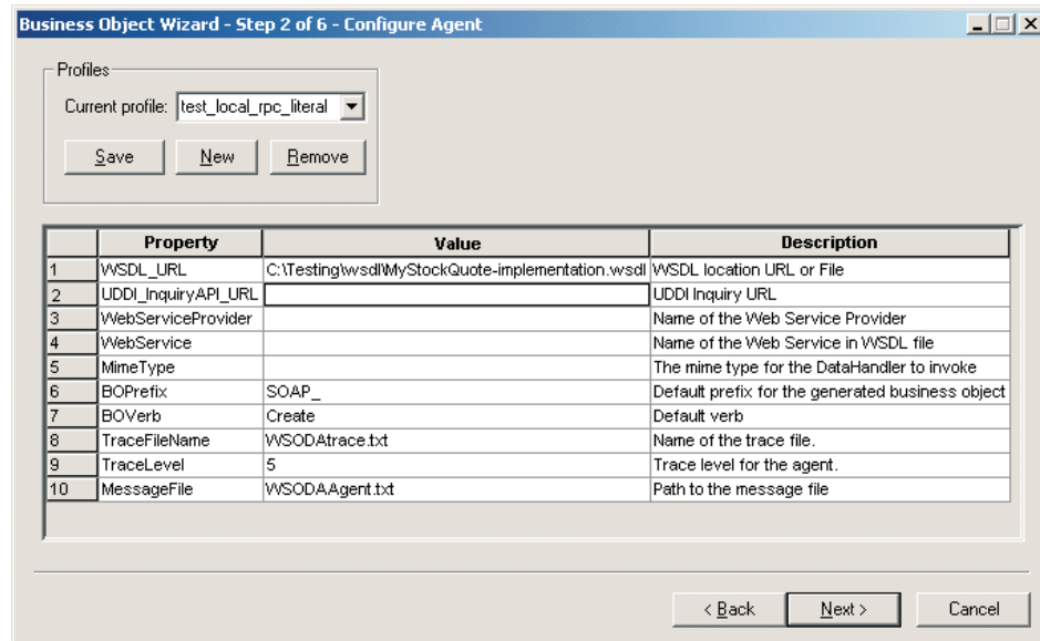
図 63. 「エージェントの構成」ウィンドウ
