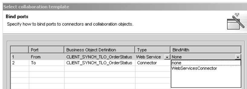
図 56. Web サービス・コネクターのインスタンスの選択
