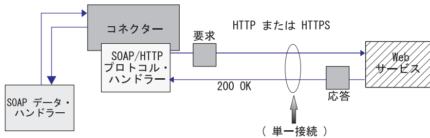
図 28. SOAP/HTTP-HTTPS プロトコル・ハンドラー: 同期要求処理
