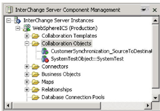
图 30. “InterChange Server 组件管理”视图中的“协作对象”文件夹
