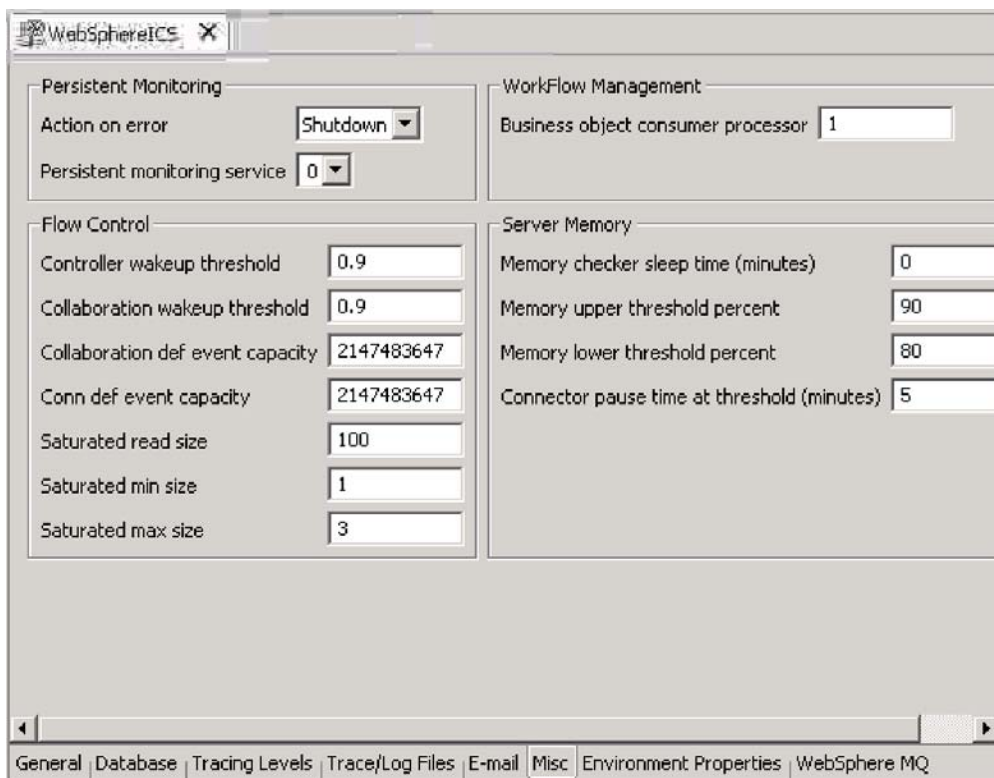
图 16. “编辑配置”工具，“其它”选项卡
