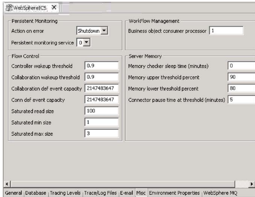
图 24. 编辑配置工具，“其它”选项卡
