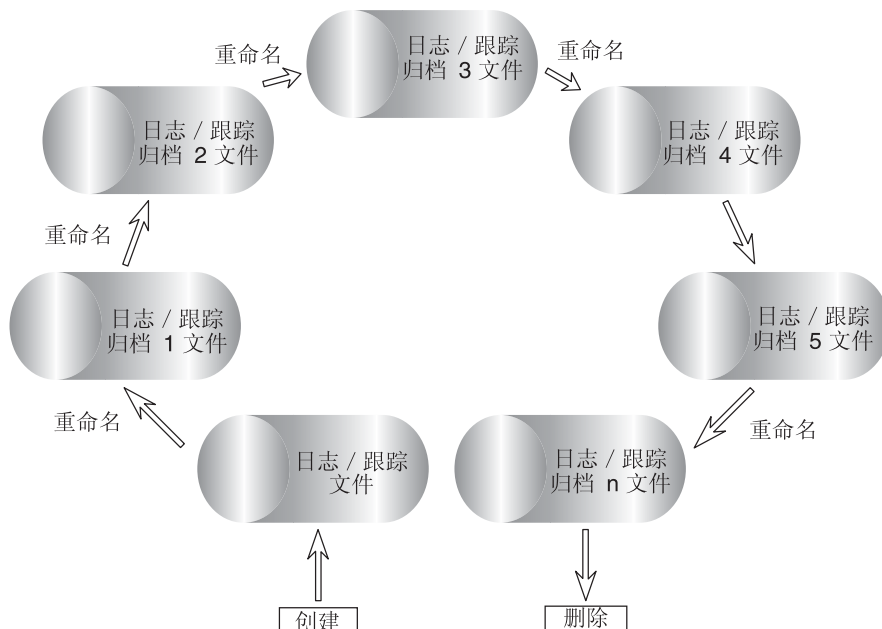
图 48. 循环归档记录
