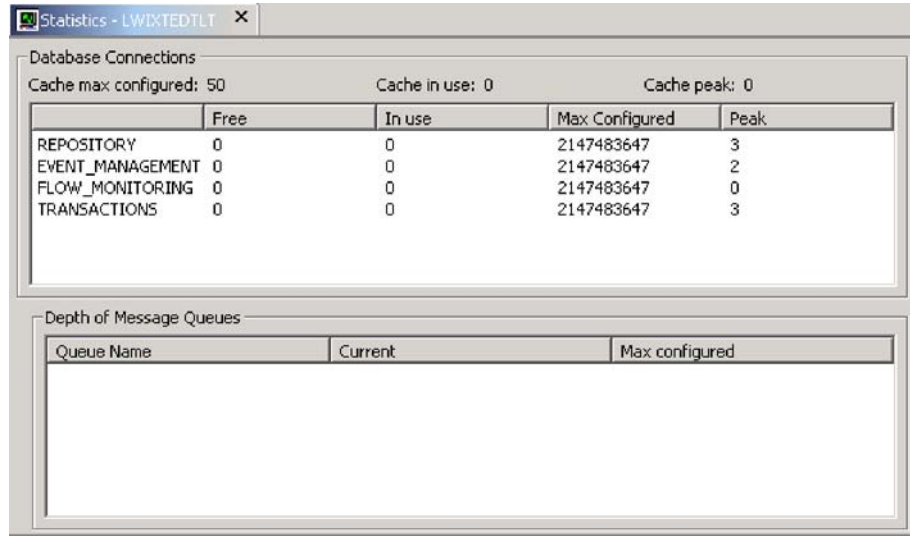
图 19. InterChange Server Express 的统计信息窗口
