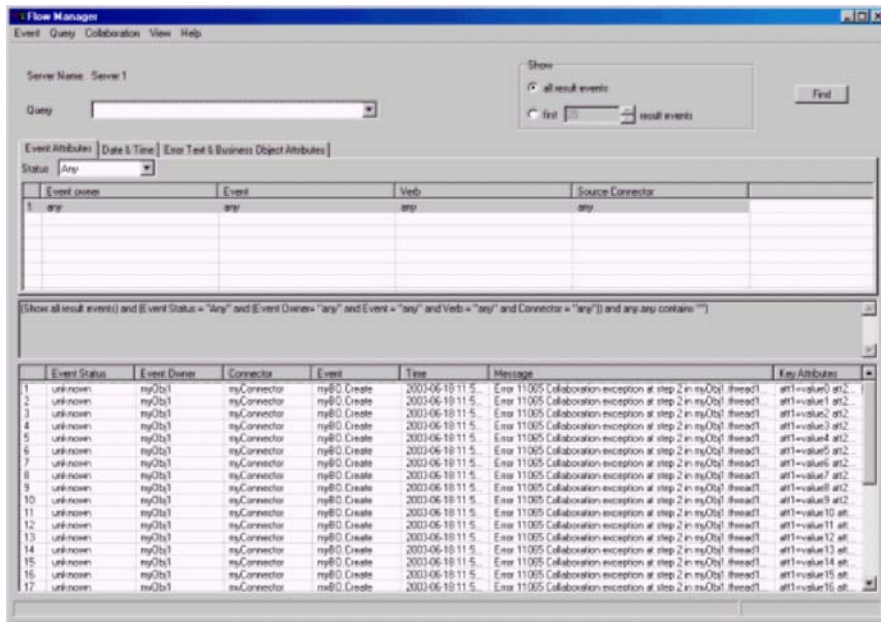
图 71. 显示过滤结果的流管理器
