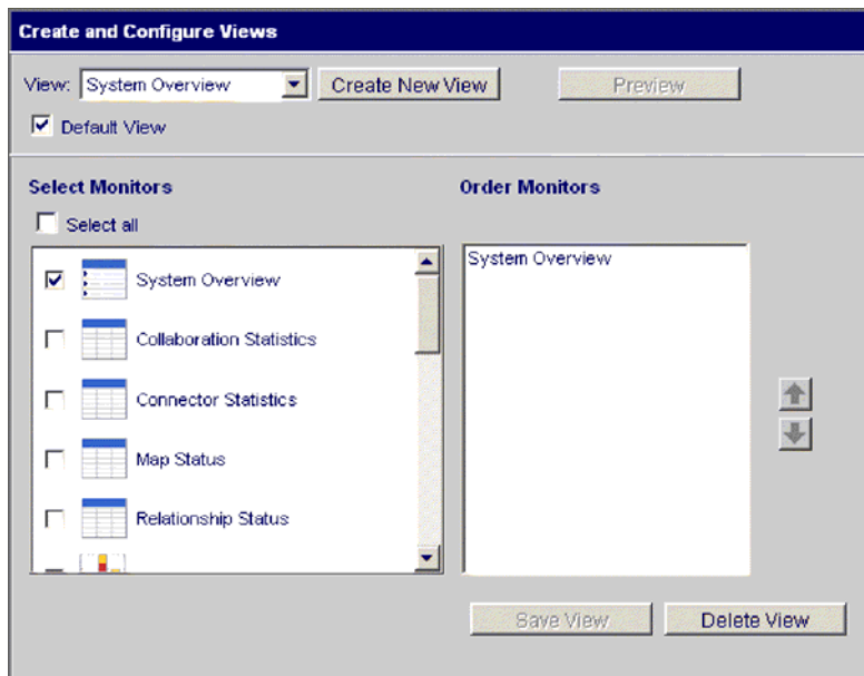
图 12. 系统监视器，“创建和配置视图”对话框
