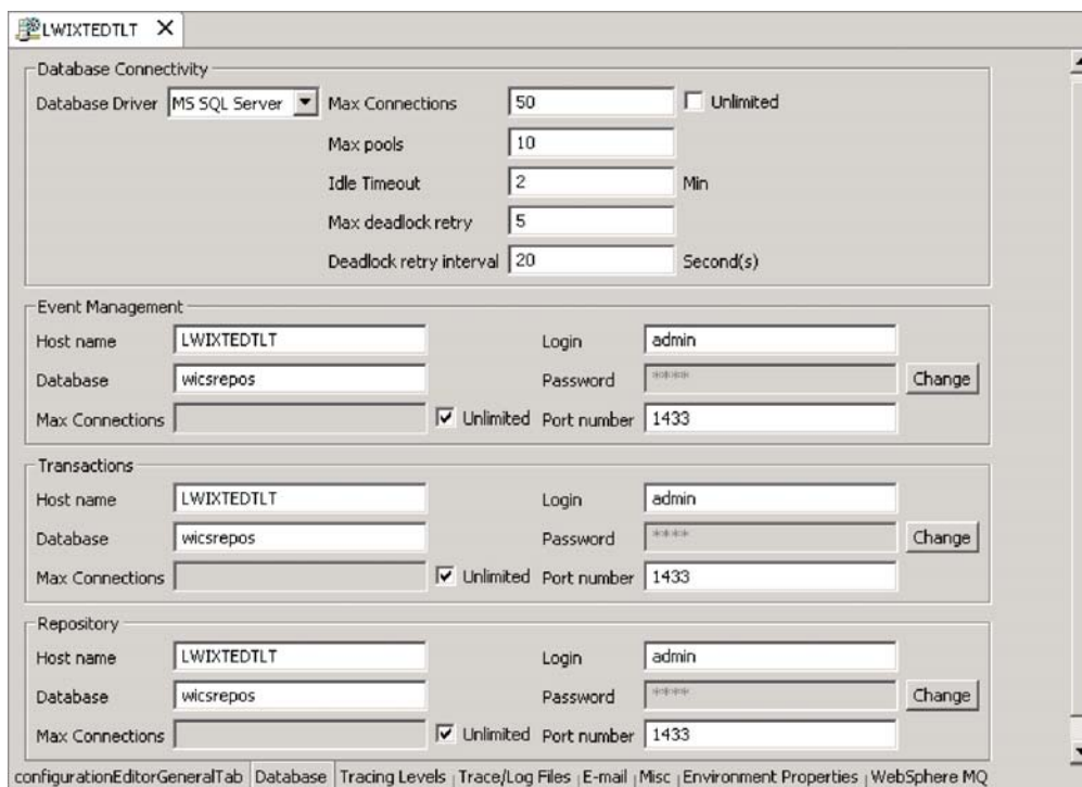
图 22. “编辑配置”窗口的“数据库”选项卡
