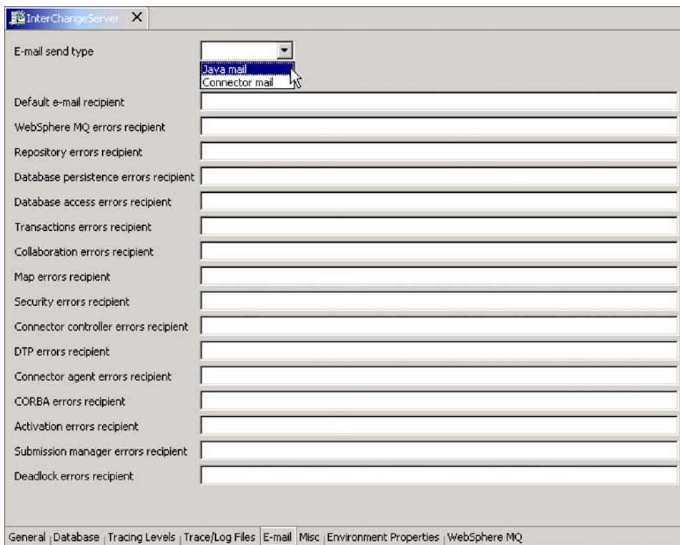
图 49. 编辑配置，“电子邮件”选项卡
