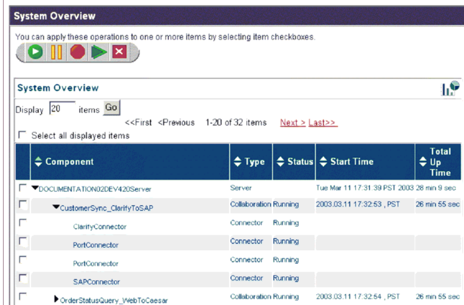
图 29. 系统监视器，显示协作对象状态的“系统概述”
