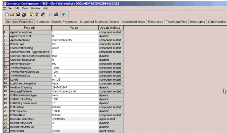
图 28. 连接器配置器易捷版，“标准属性”选项卡
