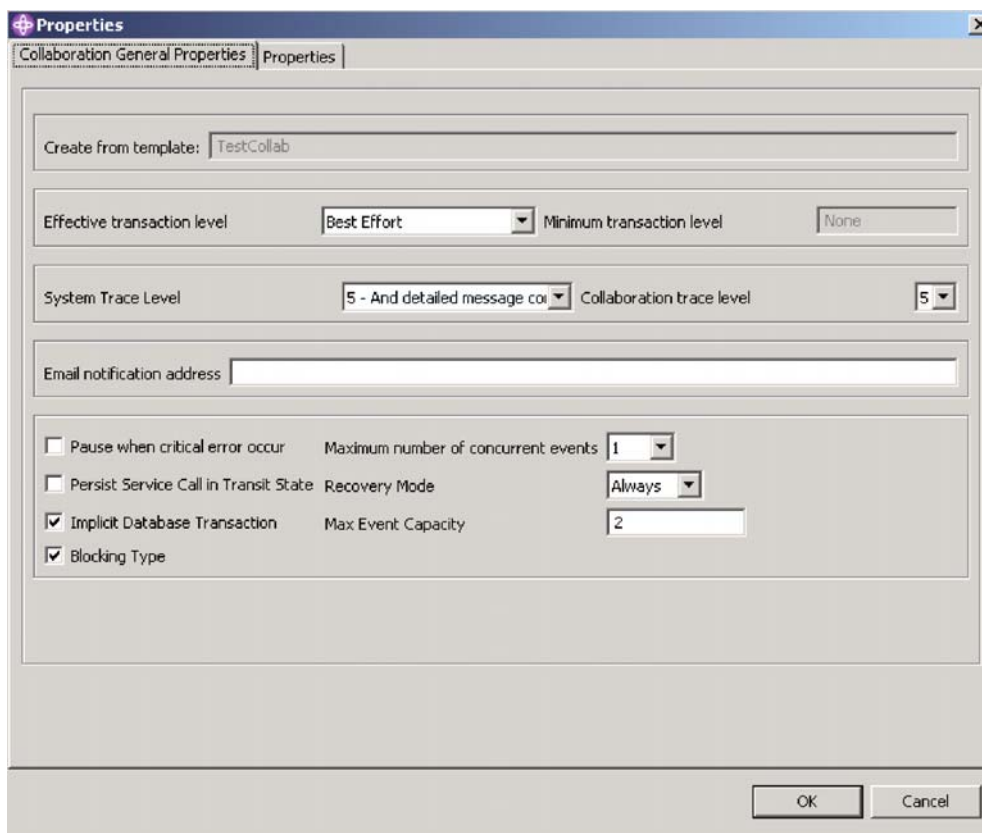
图 31. “属性”对话框, “协作一般属性”选项卡
