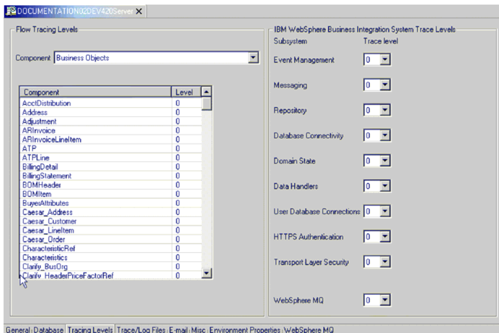
图 51. “编辑配置”工具，“跟踪级别”选项卡
