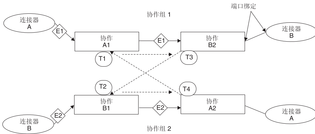
图 77. 协作组之间的死锁
