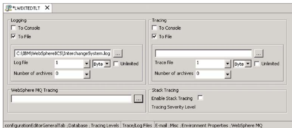
图 50. “编辑配置”工具，“跟踪 / 日志文件”选项卡
