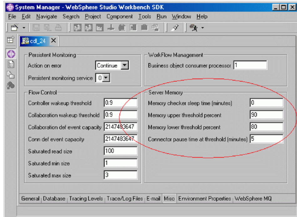
图 59. “编辑配置”工具，“其它”选项卡
