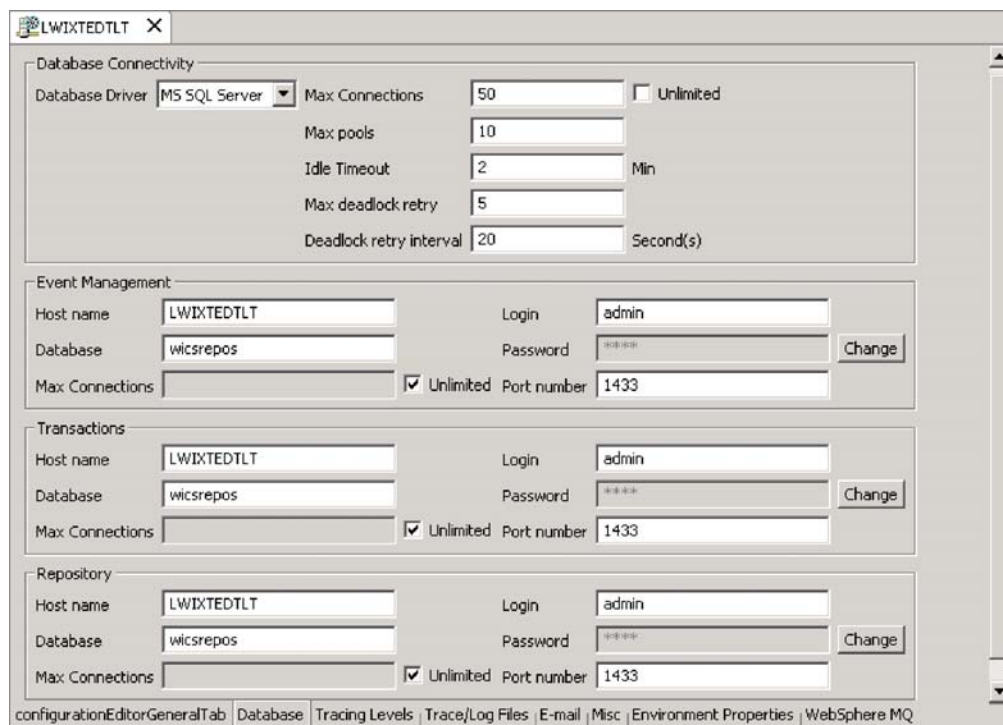
图 78. “编辑配置”屏幕, “数据库”选项卡
