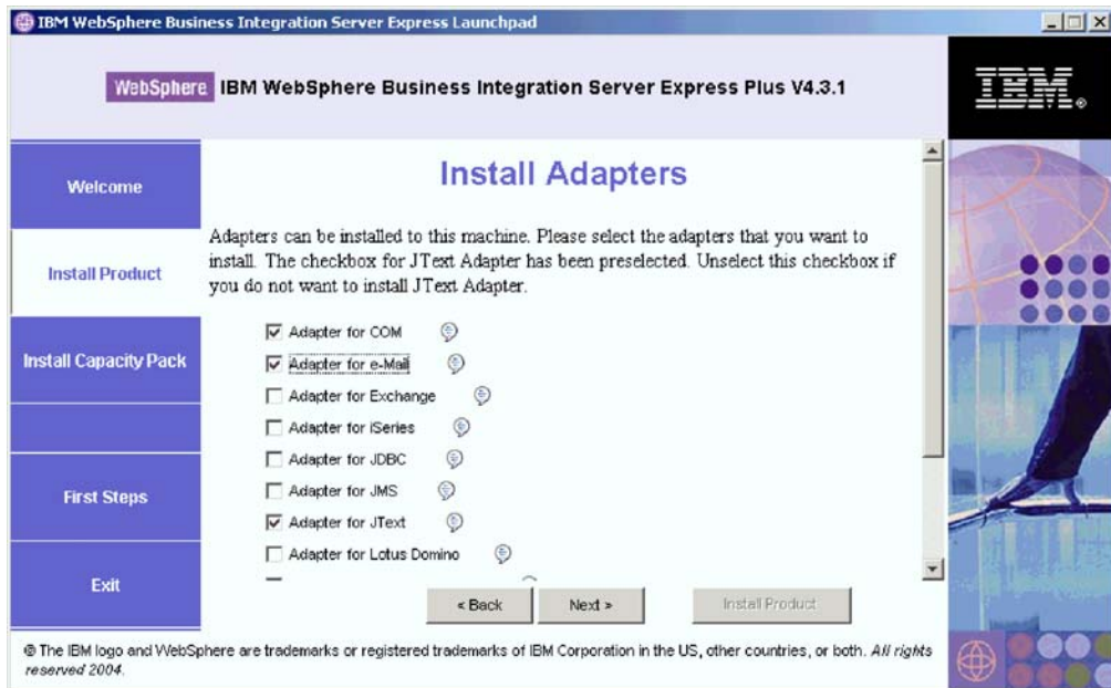
图 5. 安装适配器屏幕
