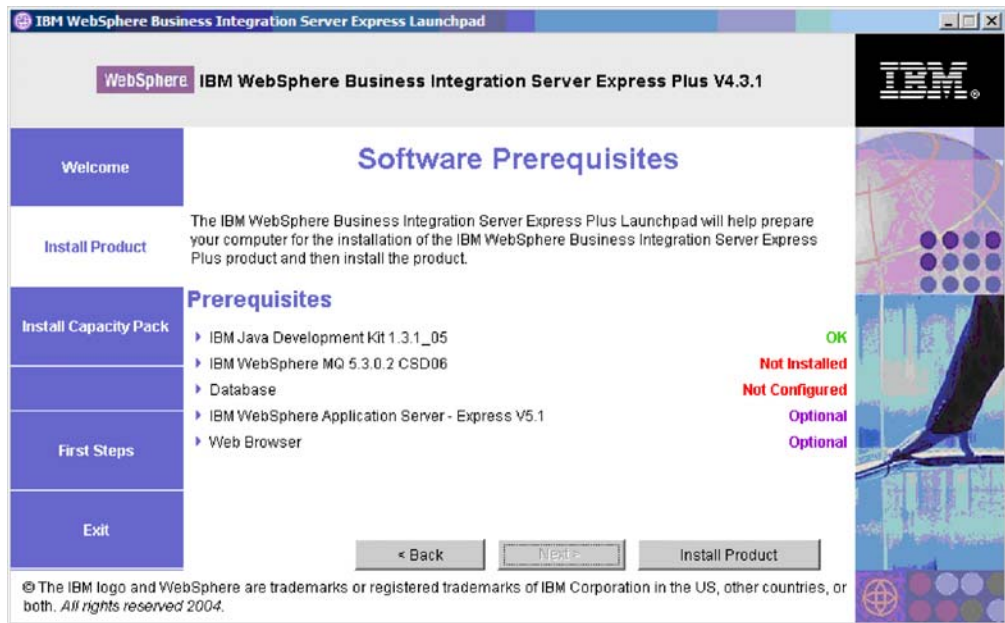
图 7. 安装选择的先决条件之前的“软件先决条件”屏幕
