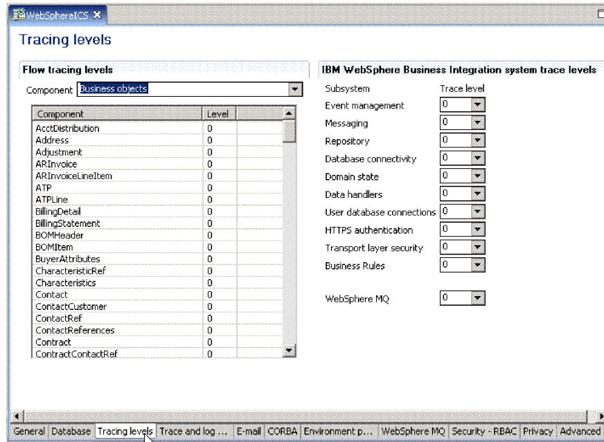
図 51. 「構成を編集」ツール、「トレース・レベル」タブ
