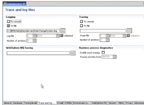
図 50. 「構成を編集」ツール、「トレース/ログ・ファイル」タブ
