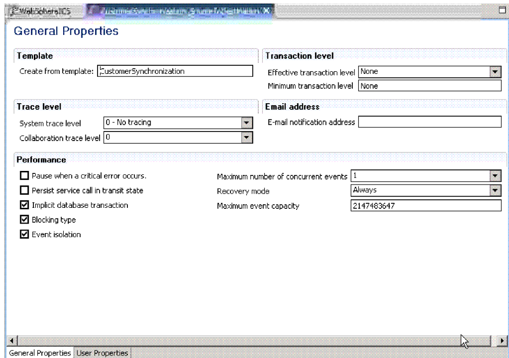
図 30. 「プロパティ」ダイアログ・ボックス、「コラボレーションの一般プロパティ」タブ
