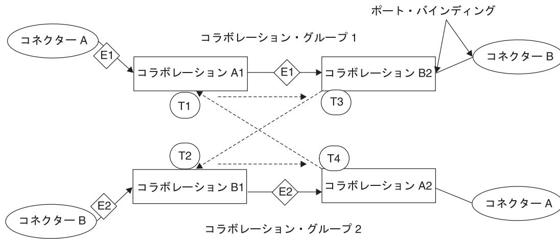
図 72. コラボレーション・グループ間のデッドロック
