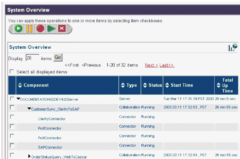
図 28. System Monitor、「システム概要」におけるコラボレーション・オブジェクト状況の表示
