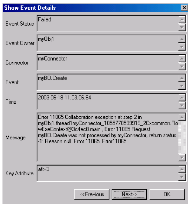
図 70. Flow Manager の「イベントの詳細を表示」ダイアログ・ボックス
