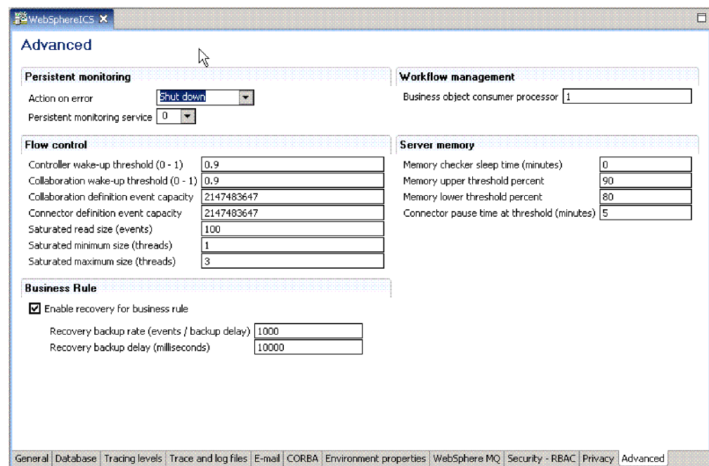
図 15. 「構成を編集」ツールの「拡張」タブ
