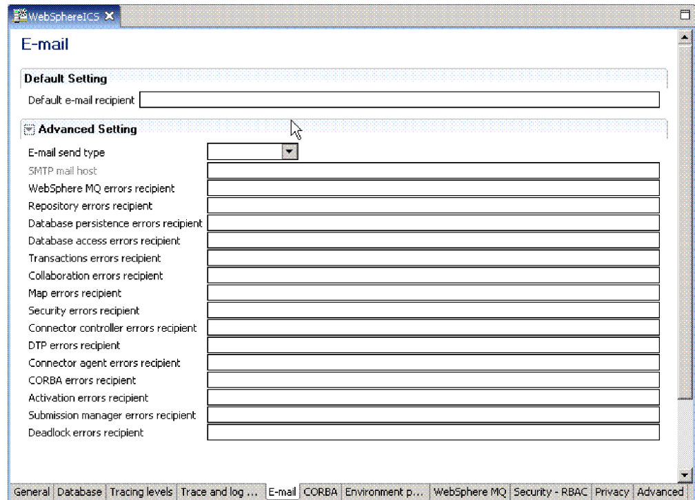
図 49. 「構成を編集」、 「E メール」タブ
