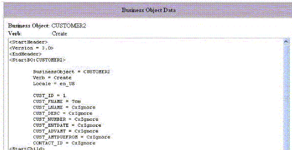
図 64. Failed Event Manager の「ビジネス・オブジェクト・データ」ダイアログ・ボックス
