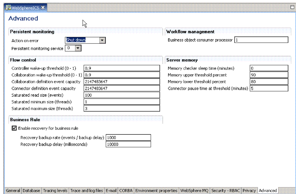
図 23. 「構成を編集」ツールの「拡張」タブ
