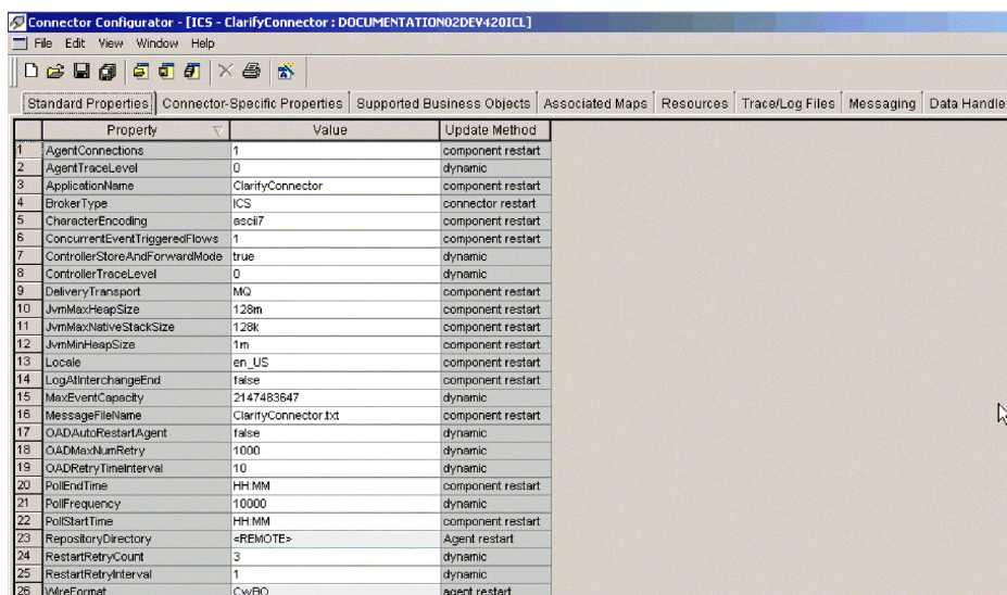
図 27. Connector Configurator Express、「標準のプロパティ」タブ
